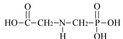
Figure 1: La structure chimique de la forme acide du glyphosate.
