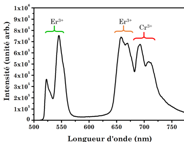
Figure 3.24 : Spectre d'émission des particules ZGO:Cr 0,5% Yb 5% Er 1% - cal ( \lambda_{\text{exc}} = 980 \text{ nm} ).
