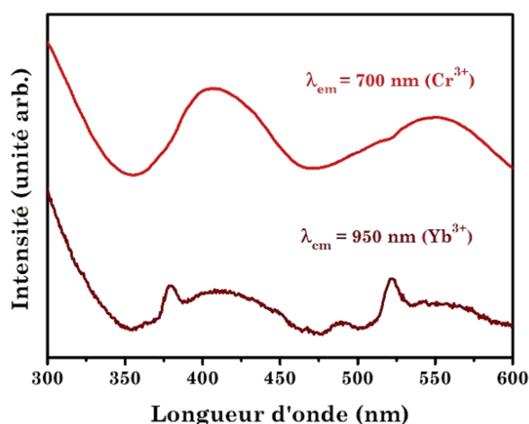
Figure 3.28 : Spectres d'excitation des nanoparticules de \text{ZGO}:\text{Cr}_{0,5\%}\text{Yb}_{5\%},\text{Er}_{1\%} - cal à 700 ( \text{Cr}^{3+} ) et 950 nm ( \text{Yb}^{3+} ).
