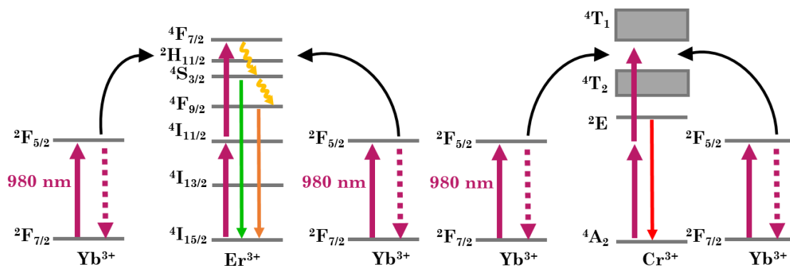
Figure 3.27 : Représentation schématique du mécanisme de transfert énergétique entre les ions \text{Yb}^{3+} et \text{Er}^{3+} et \text{Yb}^{3+} et \text{Cr}^{3+} .
