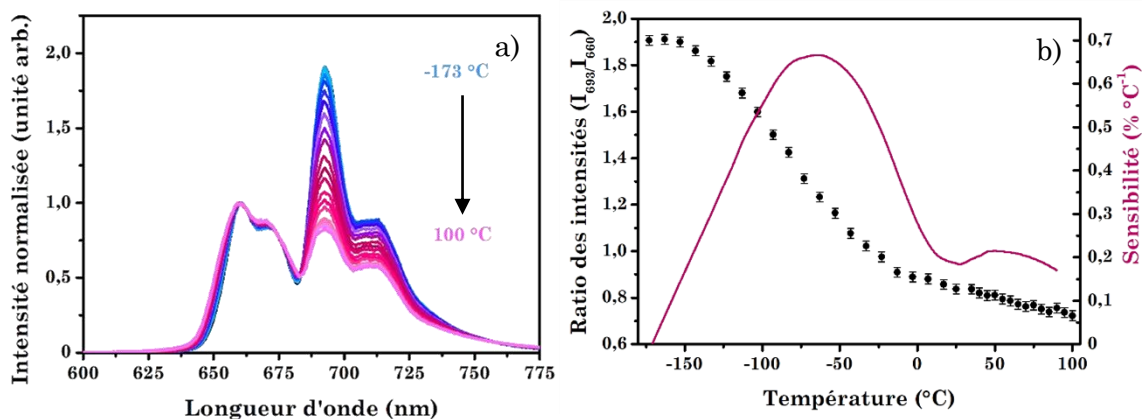
Figure 3.26 : a) Spectres d'émission normalisés à différentes températures des nanoparticules ZGO:Cr 0,5% Yb x% ,Er 1% - cal ( \lambda_{exc} = 980 nm) b) Ratio des intensités des pics d'émission centrés à 692 nm (Cr 3+ ) et 660 nm (Er 3+ ), la sensibilité associée est représentée en rose.
