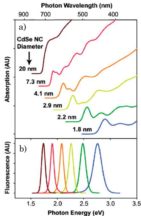
Figure 1.3 : Spectres d'absorption a) et d'émission b) de quantum dots CdSe/ZnS cœur/coquille dont le diamètre du cœur varie de 1,8 à 20 nm, issu de Chou et al. 11 .
