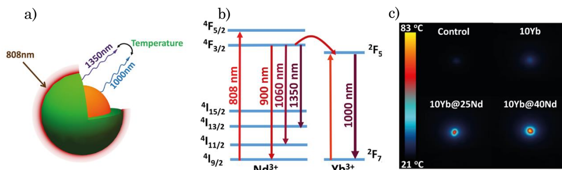
Figure A6.2: Représentation schématique a) de la particule cœur (diamètre 15 nm)/coquille (épaisseur 4,5 nm) \text{LaF}_3\text{:Nd}^{3+}, \text{Yb}^{3+}/\text{LaF}_3\text{:Nd}^{3+} , b) des niveaux énergétiques des centres émetteurs \text{Nd}^{3+} et \text{Yb}^{3+} ainsi que des transitions radiatives et le transfert énergétique ion-ion. c) Image par caméra thermique des particules cœur simple ou cœur/coquille avec une concentration en ions dopants de la coquille différente sous excitation à 808 nm de puissance de 3,4 W/cm 2 , issu de Ximendes et al. * 1 .
