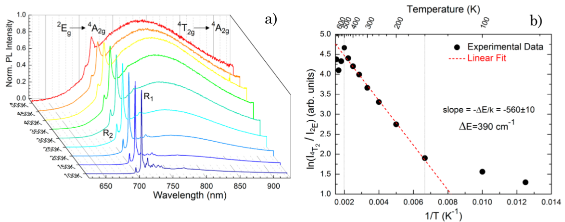
Figure 1.12 : a) Spectre de photoluminescence du composé Bi_2Ga_4O_9:Cr^{3+} à différentes températures (de -193 °C (bleu) à 327 °C (rouge)) b) Ratio des intensités en fonction de la température, adapté de Back et al. 58 .
