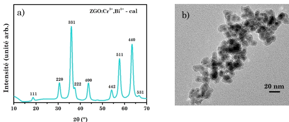
Figure 2.24 : a) Diffractogramme des RX et b) cliché MET de nanoparticules de \text{ZGO}:\text{Cr}^{3+},\text{Bi}^{3+} - cal.
