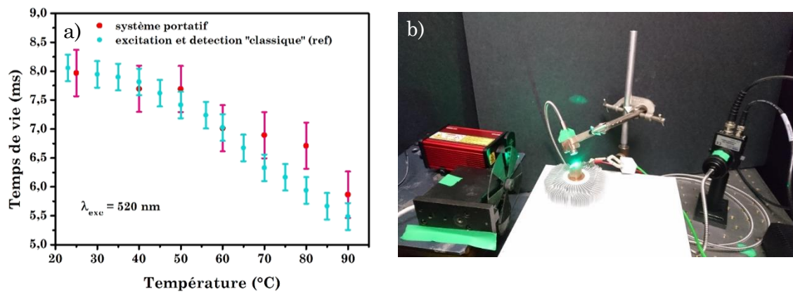
Figure 4.25 : a) Temps de vie de luminescence des nanoparticules ZGO:Cr 3+ ,Bi 3+ - cal sous excitation à 520 nm par le dispositif expérimental « classique » (en bleu) et par le dispositif portable (en rouge) b) Photo du dispositif portable mis en place au cours de cette thèse.
