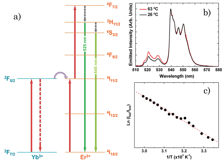
Figure 1.9 : a) Représentation schématique de l'excitation et la désexcitation au sein de nanoparticules à up-conversion b) Spectres d'émission en solution aqueuse à deux températures différentes après excitation à 920 nm c) Ratio des intensités des pics à 525 et 545 nm en fonction de 1/T , Vetrone et al. 39 .
