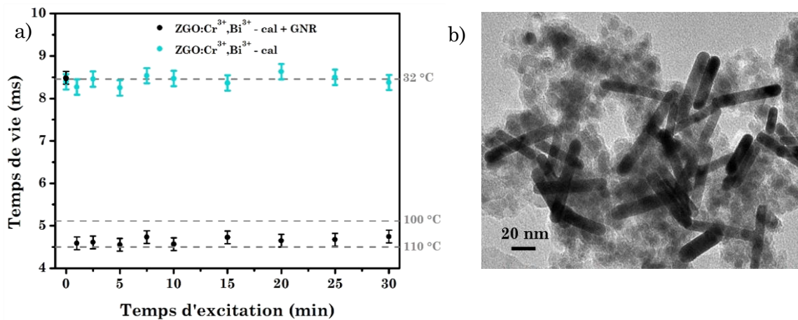
Figure 4.13 : a) Suivi de l'évolution de la température en fonction du temps d'excitation par une diode laser ( \lambda_{\text{exc}} = 976 nm), par le biais des temps de vie extraits des courbes de déclin de luminescence d'un mélange de \text{ZGO:Cr}^{3+},\text{Bi}^{3+} - cal, et de nanobâtonnets d'or sous forme de poudre. b) Cliché MET d'un mélange de \text{ZGO:Cr}^{3+},\text{Bi}^{3+} - cal et de nanobâtonnets d'or.
