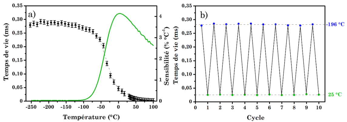
Figure 3.17 : a) Variation du temps de vie de luminescence des particules de \text{MgTiO}_3:\text{Mn}^{4+} en fonction de la température et sensibilité associée b) Temps de vie enregistrés alternativement entre deux températures respectivement -196\text{ }^{\circ}\text{C} et 25\text{ }^{\circ}\text{C} .
