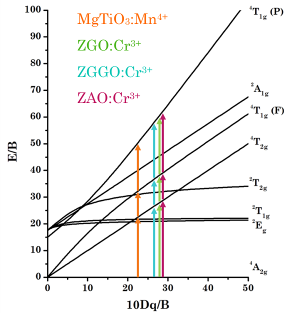
Figure A4.1 : Diagramme de Tanabe Sugano pour les ions en configuration d 3 (Cr 3+ et Mn 4+ ) en environnement octaédrique, les flèches indiquent les transitions se produisant dans les différentes matrices : MgTiO 3 (23,6 en orange) ZGGO (27,2 en bleu) ZGO (28,4 en vert) et ZAO (28,7 en rose).
