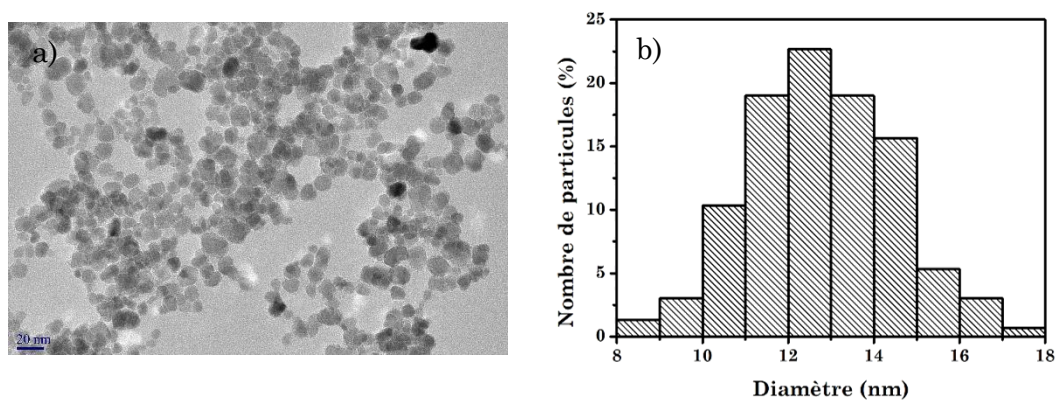
Figure 4.22 : a) Cliché MET des nanoparticules de \text{Fe}_2\text{O}_3 b) Diagramme de distribution associé.
