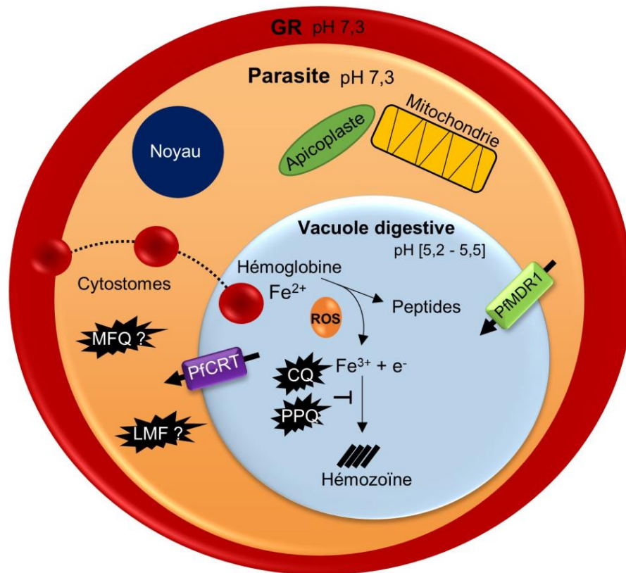
Figure 19 : Sites d'action de divers antipaludiques à base de quinoléine. CQ, chloroquine ; PPQ, pipéraquline ; LMF, luméfantrine ; MFQ, méfloquine ; PfcRT, P. falciparum chloroquine resistance transporter; PfMDR1, P. falciparum multidrug resistance 1. La CQ et la PPQ sont supposées traverser les membranes, probablement par diffusion passive, pour se concentrer au sein de la vacuole digestive du parasite et empêcher la conversion de l'hème toxique en hémotoïne non toxique pour le parasite. La méfloquine et la luméfantrine, elles, agiraient dans d'autres compartiments cellulaires ; pour ces deux dernières molécules, leur stockage dans la vacuole digestive pourrait être un mécanisme de résistance du parasite.
