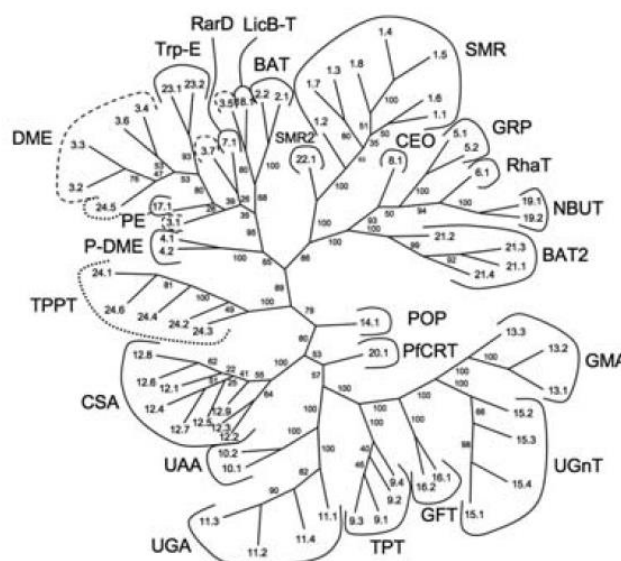
Figure 22 : Phylogénie des DMTs. PfCRT s'avère être proche de protéines Nucleotide-sugar transporter (NST), une sous-famille incluant les protéines CMP-sialate:CMF antiporter (CSA). La phylogénie est tirée du chapitre axée sur les transporteurs et leur lien avec la résistance aux médicaments, par Yen et ses collaborateurs (2010) 159 .
