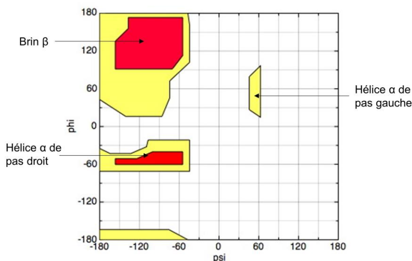
Figure 29 : Diagramme de Ramachandran. Chaque acide aminé dans la structure tertiaire est associé à des angles \phi ( \phi ) et \psi ( \psi ) formés par les liaisons peptidiques. Toutes les paires d'angles \phi et \psi ne sont pas possibles car certaines conduisent à des distances inter-atomiques qui sont énergétiquement très défavorables. Trois régions sont qualifiées comme favorables. Les deux principales (en rouge) correspondent aux structures secondaires régulières majoritairement observées dans les protéines : les hélices \alpha de pas droit et les brins \beta . La troisième région, plus petite, correspond à une conformation en hélice \alpha de pas gauche ( \phi > 0 ).
