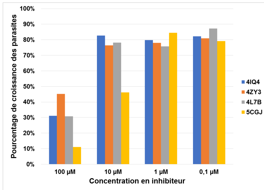
Figure 48 : Pourcentage de croissance des parasites P. falciparum après exposition à différentes concentrations en inhibiteurs KEAP1. Les noms des différentes molécules testées correspondent aux identifiants PDBs. La croissance des parasites est approximée par la mesure de la quantité d'ADN parasitaire détectée après 72 heures d'incubation en présence ou absence d'inhibiteur. La croissance des parasites en présence d'inhibiteur est exprimée en pourcentage de celle sans inhibiteur. Les expériences et analyses ont été réalisées par Laurine Rondepierre (doctorante, UMR 261).
