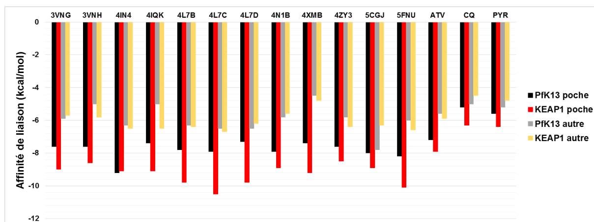
Figure 47 : Résultats des différents docking pour 15 molécules avec les poches KREP KEAP1 et KREP PfK13 . Seule la meilleure pose par molécule, correspondant à la plus haute affinité de liaison, est indiquée. L'affinité de liaison correspond à un échange énergétique, exprimée en kcal/mol. Généralement, on suppose qu'une énergie inférieure à -7 kcal/mol représente une forte affinité de liaison 270 . Les différentes molécules testées sont indiquées par leur identifiant PDB. Les trois derniers groupes d'histogrammes à droite exposent les résultats de docking pour trois antipaludiques servant de contrôles négatifs : ATV, atovaquone ; CQ, chloroquine ; PYR, pyriméthamine.
