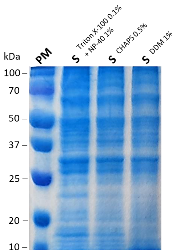
Figure 42 : Solubilisation des protéines de P. falciparum . Trois tampons de solubilisation à base de différents détergents ont été testés : Triton X-100 0,1% + NP-40 1% (TLp1) ; CHAPS 0,5% (TLp2) ; DDM 1% (TLp3). De multiples bandes couvrant l'échelle des poids moléculaires (PM) ont été observées, suggérant que de nombreuses protéines du parasite sont solubles. Une quantité similaire de protéines a été incubée avec les différents tampons : après centrifugation, un aliquot du surnageant a été analysé par SDS-PAGE. S : fraction soluble. La coloration des gels a été faite au Coomassie (0,25% bleu de Coomassie, complété par de l'éthanol à 96%).
