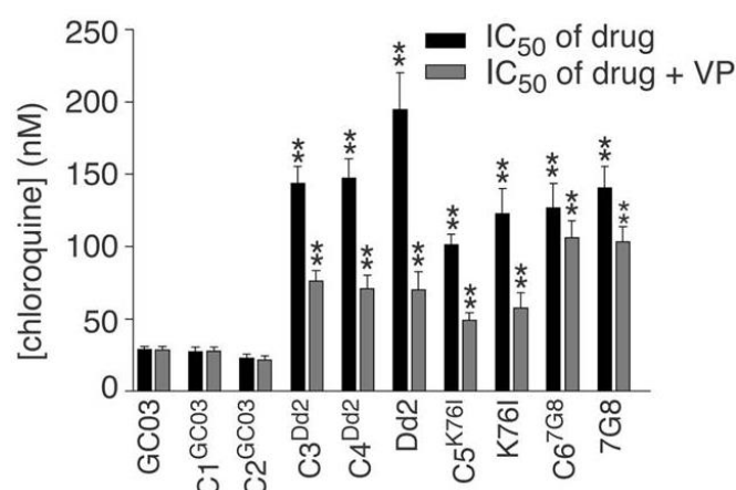
Figure 23 : Évaluation du rôle des mutations pfcr t dans la résistance à la CQ par mesure de la IC_{50} chez des parasites P. falciparum cultivés in vitro . Les souches GC03, C1 et C2 portent un haplotype pfcr t sauvage. C3, C4 portent l'haplotype pfcr t de la souche asiatique Dd2. C5 modifie l'haplotype Dd2 sur deux positions : K76I (au lieu de K76T) et absence de la mutation I356T. C6 porte l'haplotype pfcr t de la souche brésilienne 7G8. Le vérapamil (VP) est un inhibiteur de canaux calciques et réverse partiellement la IC_{50} des parasites pfcr t mutants. Les tests statistiques ont été réalisés entre la souche de référence C2 GC03 et les autres (** : P < 0.01 ). D'après Sidhu et al. (2002) 52 .
