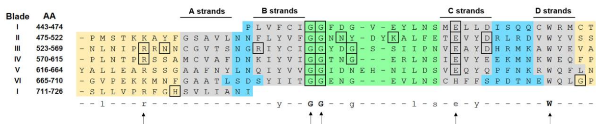
Figure 49 : Mise en évidence des sites les plus conservés du domaine KREP de Pfk13 avec l'outil codeml de PAML. Les motifs kelch (blades) ont été structuralement alignés pour produire l'alignement multiple des séquences. Une séquence consensus de l'alignement est indiquée en dessous de celui-ci. Les sites les plus conservés (au seuil 10%) d'après l'outil codeml sont entourés en noir. Les flèches indiquent les acides aminés importants pour le bon repliement d'un domaine KREP 107,108 .
