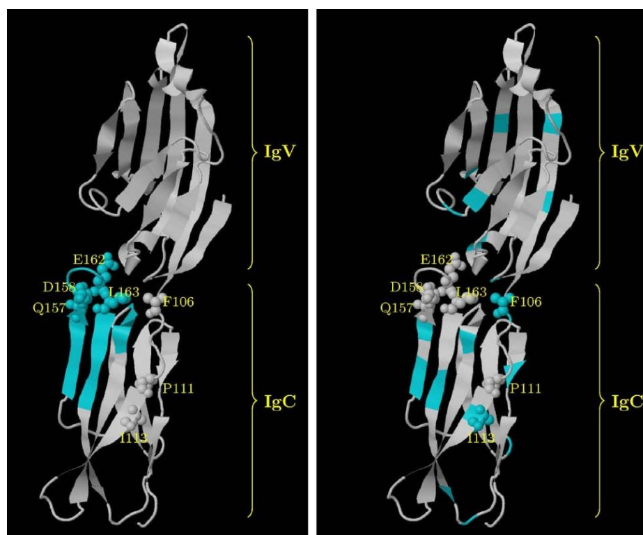
Figure 26 : Localisation dans la structure tertiaire des sites les plus conservés (au seuil de 10%) dans la protéine humaine B7-1 en considérant (panel gauche) ou non (panel droite) l'environnement spatial des sites pour l'estimation de leur taux de substitution. GP4Rate a été utilisé pour estimer les taux de substitution en prenant en compte la structure tertiaire 192 ; Rate4Site a été utilisé pour estimer les taux de substitution sans considérer les informations de la structure tertiaire. Les sites les plus conservés sont représentés en bleu cyan ; les sites clés dans la fonction de B7-1 sont indiqués en lettres jaunes. La figure est tirée du travail de Huang et Golding (2014) 192 .
