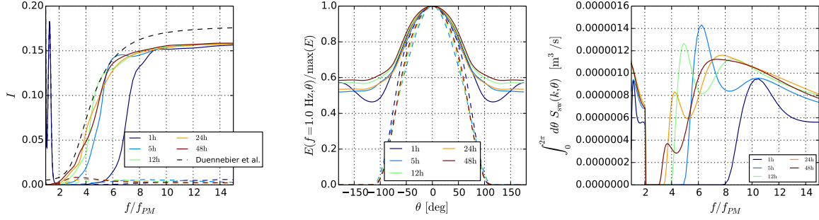
FIGURE 4.13 – Évolution temporelle de l'intégrale de recouvrement, de la distribution directionnelle à f = 1 \text{ Hz} et du terme source de création de vagues courtes (4.1) en fonction de f/f_{PM} lorsque les interactions non-linéaires sont calculées de manière approchée, à un vent U_{10} = 12 \text{ m} \cdot \text{s}^{-1} . Sont représentés en traits pleins, les résultats de la configuration donnant la meilleure intégrale de recouvrement ( c_0 = 0.01 ), et en pointillés ceux de la simulation de référence sans terme source de vagues courtes ( c_0 = 0 ).
