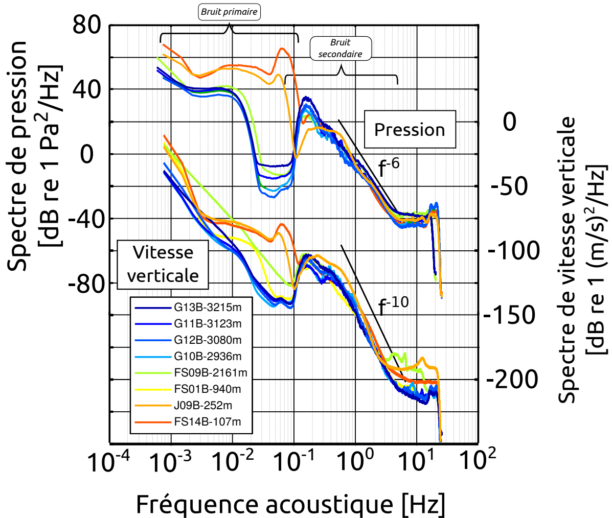
FIGURE 2.9 – Spectres médians de pression et de vitesse verticale de la croute aux stations étudiées.
