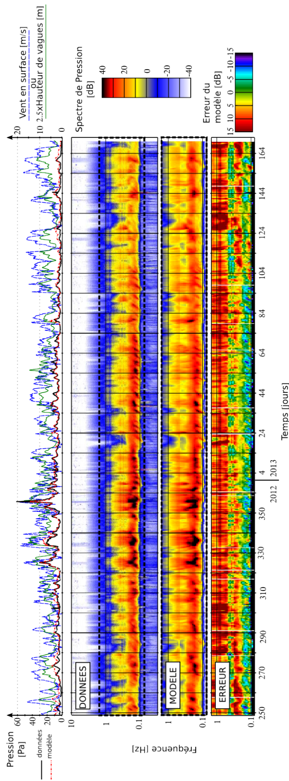
FIGURE 2.12 – Spectrogrammes de bruit acoustique à la station G10B. (a) Moyenne quadratique de l'amplitude de la pression, p_{\text{RMS}} = \sqrt{\int_{0.04 \text{ Hz}}^{10 \text{ Hz}} F_p(f_s) df_s} et conditions météo. (b-d) Spectrogrammes de bruit acoustique observé, modélisé et erreur associée \Delta_{\text{dB}} = 10 \log_{10} (F_p^{\text{modèle}}) - 10 \log_{10} (F_p^{\text{données}}) . Adapté de Peureux et Arduin [129].
