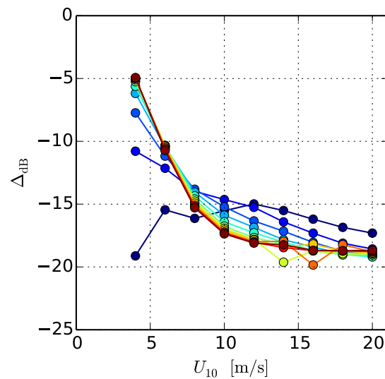
FIGURE 4.8 – Différence en décibels entre les prédictions du modèle de vagues avec formulation R&A et la paramétrisation de Duennebier et al. pour des vagues de 1 Hz. les calculs sont réalisés dans la configuration la plus proche de la modélisation du chapitre 2 (à savoir une formulation R&A des termes sources et un calcul approché des interaction non-linéaires). L'erreur est tracée de t = 4 h (bleu) jusqu'à t = 48 h (rouge) toutes les 4 h.
