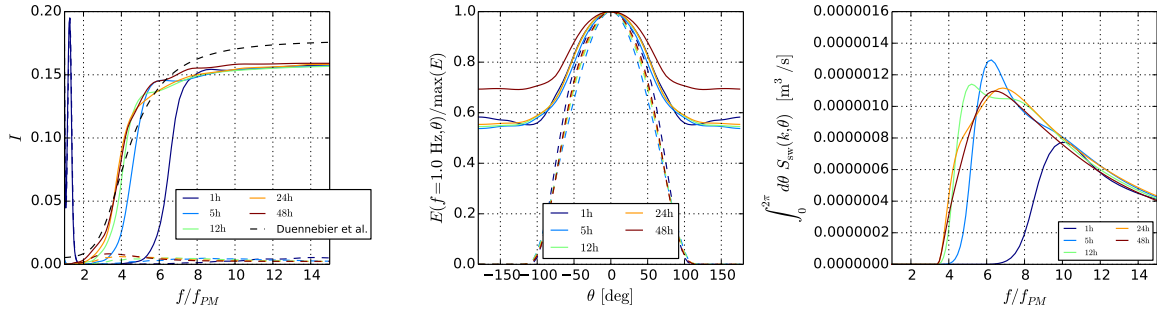
FIGURE 4.15 – Évolution temporelle de l'intégrale de recouvrement, de la distribution directionnelle à f = 1 \text{ Hz} et du terme source de création de vagues courtes en fonction de f/f_{PM} pour le terme source (4.3) lorsque les interactions non-linéaires sont calculées de manière approchée à un vent U_{10} = 12 \text{ m} \cdot \text{s}^{-1} . Sont représentés en traits pleins, les résultats de la configuration donnant la meilleure intégrale de recouvrement ( c_1 = 0.1 ), et en pointillés ceux de la simulation de référence sans terme source de vagues courtes ( c_1 = 0 ).
