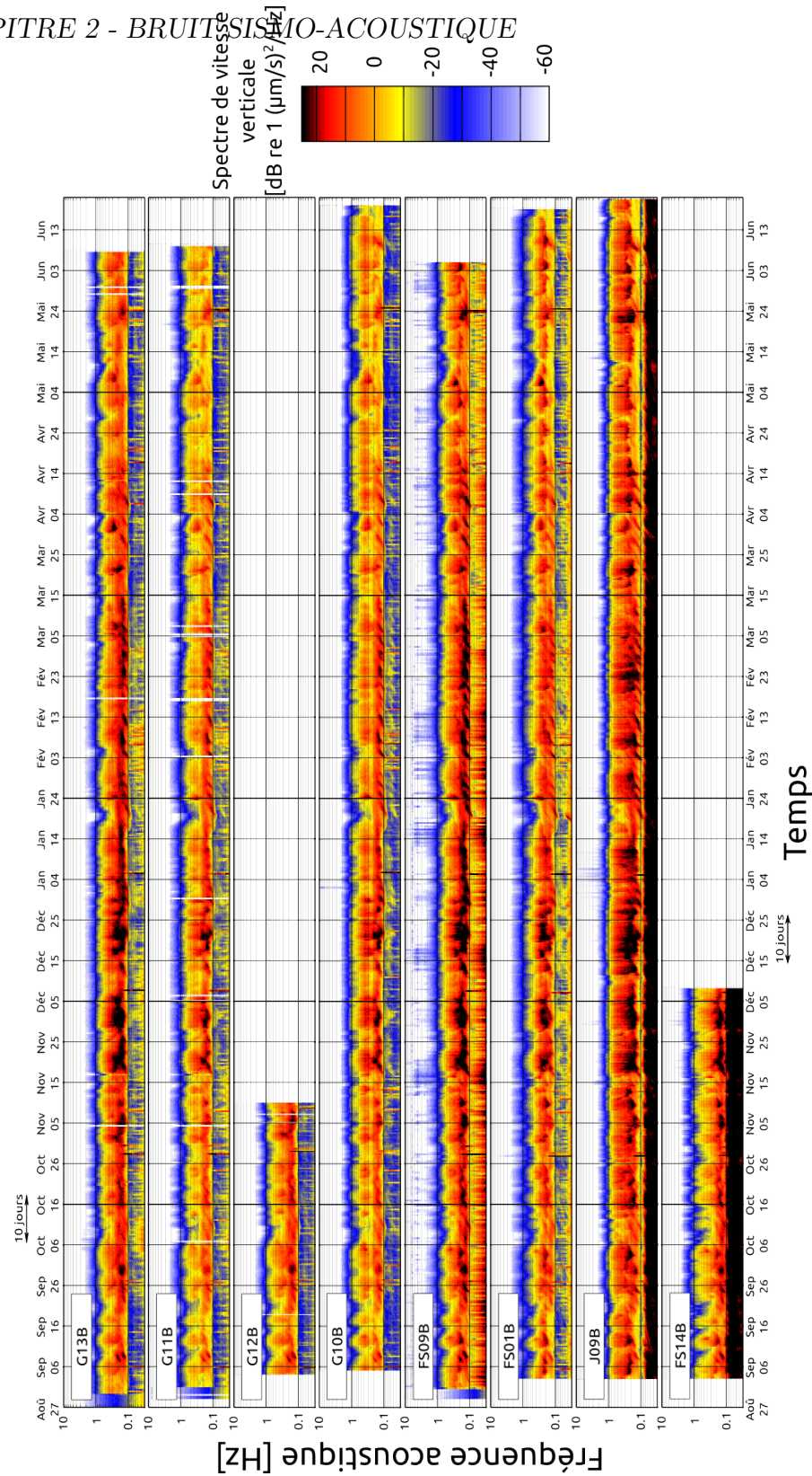
FIGURE 2.8 – Identique à la figure 2.7, cette fois pour le spectre de vitesse verticale de la croute terrestre.
