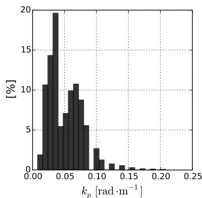
FIGURE 2.5 – Histogramme du nombre d'onde pic k_p à la bouée NDBC 46022 de décembre 2013 à décembre 2013.
