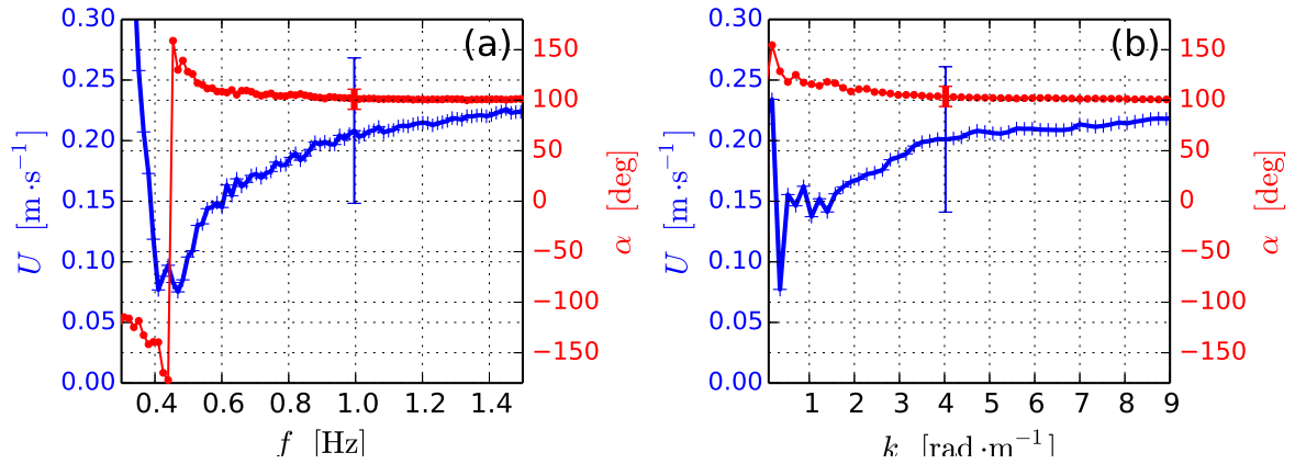
FIGURE 3.3 – Exemple de profil de courant effectif (3.3) (norme et direction) pour le cas de référence à Acqua Alta (27/03/2014), à partir de coupes à fréquence constante (a) ou nombre d'onde constant (b). Adapté de Peureux et al. [131].
