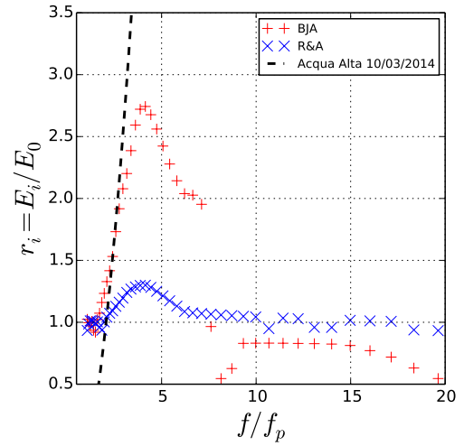
FIGURE 4.5 – Ratios des lobes pour les différentes configurations employant le calcul complet des interactions non-linéaires.
