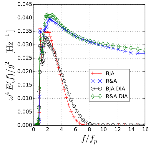
FIGURE 4.7 – Spectres de variance des pentes obtenus à l'issue des cas tests pour les différentes combinaisons de termes sources (voir équation (??)).
