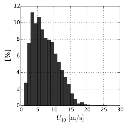
FIGURE 2.6 – Histogramme de vitesse du vent à la bouée (1 h) à la bouée NDBC 46022 de décembre 2012 à décembre 2013.
