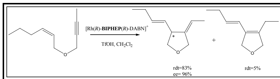
Schéma I.27 : réaction de cyclisation-ène catalysée par un complexe Rh/BIPHEP.
