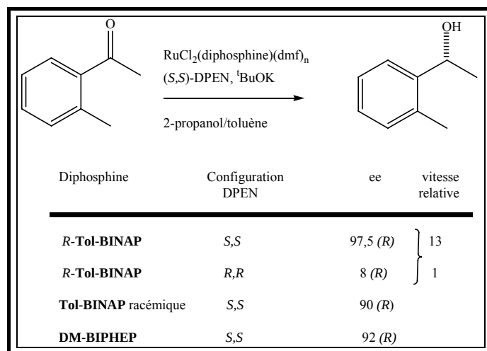
Schéma I.21 : utilisation de la Tol-BINAP et du BIPHEP en réduction des cétones.
