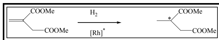
Schéma IV.22 : Hydrogénation du diméthyle itaconate.
