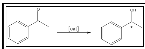
Schéma I.41 : réaction d'hydrogénation ou réaction par transfert d'hydrogène sur l'acétophénone.
