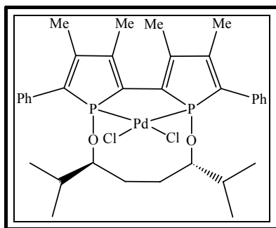
Dichloro-1,1'-(2,7-diméthyl-octane-3,6-dioxy)- 3,3',4,4'-tétraméthyl-5,5'-diphényl-2,2'-biphosphole
