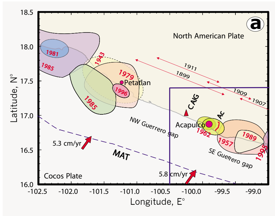
FIGURE 1.15: Localisation des séismes majeurs au niveau de la lacune de Guerrero ( Guerrero gap ). Les deux parties de la lacune (nord-ouest et sud-est) sont présentées. La localisation des séismes anciens est indiquée par des flèches, celle des séismes récents par les contours des glissements. D'après Ortiz et al. [2000].
