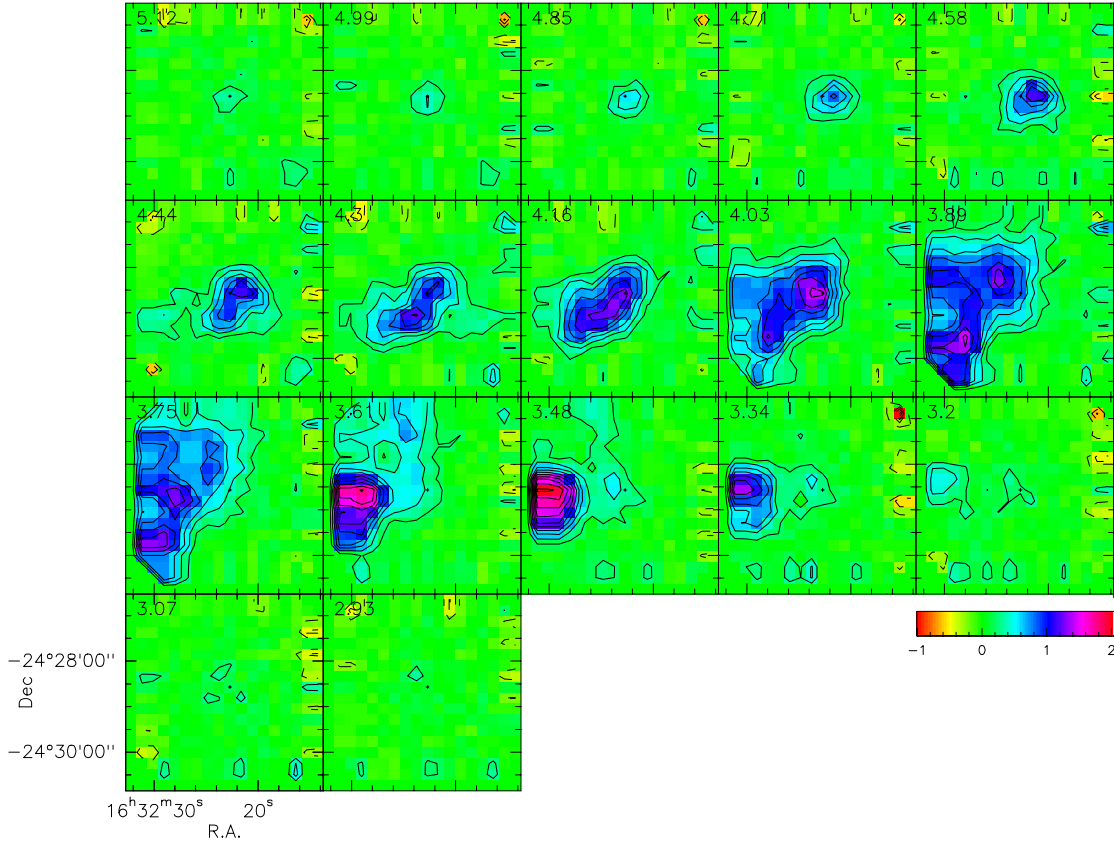
FIGURE A.5 – Carte de la transition de ortho- c\text{-C}_3\text{H}_2 à 85.339 GHz en fonction des canaux de vitesse obtenue avec le télescope de l'IRAM.
