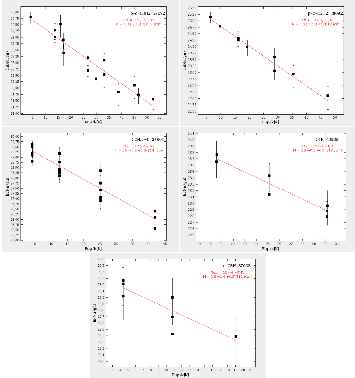
FIGURE A.1 – Diagrammes rotationnels des espèces ortho- \text{c-C}_3\text{H}_2 , para- \text{c-C}_3\text{H}_2 , CCH, \text{C}_4\text{H} et \text{c-C}_3\text{H} détectées dans le relevé spectral TIMASSS sans correction de dilution.
