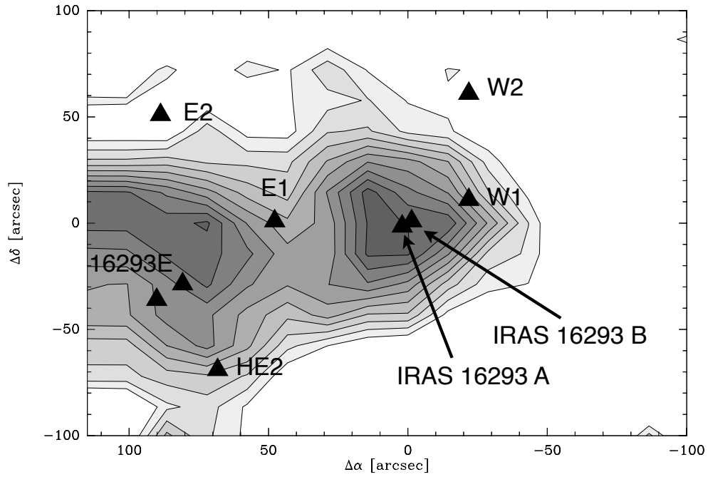
FIGURE A.9 – Carte intégrée en vitesse de la transition de ortho-c-C 3 H 2 à 85.339 GHz obtenue avec le télescope de l'IRAM. Les contours représentent 0.3, 0.4, ... 1.2 K.km s -1 . Le rms est de 0.15 K.
