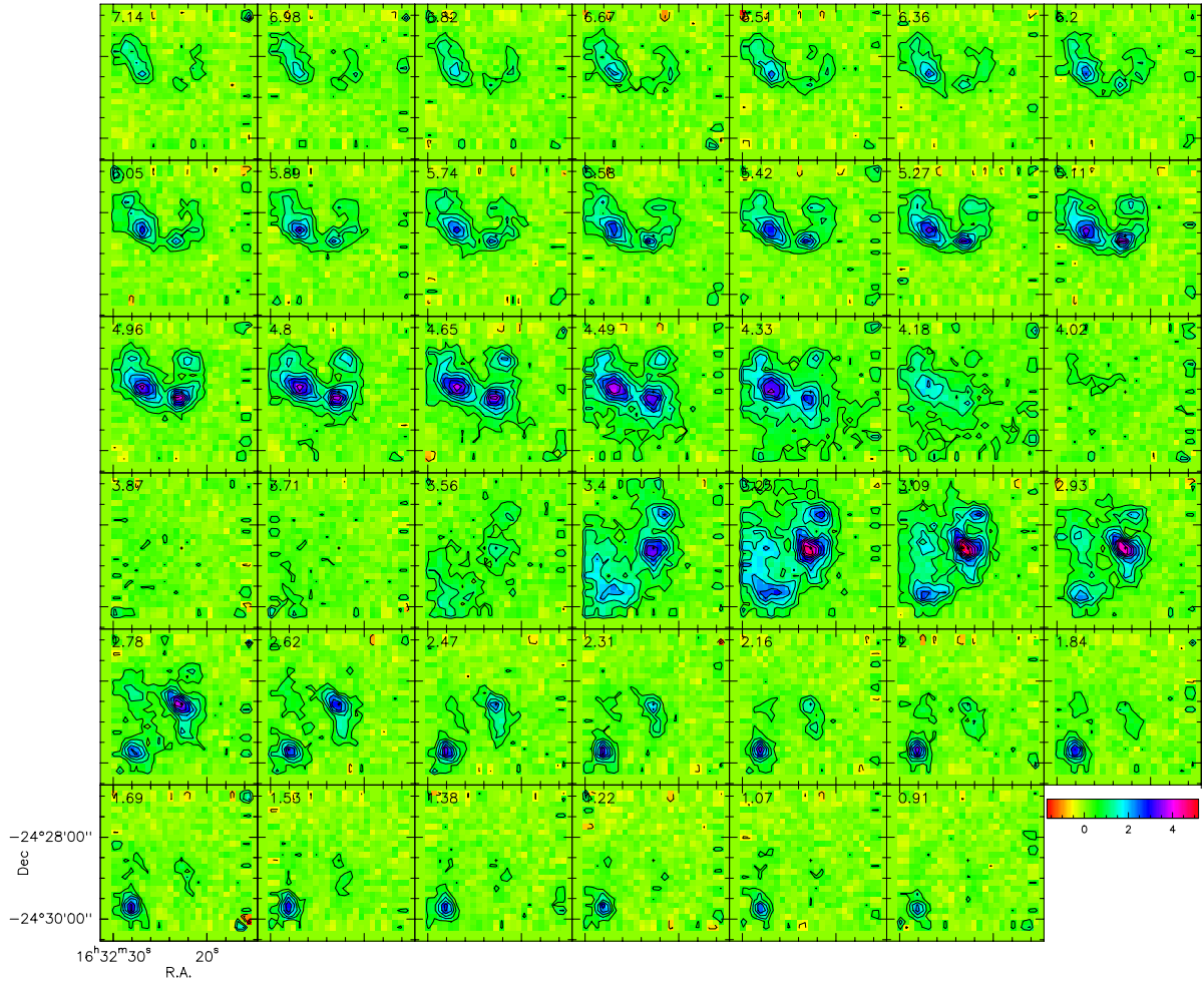
FIGURE A.21 – Carte de la transition de \text{H}_2\text{CO} à 150.498 GHz en fonction des canaux de vitesse obtenue avec le télescope de l'IRAM.
