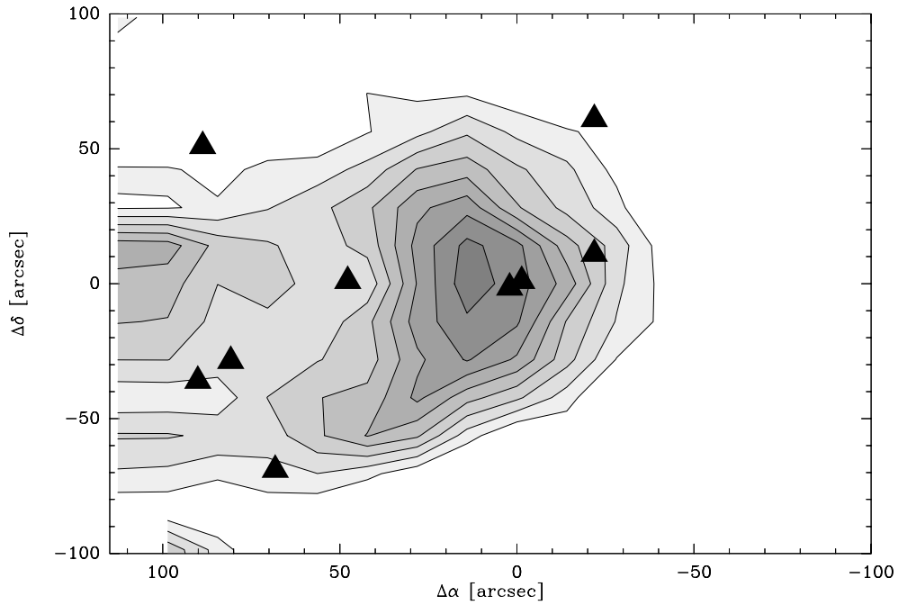
FIGURE A.12 – Carte intégrée en vitesse de la transition de CCH à 87.329 GHz obtenue avec le télescope de l'IRAM. Les contours représentent 0.3, 0.4, ... 1.0 K.km s -1 . Le rms est de 0.2 K.
