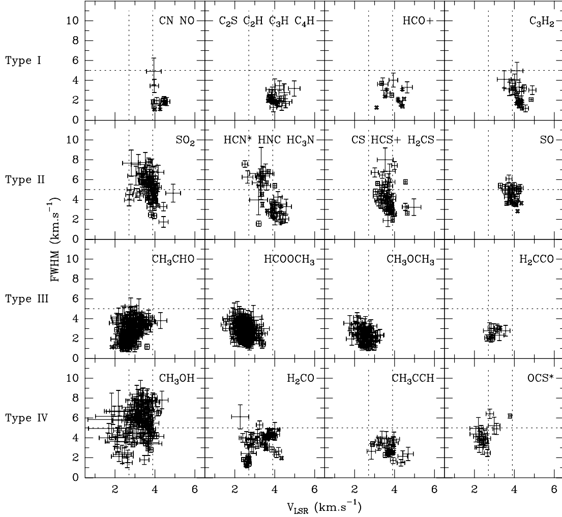
FIGURE 2.9 – Graphes des largeurs à mi-hauteur FWHM en fonction des vitesses au repos v_{LSR} déduits des ajustements gaussiens des raies. Les notations HCN* et OCS* indiquent que les isotopes principaux de ces espèces n'ont pas été inclus à cause de leur profil non-gaussien. Les barres d'incertitude à 1\sigma incluent à la fois les incertitudes d'ajustement et de résolution spectrale. Les traits verticaux à v_{LSR} = 2.7 et 3.9 \text{ km s}^{-1} correspondent aux vitesses des cœurs B et A respectivement. Le trait horizontal à 5 \text{ km s}^{-1} correspond approximativement à la moyenne des FWHM . Figure extraite de Caux et al. (2011).
