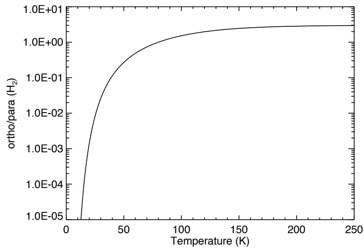
FIGURE 3.7 – Rapport ortho/para de H_2 à l'équilibre thermodynamique local.
