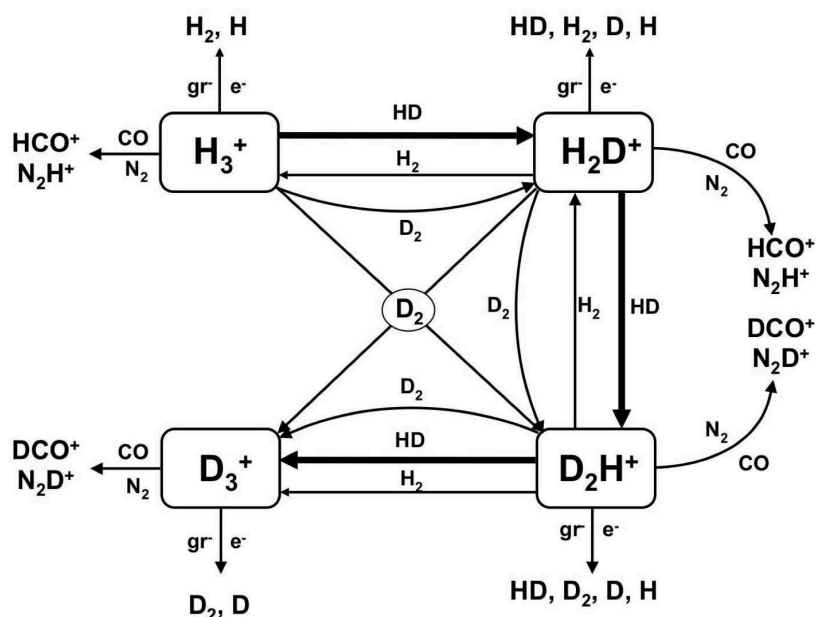
FIGURE 1.5 – Principales réactions impliquant l'ion \text{H}_3^+ et ses formes deutérées. Lorsque \text{CO} et \text{N}_2 déplètent, les réactions dominantes sont indiquées par des flèches en gras. e^- et \text{gr}^- représentent les électrons et grains négativement chargés respectivement. Figure extraite de Pagani et al. (2009).
