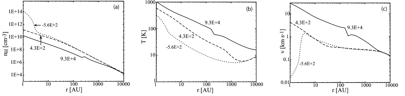
FIGURE 3.26 – Distributions radiales de la densité, la température et la vitesse d'effondrement prédites par le modèle radiatif hydrodynamique à t = -5.6 \times 10^2 ans, t = 4.3 \times 10^2 ans et t = 9.3 \times 10^4 ans. Figure extraite de Aikawa et al. (2012).
