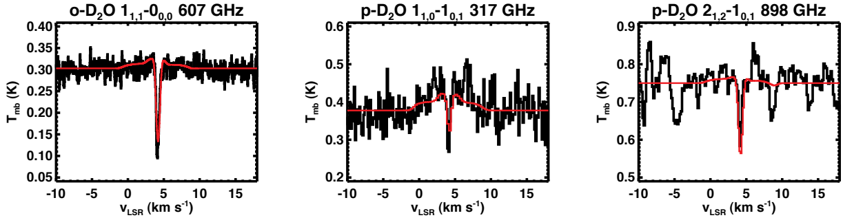
FIGURE 3.23 – En noir : les raies de D 2 O observées avec HIFI et JCMT. La transition de CH 3 OD qui chevauche la raie de para-D 2 O à 317 GHz a été soustraite pour la modélisation. En rouge : le meilleur ajustement obtenu en ajoutant une couche d'absorption avec N(para-D 2 O) = 1.1 \times 10^{12} \text{ cm}^{-2} et N(ortho-D 2 O) = 1.4 \times 10^{12} \text{ cm}^{-2} . L'abondance interne est de 7 \times 10^{-10} et l'abondance externe est de 5 \times 10^{-12} .
