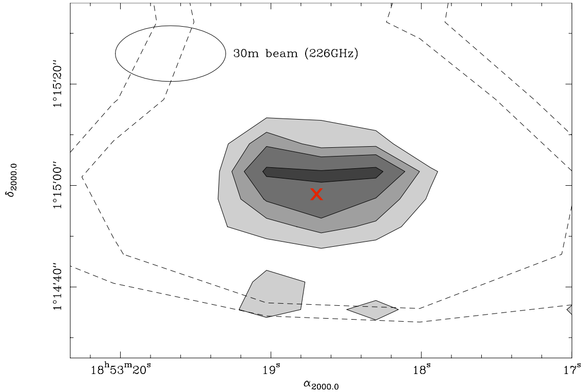
FIGURE 5.3 – Carte des transitions 3_{1,2}\text{--}2_{2,1} (trait continu) et 1_{1,0}\text{--}1_{1,1} (pointillés) de HDO observées avec le télescope de 30 m de l'IRAM en direction de la région HII G34 à 226 GHz et 81 GHz respectivement. Les niveaux de contour des observations (en T_A^* ) correspondent à 226 GHz à 2, 4, 6 et 9 \text{K.km s}^{-1} et à 81 GHz à 2 et 3 \text{K.km s}^{-1} . La croix rouge indique la position pointée par Herschel/HIFI.
