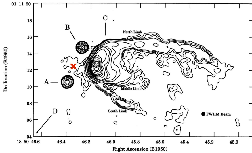
FIGURE 5.1 – Carte du continuum à 2 cm de la région G34. Les niveaux de contour sont -0.3, 0.3, 0.5, 0.75, 1.0, 2.5, 5, 10, 15, 25, 35, ..., 95% de la densité de flux au pic 0.303 \text{ Jy beam}^{-1} . Les sources A, B et C sont indiquées sur la carte. La source circulaire D qui s'étend sur 1' est hors de la carte. La direction de sa position est indiquée par une flèche. La croix rouge signale la position pointée par Herschel/HIFI. Figure extraite de Gaume et al. (1994).
