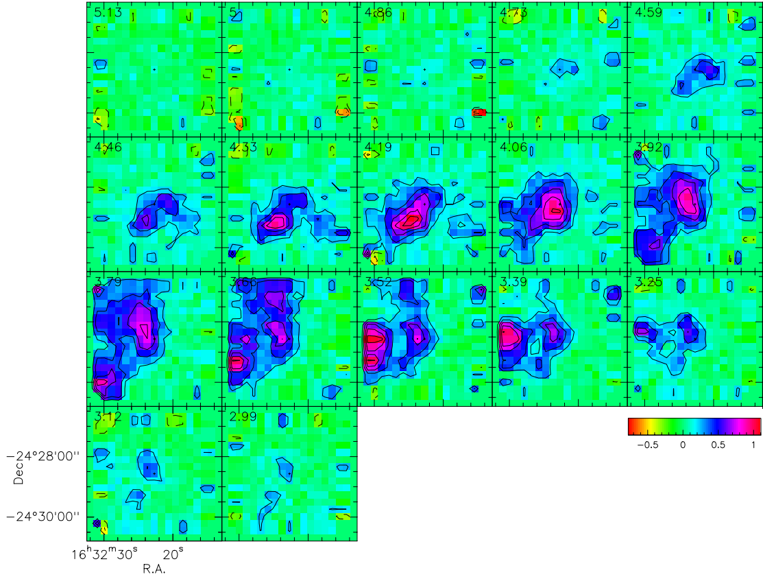
FIGURE A.6 – Carte de la transition de CCH à 87.402 GHz en fonction des canaux de vitesse obtenue avec le télescope de l'IRAM.
