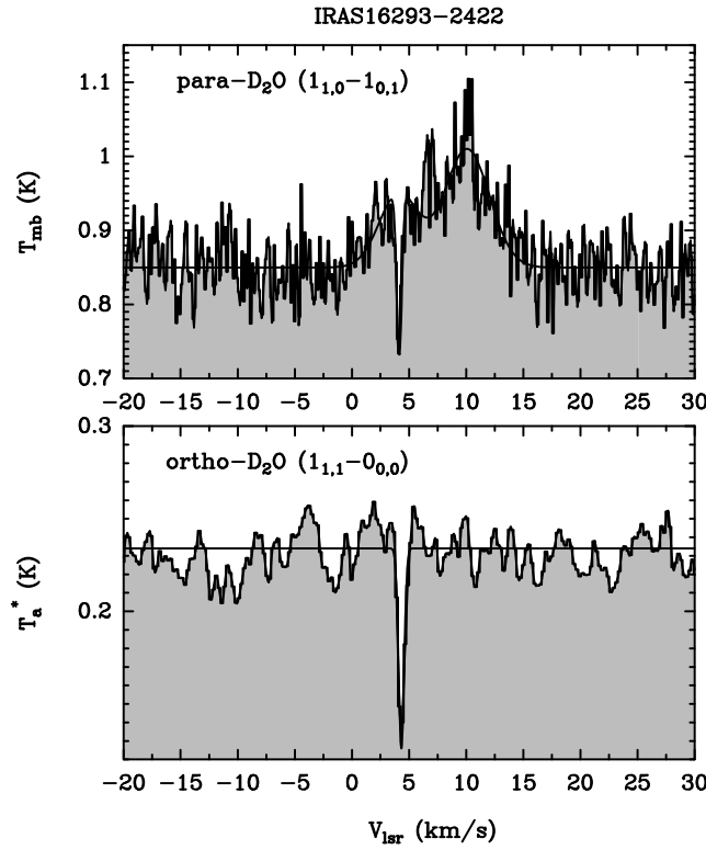
FIGURE 3.20 – Observations de la transition fondamentale 1_{1,0}-1_{0,1} de para- \text{D}_2\text{O} obtenue avec le télescope JCMT (panneau supérieur) et ajustée par une somme de 3 Gaussiennes et de la transition fondamentale 1_{1,1}-0_{0,0} de ortho- \text{D}_2\text{O} obtenue avec HIFI (panneau inférieur). La raie située à environ 10 \text{ km s}^{-1} de la raie de para- \text{D}_2\text{O} est attribuée à la transition ( 7_0-6_0+ ) de \text{CH}_3\text{OD} . Figure extraite de Vastel et al. (2010).
