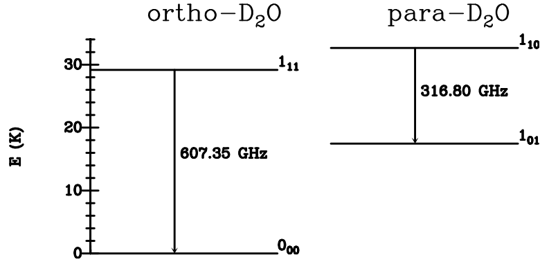
FIGURE 3.19 – Niveaux en énergie des transitions fondamentales de \text{D}_2\text{O} . Figure extraite de Vastel et al. (2010).
