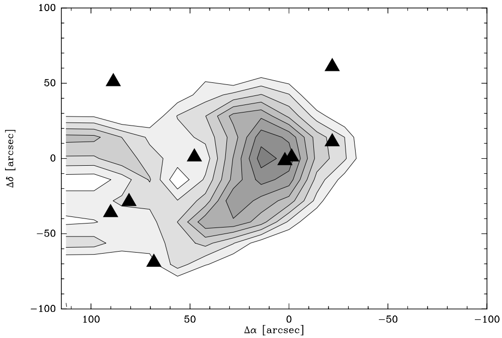
FIGURE A.13 – Carte intégrée en vitesse de la transition de CCH à 87.402 GHz obtenue avec le télescope de l'IRAM. Les contours représentent 0.4, 0.5, ... 1.1 K.km s -1 . Le rms est de 0.2 K.
