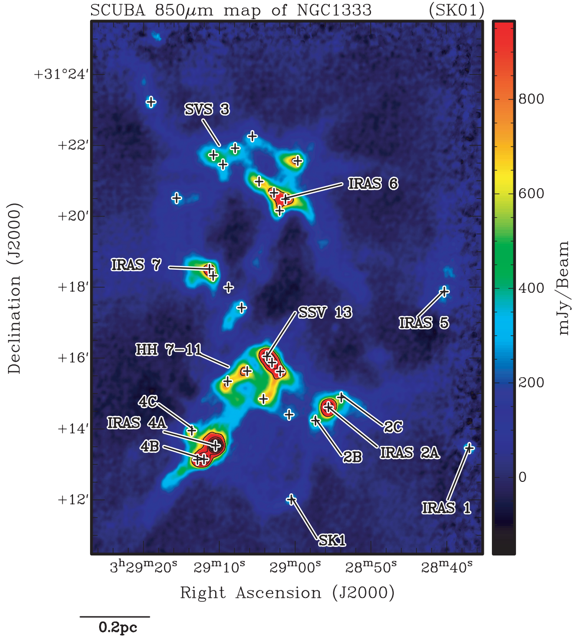
FIGURE 4.1 – Carte du continuum de la poussière à 850 \mu m dans NGC 1333 (Sandell & Knee 2001). Les contours représentent 10%, 20%, 30%, ..., 90% du flux maximum de 6.68 Jy beam ^{-1} . Les symboles + indiquent les positions des sources de continuum SCUBA identifiées par Sandell & Knee (2001).
