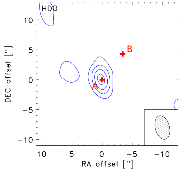
FIGURE 3.5 – Observations interférométriques de la transition HDO à 226 GHz en direction de la proto-étoile IRAS 16293. Le point ( 0'' , 0'' ) a pour coordonnées \alpha_{2000} = 16^h 32^m 22^s.91 , \delta_{2000} = -24^\circ 28' 35.5'' . Figure extraite de Jørgensen et al. (2011).
