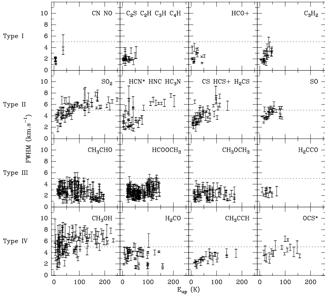
FIGURE 2.10 – Graphes des largeurs à mi-hauteur FWHM en fonction des énergies de niveau supérieur E_{up} des différentes transitions. Les notations HCN^* et OCS^* indiquent que les isotopes principaux de ces espèces n'ont pas été inclus à cause de leur profil non-gaussiens. Les barres d'incertitude à 1\sigma incluent à la fois les incertitudes d'ajustement et de résolution spectrale. Le trait horizontal à 5 \text{ km s}^{-1} correspond approximativement à la moyenne des FWHM . Figure extraite de Caux et al. (2011).
