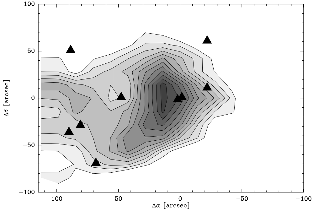
FIGURE A.11 – Carte intégrée en vitesse de la transition de CCH à 87.317 GHz obtenue avec le télescope de l'IRAM. Les contours représentent 0.4, 0.5, ... 1.5 K.km s -1 . Le rms est de 0.2 K.
