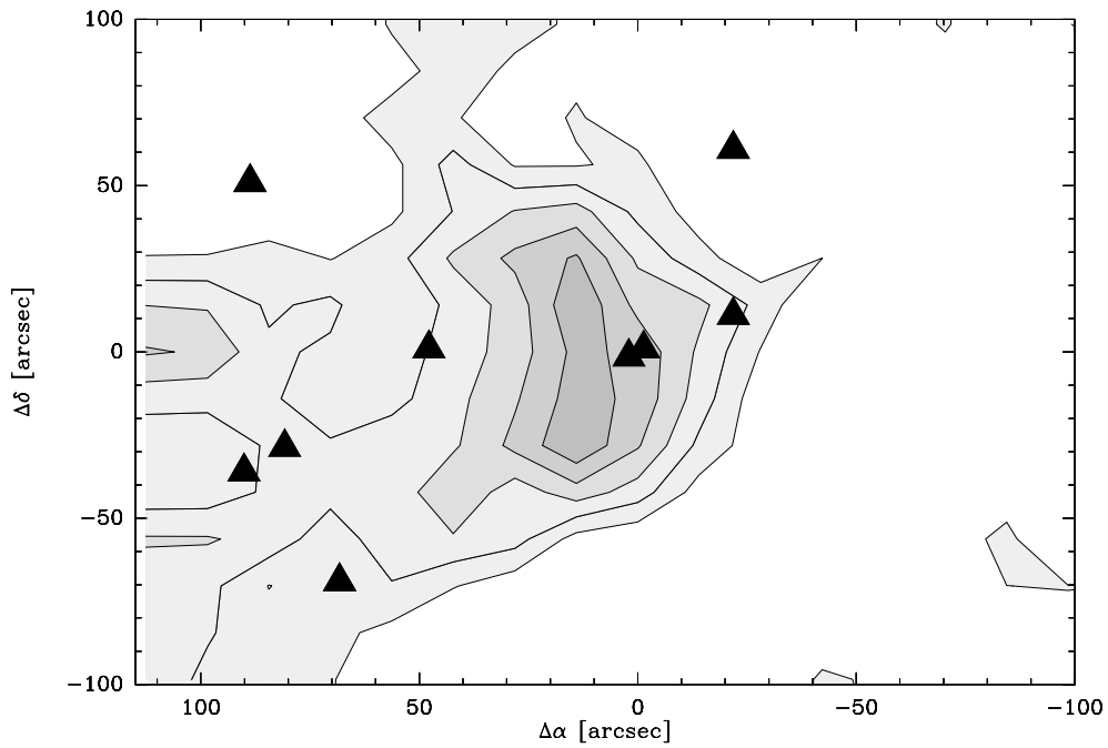
FIGURE A.14 – Carte intégrée en vitesse de la transition de CCH à 87.407 GHz obtenue avec le télescope de l'IRAM. Les contours représentent 0.3, 0.4, ... 0.7 K.km s -1 . Le rms est de 0.2 K.
