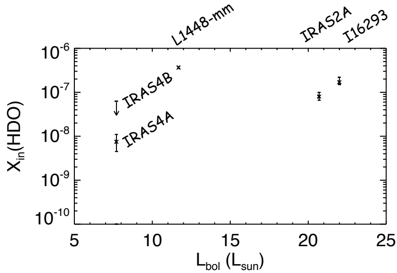
FIGURE 4.14 – Variation de l'abondance interne de HDO en fonction de la luminosité bolométrique des proto-étoiles de faible masse IRAS 16293, IRAS 4A, IRAS 4B ainsi que NGC 1333 IRAS 2A étudiée par Liu et al. (2011) et L1448-mm étudiée par Codella et al. (2010). Les barres d'erreur correspondent aux incertitudes à 3\sigma . L'incertitude sur l'abondance interne de L1448-mm n'est pas connue.
