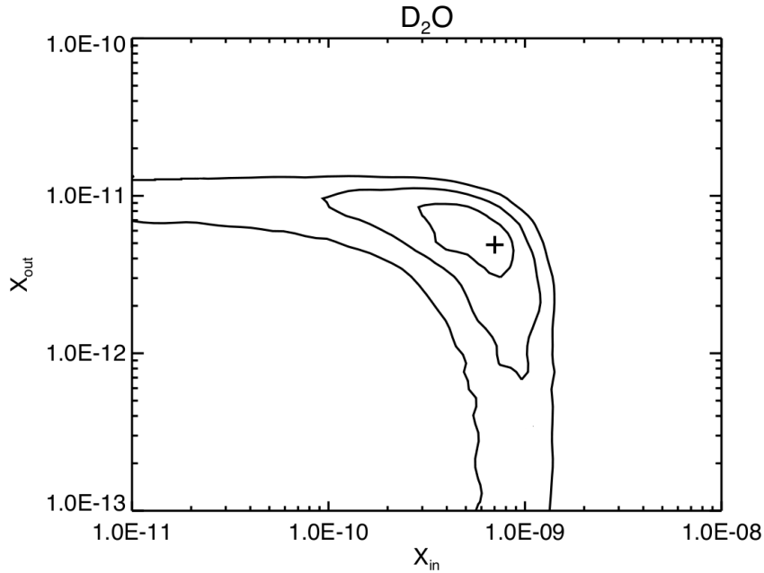
FIGURE 3.22 – Contours de \chi^2 à 1 \sigma , 2 \sigma et 3 \sigma obtenus en ajoutant à la structure une couche d'absorption avec N(\text{para-D}_2\text{O}) = 1.1 \times 10^{12} \text{ cm}^{-2} et N(\text{ortho-D}_2\text{O}) = 1.4 \times 10^{12} \text{ cm}^{-2} . Le meilleur modèle est représenté par le symbole “+” et a été obtenu avec la méthode de \chi^2 n° 2.
