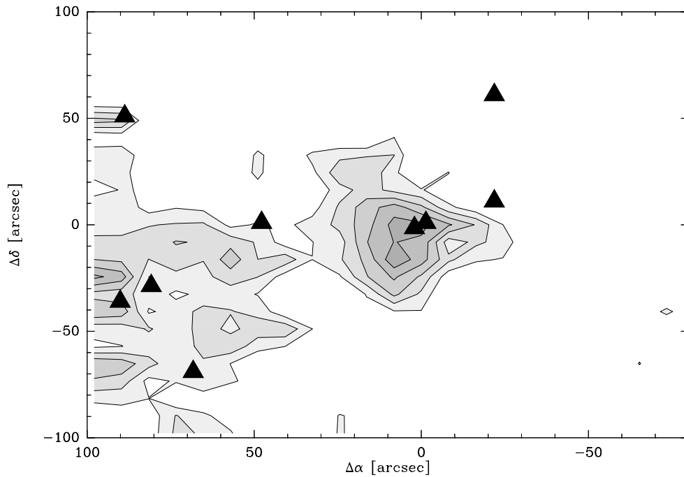
FIGURE A.10 – Carte intégrée en vitesse de la transition de ortho-c-C 3 H 2 à 150.852 GHz obtenue avec le télescope de l'IRAM. Les contours représentent 0.5, 0.7, ... 1.3 K.km s -1 . Le rms est de 0.33 K.
