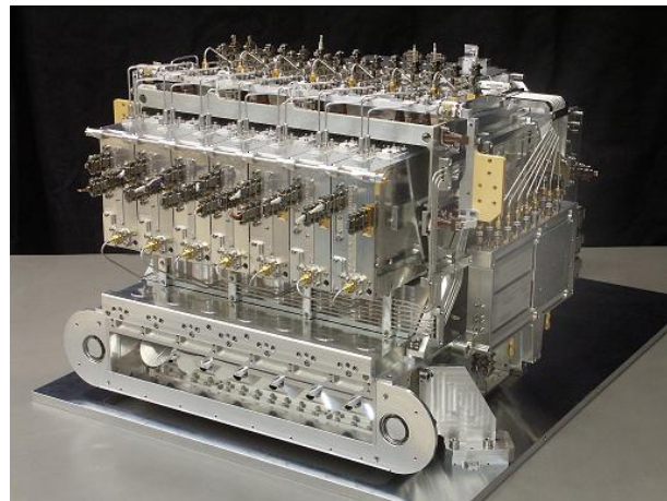
FIGURE 1.14 – Le spectromètre HIFI (Source : her-schel.fr).
