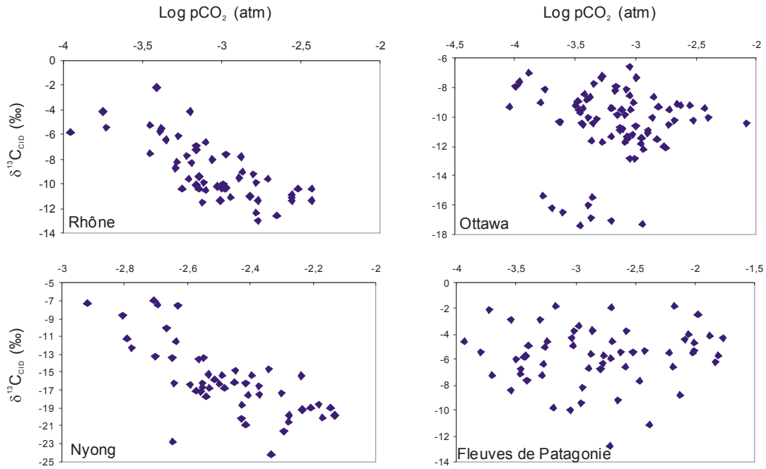
Figure 83 : Relation entre le \delta^{13}C_{CID} (en ‰) et la pCO_2 ( \log pCO_2 en atm) dans les eaux de surface du Rhône (Aucour et al., 1999), de l'Ottawa (Telmer et Veizer, 1999), du Nyong et des fleuves de Patagonie
