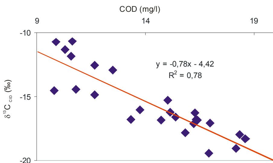
Figure 22 : Relation entre le \delta^{13}\text{C}_{\text{CID}} et la concentration en COD à l'exutoire du bassin du Mengong
