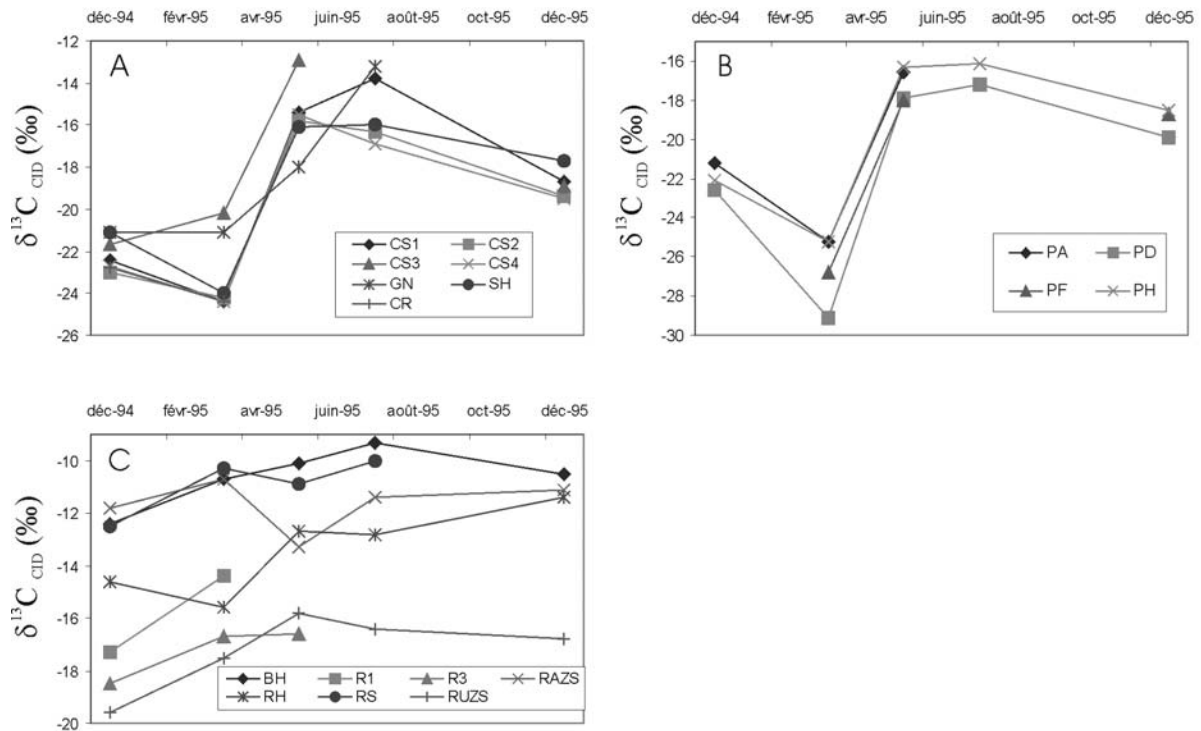
Figure 26 : Variations temporelles du \delta^{13}\text{C}_{\text{CID}} (A) aux sources, (B) dans les piézomètres, (C) dans les ruisseaux au cours des 5 campagnes de prélèvement
