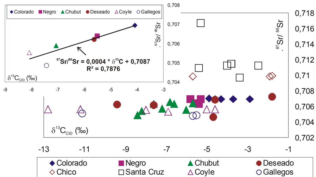
Figure 52 : Relation entre le rapport isotopique du strontium ( ^{87}\text{Sr}/^{86}\text{Sr} ) et le rapport isotopique du carbone inorganique dissous ( \delta^{13}\text{C}_{\text{CID}} ).
