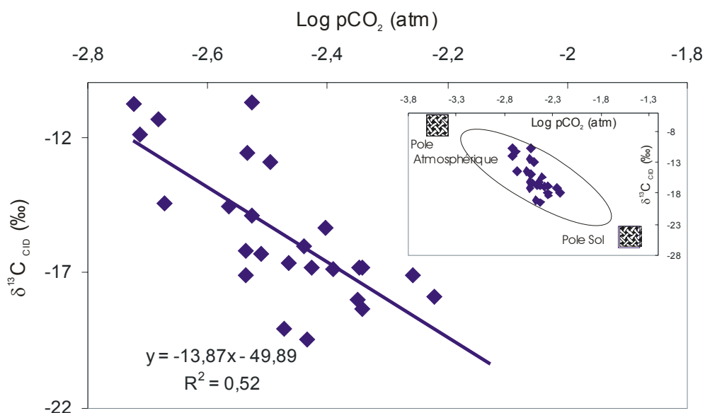
Figure 21 : Relation entre la signature isotopique du CID ( \delta^{13}\text{C} ) et la \text{pCO}_2 dans les eaux à l'exutoire du bassin du Mengong
