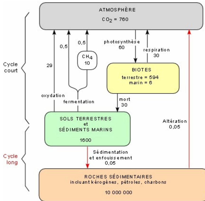
Figure 1 : Cycle du carbone organique. Valeurs en gigatonnes de carbone ( \text{Gt}_\text{C} ). Selon Kump et al. (1999)
