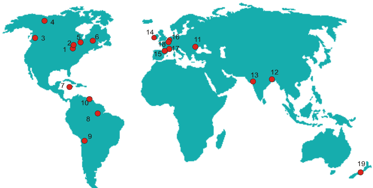
Figure 6 : Localisation des bassins sur lesquels des études du \delta^{13}\text{C}_{\text{CID}} ont été réalisées. Les références des différentes études sont répertoriées dans le Tableau II
