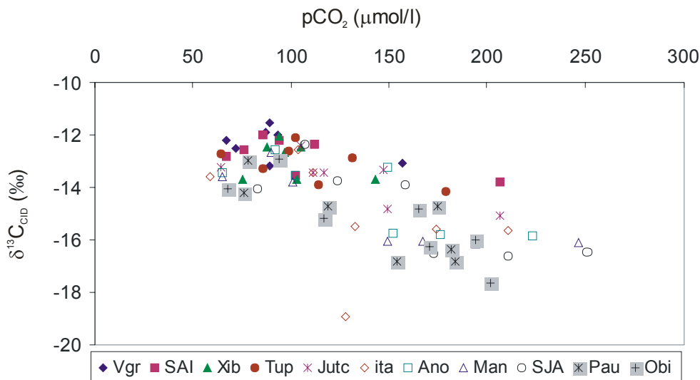
Figure 77 : Relation entre le \delta^{13}\text{C}_{\text{CID}} et la \text{pCO}_2 dans les eaux de surface de l'Amazonie
