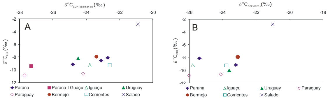
Figure 71 : Relation entre le \delta^{13}\text{C}_{\text{CID}} et le \delta^{13}\text{C} du COP (A) dans les sédiments et (B) dans les MES
