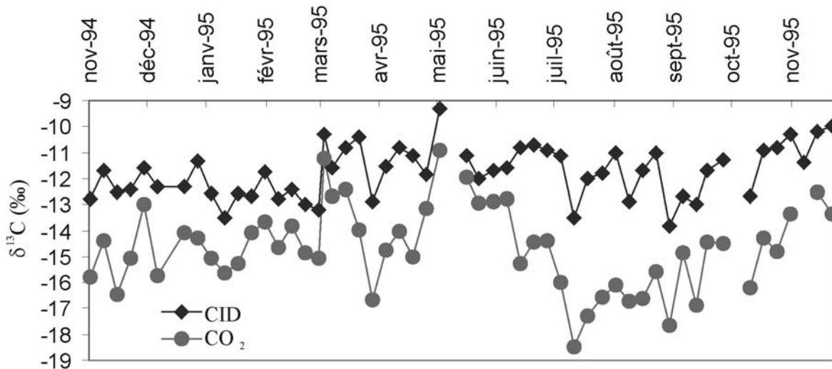
Figure 27 : Variations hebdomadaires du \delta^{13}\text{C}_{\text{CID}} (valeurs mesurées) et du \delta^{13}\text{C} du \text{CO}_2 (valeurs calculées) qui est à l'origine du CID à l'exutoire du bassin versant (RS)
