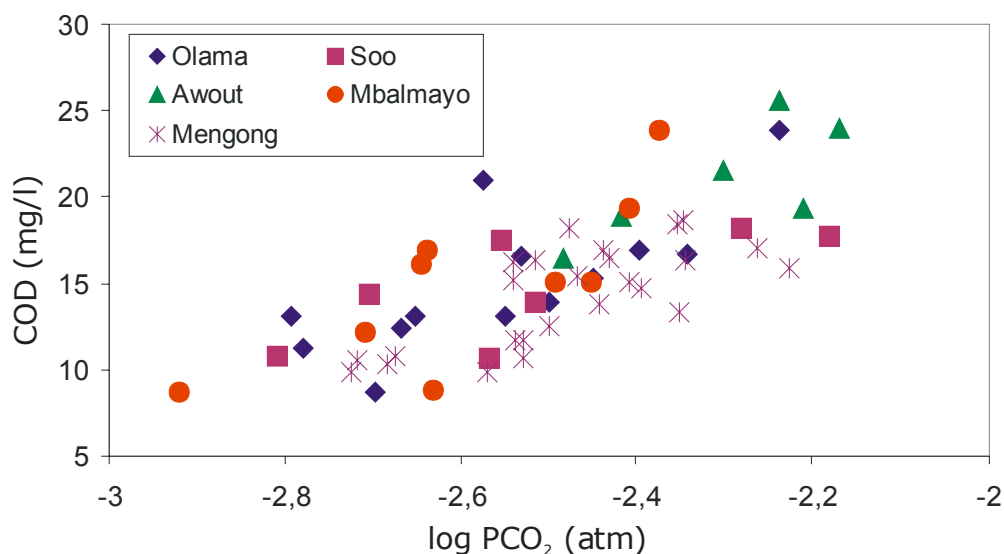
Figure 42 : Relation entre les teneurs en COD et les pCO_2 calculées dans les eaux de surface du Nyong
