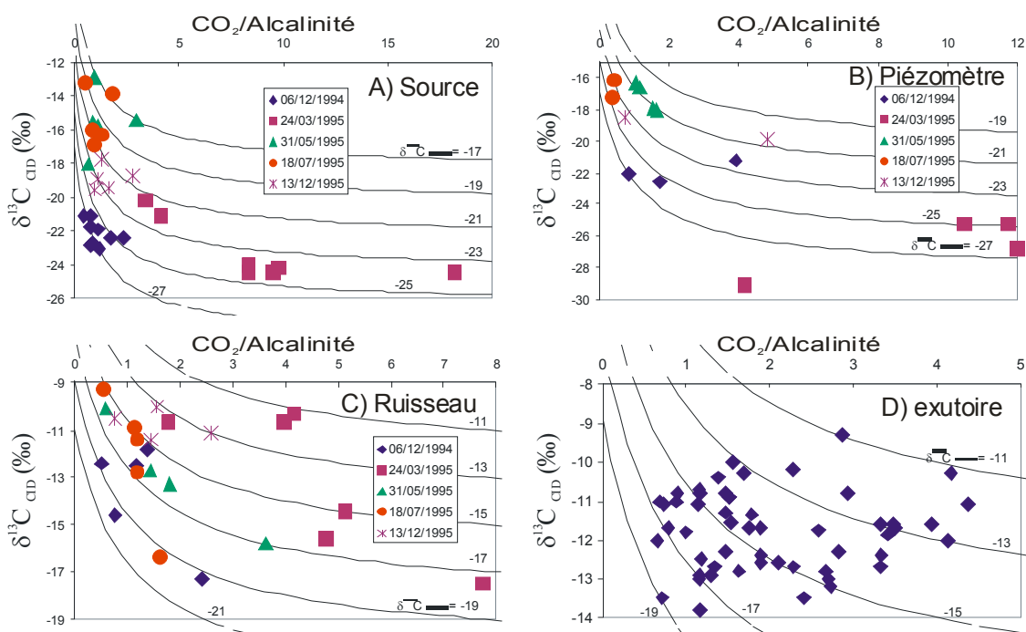
Figure 29 : Relation entre le \delta^{13}\text{C}_{\text{CID}} et le rapport \text{CO}_2/\text{alcalinité} dans les eaux : A) aux sources ; B) dans les piézomètres ; C) dans les ruisseaux et D) à l'exutoire du bassin
