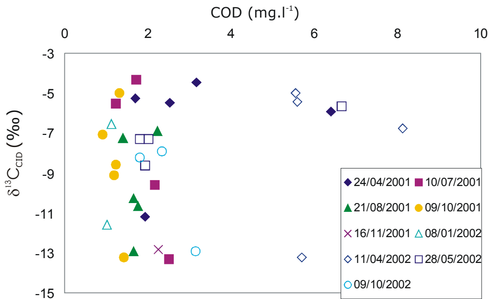
Figure 57 : Evolution du \delta^{13}\text{C}_{\text{CID}} en fonction de la teneur en COD lors des différentes campagnes de prélèvement sur le bassin versant de la Têt.
