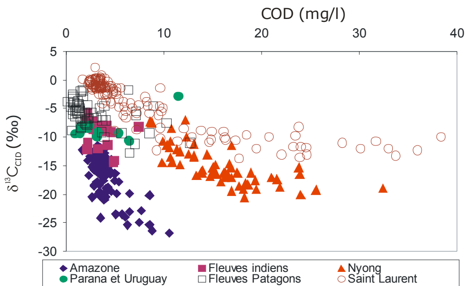
Figure 85 : Relation entre le \delta^{13}\text{C}_{\text{CID}} et la teneur en COD dans les eaux de l'Amazonie, des fleuves indiens, du Paraná, de l'Uruguay, des fleuves de Patagonie et du Saint-Laurent
