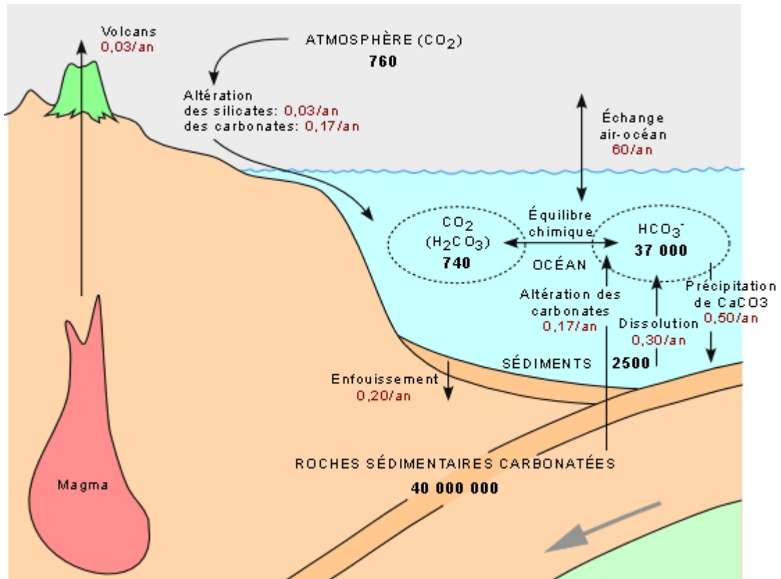
Figure 2 : Cycle du carbone inorganique. Valeurs en gigatonnes de carbone ( \text{GtC} ). Selon Kump et al. (1999)
