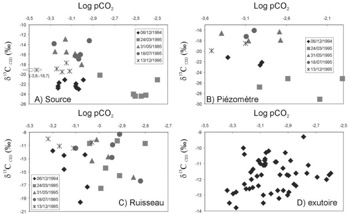
Figure 28 : Variations du \delta^{13}\text{C}_{\text{CID}} en fonction du log de la p\text{CO}_2 dans les eaux : A) aux sources ; B) dans les piézomètres ; C) dans les ruisseaux et D) à l'exutoire du bassin
