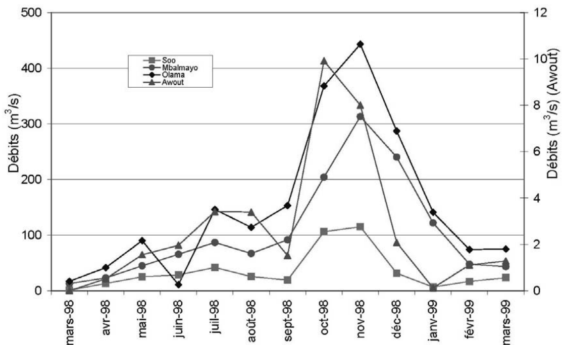
Figure 36 : Variations saisonnières des débits du Nyong aux stations de Olama et Mbalmayo, et de ses affluents, le Soó et l'Awout. L'échelle des débits du Awout se situe sur le côté droit de la figure
