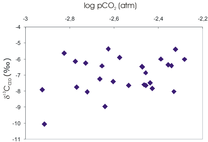
Figure 18 : Relation entre la signature isotopique du CID ( \delta^{13}\text{C} ) et la pCO 2 dans les eaux du Mengong au niveau de la source
