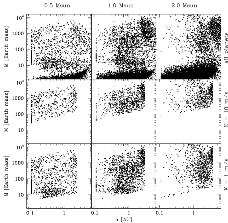
FIGURE 2.3 – Répartition des exoplanètes en fonction de leurs masses et de leur distance à l'étoile. Les planètes géantes se forment loin de leurs étoiles, après la “limite des glaces”. Les planètes de faibles masses sont réparties équitablement. Figure tirée de Alibert et al. (2011).
