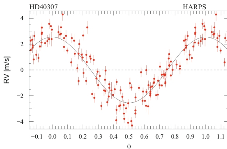
FIGURE 2.5 – Vitesse radiale de l'étoile HD 40307 en fonction de la phase de l'orbite, la période étant de 20.46 jours ici. Mesures réalisées par le spectromètre HARPS à La Silla (Chili). Figure tirée de Mayor et al. (2009).
