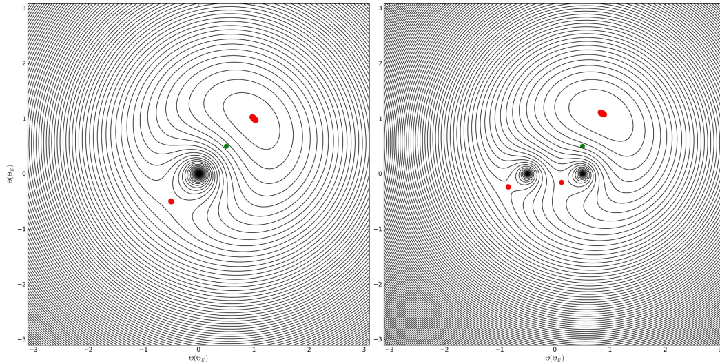
FIGURE 3.3 – Isocontours représentant la surface du retard en temps sur le plan de la lentille. Le point vert représente la position angulaire de la source, les points rouges les positions des images. A gauche, cas d'une lentille simple de 0.3M_\odot centrée. A droite, cas d'une lentille double de masse totale 0.3M_\odot , avec un rapport de masse égal à un et séparées par une distance d'un rayon d'Einstein, dont le centre de masse est centré.
