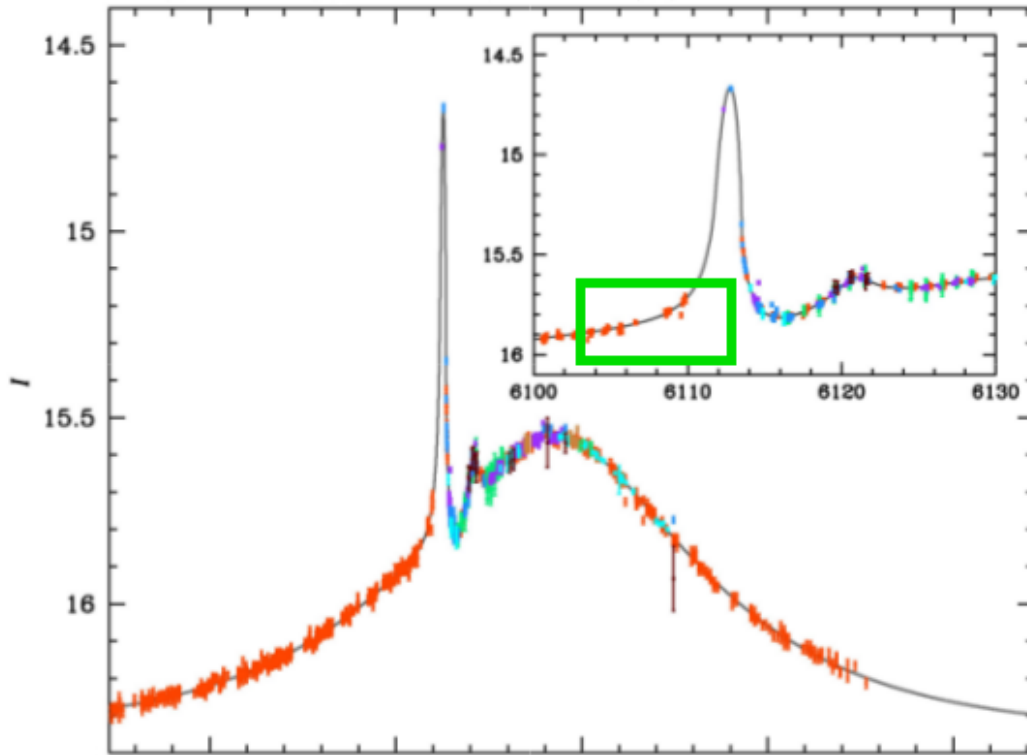
FIGURE 6.4 – Courbe de lumière de l'évènement OGLE-2012-BLG-406Lb. Les points oranges sont les données d'OGLE. Le carré vert indique la date à laquelle PHunter a passé une alerte. Figure prêtée aimablement par CHyeongho Han.
