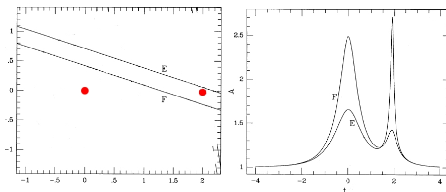
FIGURE 3.25 – Effets d’une source double fixe sur une lentille simple pour deux trajectoires. Sur la figure de gauche, les deux composantes de la binaire sont en rouges, les trajectoires sont dénotées E et F. Les courbes d’amplifications correspondantes sont visibles sur la figure de droite. Il faut noter que l’on considère ici les sources fixes et la lentille se déplaçant, à l’inverse de la convention classique. Figure dérivée de Griest & Hu (1992).
