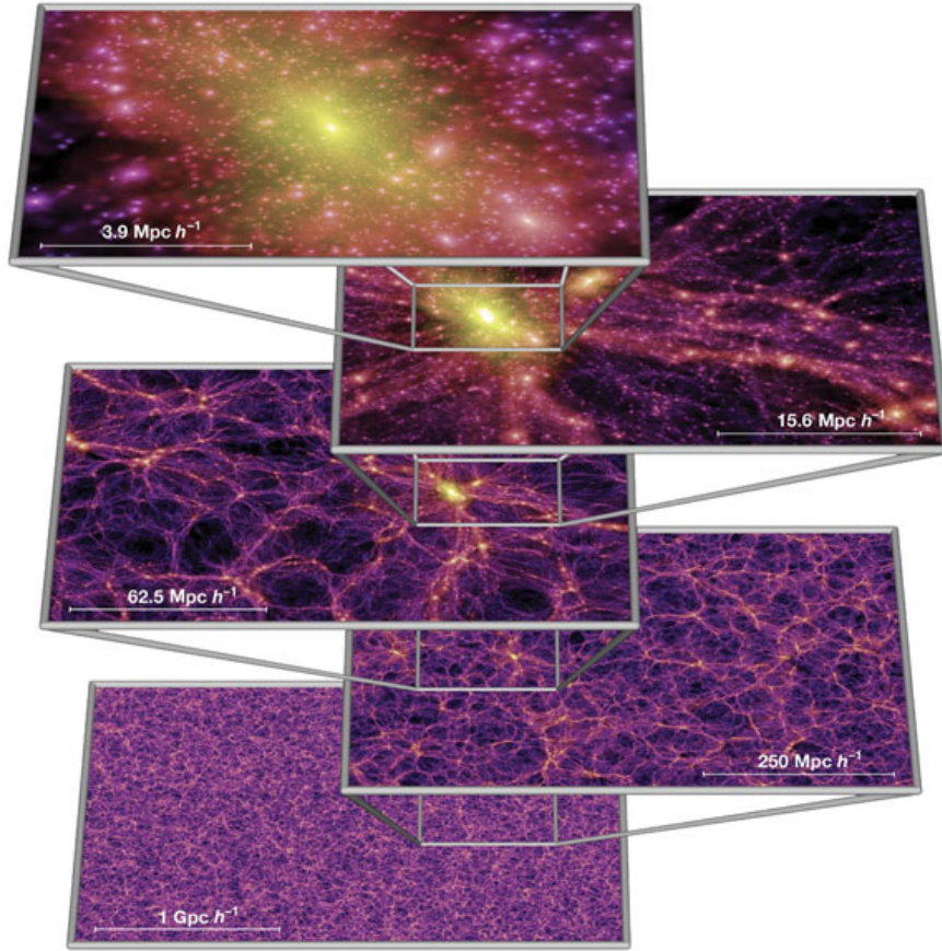
FIGURE 2.2 – Super-structure de matière noire de l'Univers et grossissement progressif dans le sens ascendant. L'image avec le plus fort grandissement représente un amas de galaxies (Springel et al. 2005).
