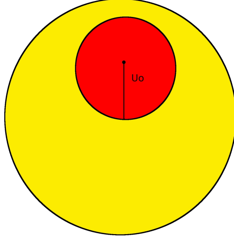
FIGURE 3.17 – Dans les deux schémas, l'étoile source est en jaune, la lentille est représentée par le point noir. Le disque de rayon U_o représente les parties de la source qui sont plus amplifiées que le centre de celle-ci (en rouge). Pour le cas a), la source est relativement éloignée de la lentille. Cependant, une grande part de cette source est plus amplifiée que son centre, les effets de taille finie engendreront une plus grande amplification que le cas source ponctuelle. Dans le cas b), c'est l'inverse qui se produit. Une grande part de la source est moins amplifiée que le centre.
