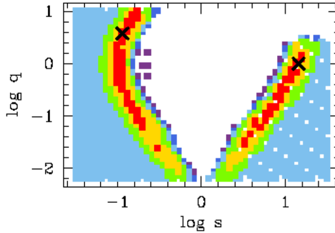
FIGURE 4.12 – Grille d’exploration en s et q pour trouver les minima locaux. Les zones rouges à violet vont de un à six sigma du meilleur modèle. Les deux croix représentent les meilleurs modèles repertoriés dans la Table 4.1. Figure tirée de Bachelet et al. (2012a).
