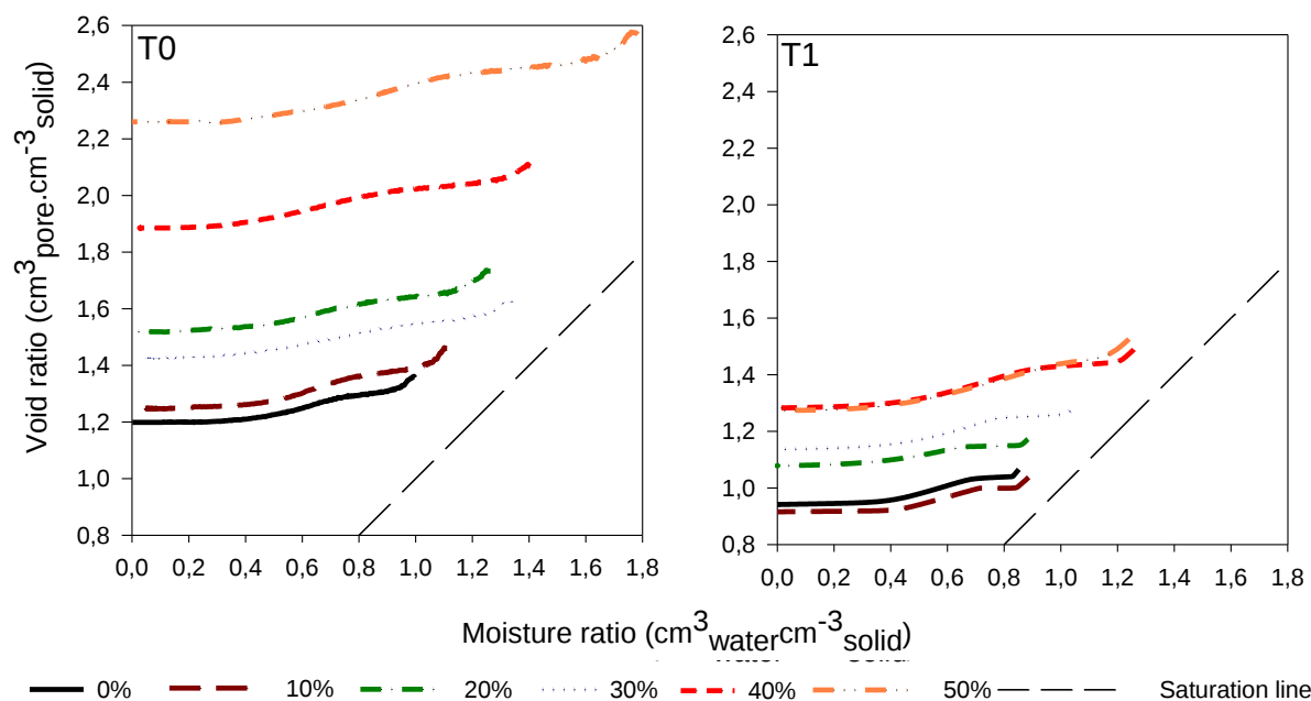
Figure 17 : Comparaison des moyennes des courbes de retrait (4 réplicas) pour les différentes proportions de compost de déchets verts, entre l'état initial (graphe de gauche, T0) et après 5 mois de cycles dessiccation/humectation (graphe de droite, T1).
