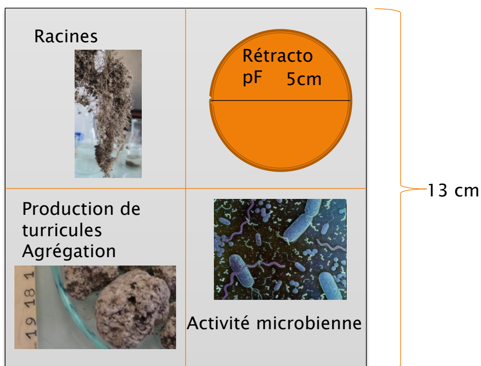
Figure 7 : Ce schéma illustre le protocole de prélèvements de Technosol suivi dans l'expérimentation. Le premier quart est pour l'analyse racinaire, le deuxième quart pour les propriétés hydro-structurales, le troisième quart pour l'analyse de la production de turricules et finalement le quatrième pour l'analyse microbiologique
