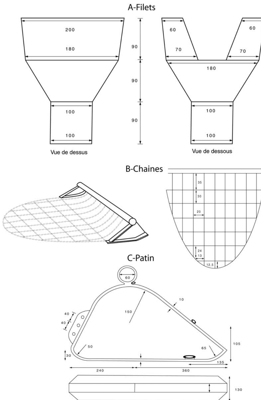
Figure 2.1 3 : Plan du chalut à perche de 2 m d'ouverture horizontale. Les longueurs sont exprimées en centimètres pour les filets et les chaînes et en millimètres pour le patin.
