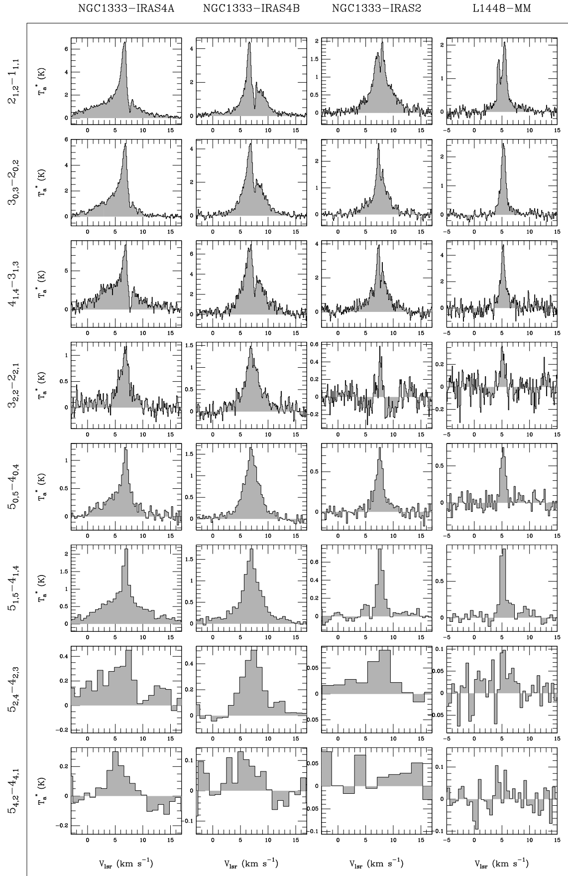
FIG. 5.1 – Spectres des huit raies de H_2CO observées sur NGC1333-IRAS4A, NGC1333-IRAS4B, NGC1333-IRAS2 et L1448-MM
