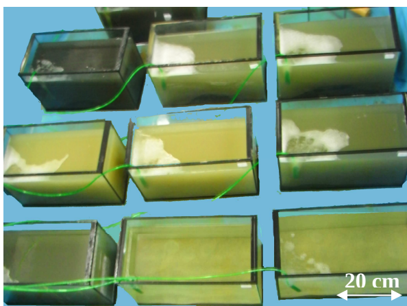
Figure 20 : Conditions d'exposition des juvéniles de turbots (75 mm) aux sédiments issus des trois sites d'étude : un sédiment de wimereux, un sédiment de la vasière nord de la Seine et trois sédiments prélevés dans le port de Boulogne sur mer.
