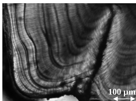
Figure 29 : Otolithe de turbot et ses stries de croissance observées après polissage manuel de l'otolithe.
