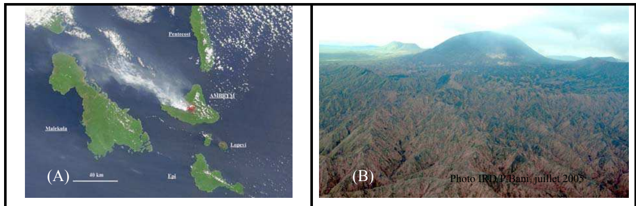
Figure 6-18. (A) Dispersion et dérive du panache d'Ambrym (MODIS 01/10/2004) ; (B) la partie nord-ouest de la caldera où l'on note l'absence de la végétation.
