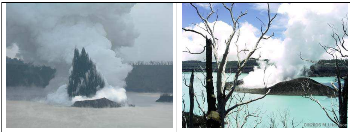
Figure 8-5. Une belle crête dans le lac Vouï, typique d’une activité surtseyenne (photo-gauche, IRD/P.Bani, 4 décembre 2005) et le nouvel îlot après l’éruption (photo-droite, DGMWR/M.Harrison, 17 janvier 2006).
