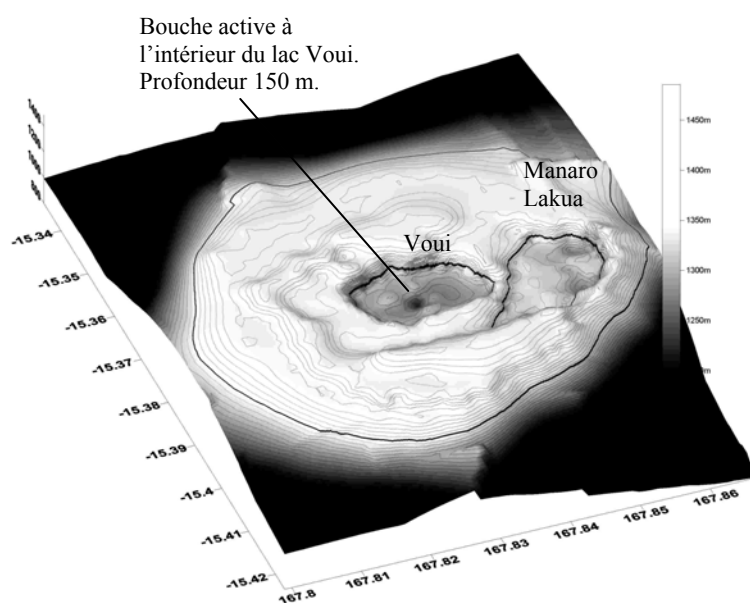
Figure 8-4. Morphologie de la zone sommitale du volcan Aoba associée à la bathymétrie des lacs où la bouche active est mise en évidence dans le Voui.
