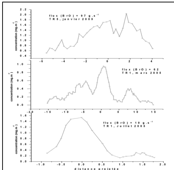
Figure 6-9. La régression du flux de BrO entre janvier et juillet 2005 (en abscisse, la distance projetée par rapport à la direction du panache). En janvier (profil du haut), le BrO a été détecté sur 10 km avec des concentrations qui dépassent le 2 mg.m 2 . En mars (profil du milieu), le BrO a été détecté sur environ 30 km, mais la teneur enregistrée ne dépasse pas ceux du janvier. En juillet (profil du bas), le BrO a été détecté seulement sur 3 km.
