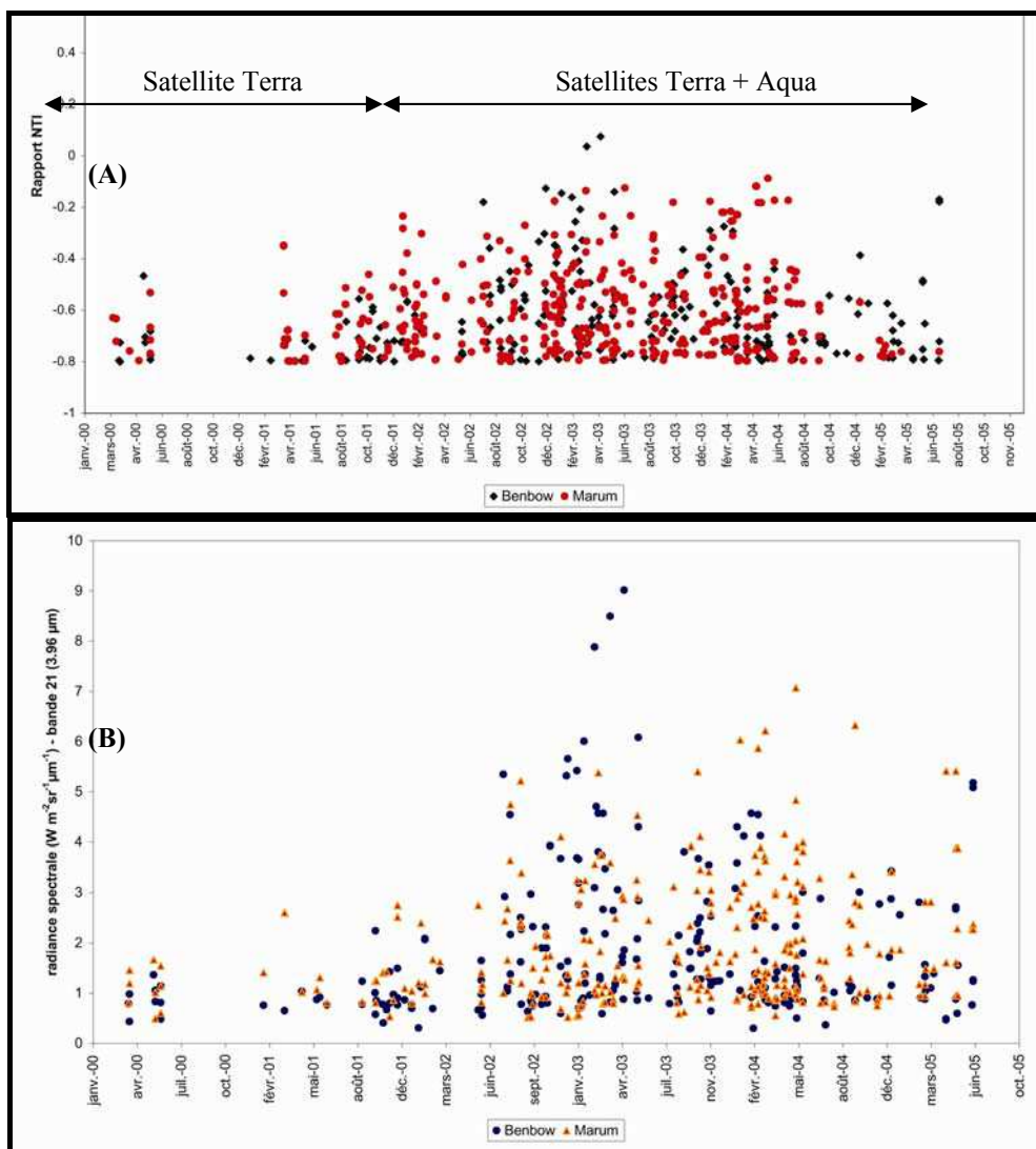
Figure 6-15. (A) Les indices NTI observés sur Ambrym; (B) Evolution de la radiance (bande 21 du MODIS – 3.96 \mu m ). A partir de 2002, on observe une forte radiance thermique sur Ambrym.
