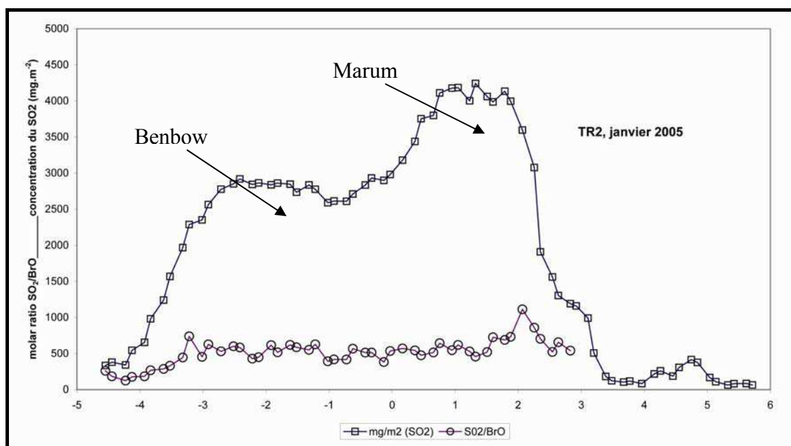
Figure 6-21. Exemple de rapport molaire \text{SO}_2/\text{BrO} restant globalement stable entre 500 et 1000 alors que la concentration du \text{SO}_2 passe de 3000 \text{mg.m}^{-2} sur Benbow à 4500 \text{mg.m}^{-2} sur Marum.
