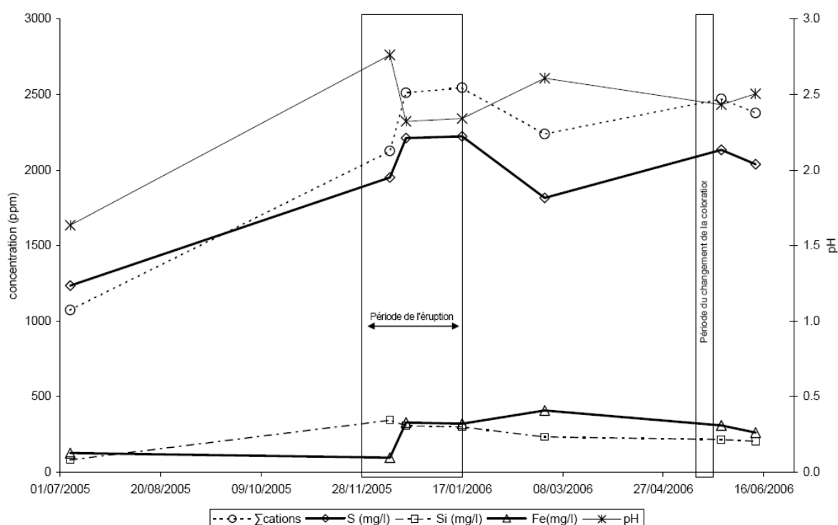
Figure 8-10. Variation de la somme des cations, du pH, du S total, du Fe et du Si dans le lac Vouï entre juillet 2005 et juin 2006.
