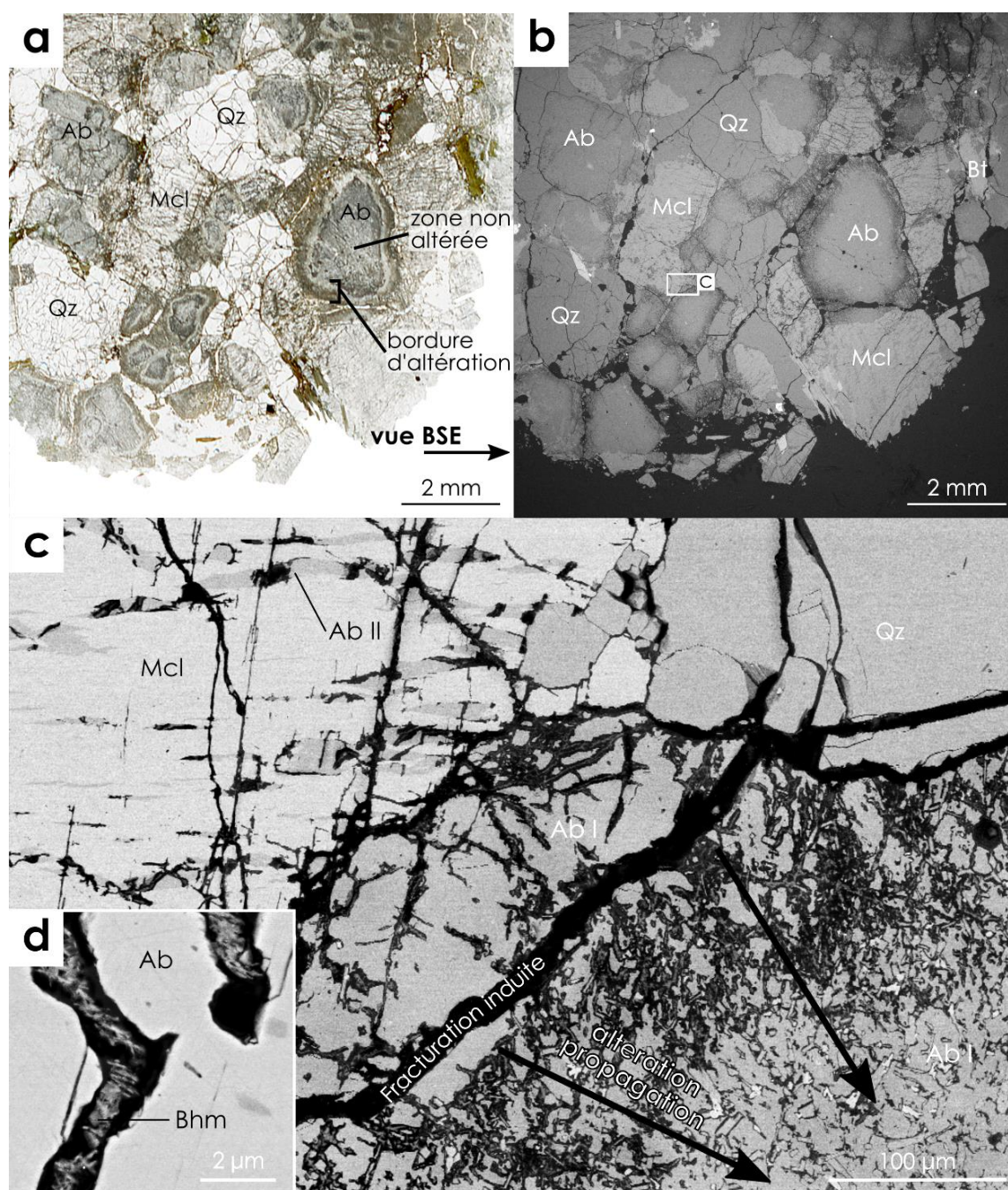
Figure 5.14. Images en microscopie optique (a) et en électron rétrodiffusés (BSE, MEB JEOL, b) en bordure de cylindre (coupe S1) montrant la minéralogie majeure (Ab + Mcl + Qz + Bt) et la texture d'altération en couronne des albites. L'altération expérimentale se caractérise par la propagation isotrope et centripète d'un réseau de micro-fractures (image MEB-FEG, c). Les inclusions (Ser + Msc + Bt) des Ab I dévient ce réseau (c). Les perthites peuvent être altérées par le même mécanisme sans affecter la microcline hôte (c). Ces canaux sont remplis de boehmite suggérant un mécanisme de dissolution/précipitation favorisant la propagation de l'altération par contrainte volumétrique (d). Ab = albite ; Bhm = boehmite ; Mcl = microcline ; Qz = quartz.
