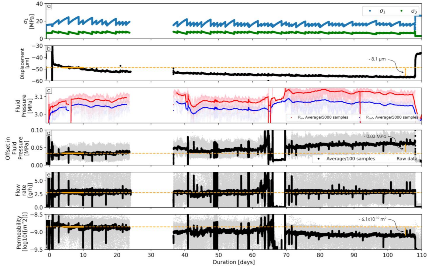
Figure 5.21. Evolution au cours de l'expérience de percolation des paramètres physiques. (a) Pressions de confinement \sigma_1 et \sigma_3 ; (b) déplacement de l'échantillon ; (c) pressions de fluides P_{in} et P_{out} ; (d) offset P_{in} - P_{out} ; (e) débit imposé. La perméabilité (f) est déterminée à partir du gradient de pression et du flux (voir texte). La médiane des valeurs entre les jours 4 et 10 (trait orange plein) est représentée sur l'ensemble des diagrammes respectifs (tirets oranges).
