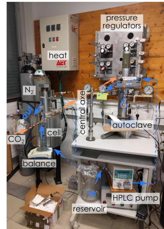
Figure 5.4. Schéma (gauche) et photographie (droite) du système des cellules de percolation. La circulation du fluide est représentée en bleu, celle du CO 2 en orange. Le dispositif présente une deuxième cellule reliée, non montrée sur la photographie. L'axe central d'insertion de l'échantillon est sorti de la cellule. Modifié d'après Le Guen et al. (2007).
