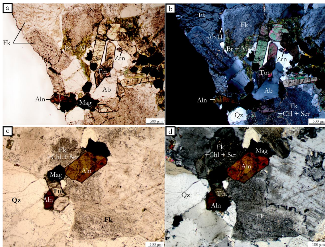
Figure E.1. Microscopie optique du Granite de la Lauzière. Vue générale d'une zone à allanite (Aln) + titanite (Ttn) + magnétite (Mag) + dans une matrice de feldspaths alcalins (Fk) + albite (Ab) + quartz (Qz) en LPNA (a) et LPA (b). Les Fk sont séricitisé (Ser), chloritisé (Chl) ou perthitisé (a et b). Ils sont souvent remplacés en bordure par de l'albite secondaire (Ab II). Beaucoup de joints intergranulaires sont ouverts et remplis de biotite (Bt), de muscovite (Ms) et d'épidote (Ep). Les Ttn sont automorphes, et parfois déstabilisées sur les bordures. Les allanites sont fréquentes, apparaissent en prismes trapus brunâtres légèrement pléochroïques, parfois maclées (c et d).
