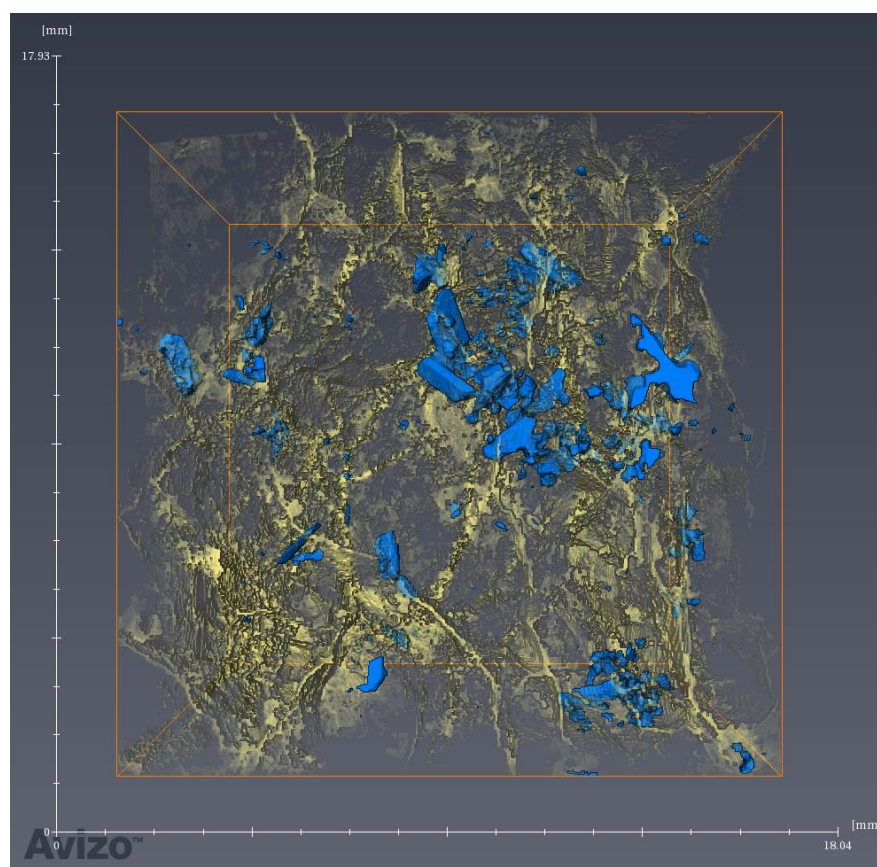
Figure 5.25. Traitement préliminaire des acquisitions d'images obtenues par Tomographie à rayons X sur l'échantillon avant l'expérience de percolation par le logiciel Avizo®. Le réseau de fracture (jaune) est continu et présente de nombreuses interconnexions avec les minéraux accessoires (bleu) porteur des éléments d'intérêts (REE, Th, U).
