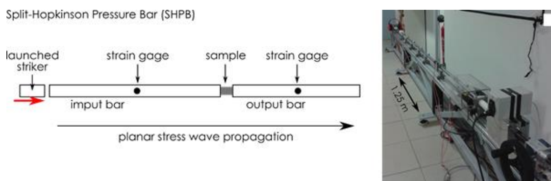
Figure 5.3 Schéma (gauche) et photographie (droite) du système SHPB. Modifié d'après Aben et al. (2017a)
