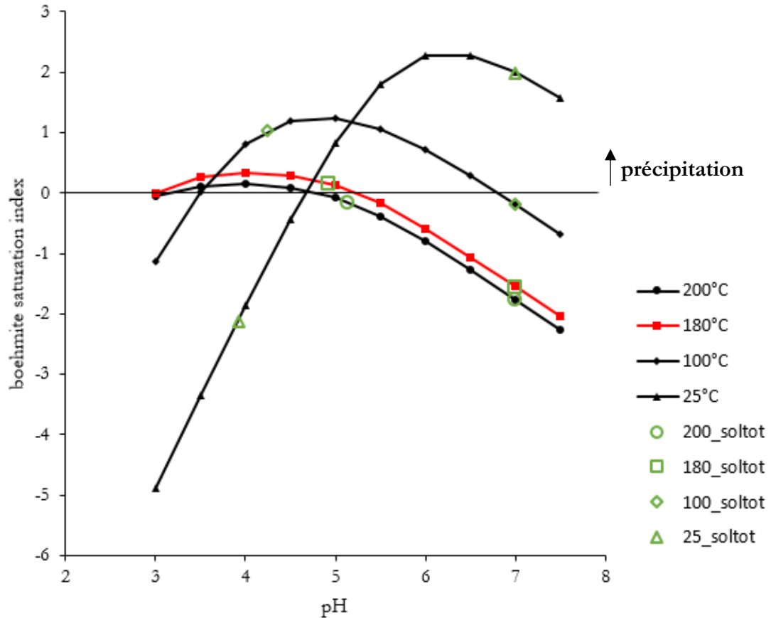
Figure F.1. Indice de saturation de la boehmite en fonction du pH à différentes températures. En trait plein : modélisation pour une solution en batch de composition simple [Al] = 0.6.10^{-6} \text{ mol.L}^{-1} pour différents pH. La température de l'expérience de percolation est 180°C (en rouge); Symboles (vert) : modélisation avec les compositions des fluides sortants (incluant donc tous les éléments) pour pH neutre et pH estimé à partir de l'équilibre avec le CO_2 . Soit un pH de 4-5 dans les conditions de l'expérience.
