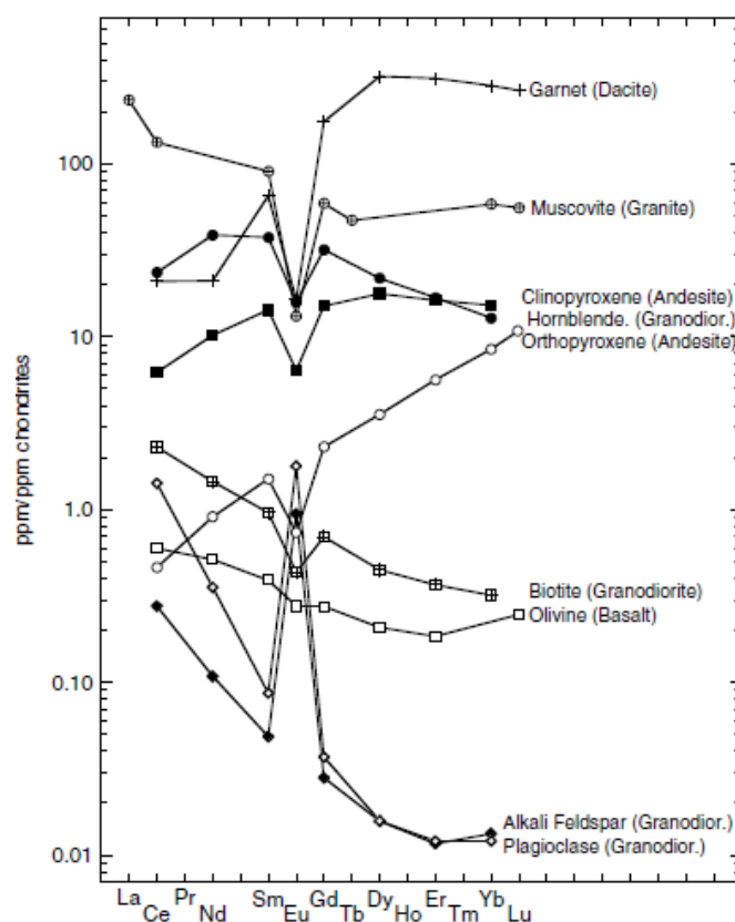
Figure 2.8. Spectres des REE normalisées aux chondrites pour quelques minéraux majeurs. Les roches magmatiques où elles sont respectivement les plus abondantes sont indiquées entre parenthèses. Illustration issue de McLennan and Ross Taylor (2012).
