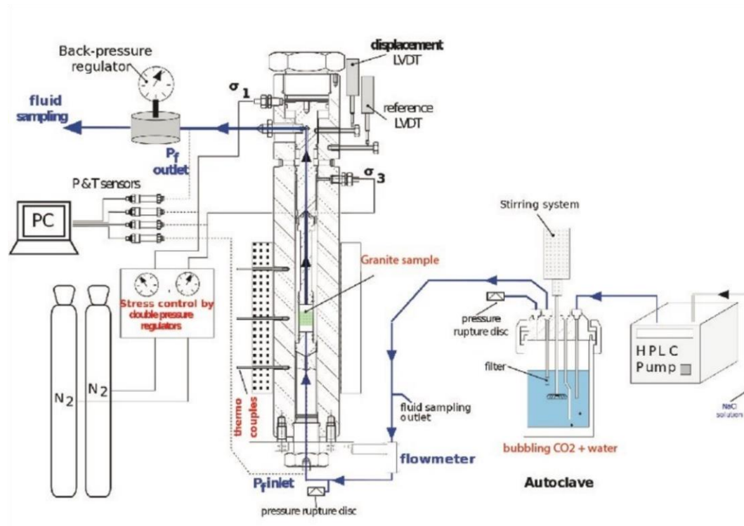
Figure 5.4. Schéma (gauche) et photographie (droite) du système des cellules de percolation. La circulation du fluide est représentée en bleu, celle du CO 2 en orange. Le dispositif présente une deuxième cellule reliée, non montrée sur la photographie. L'axe central d'insertion de l'échantillon est sorti de la cellule. Modifié d'après Le Guen et al. (2007).
