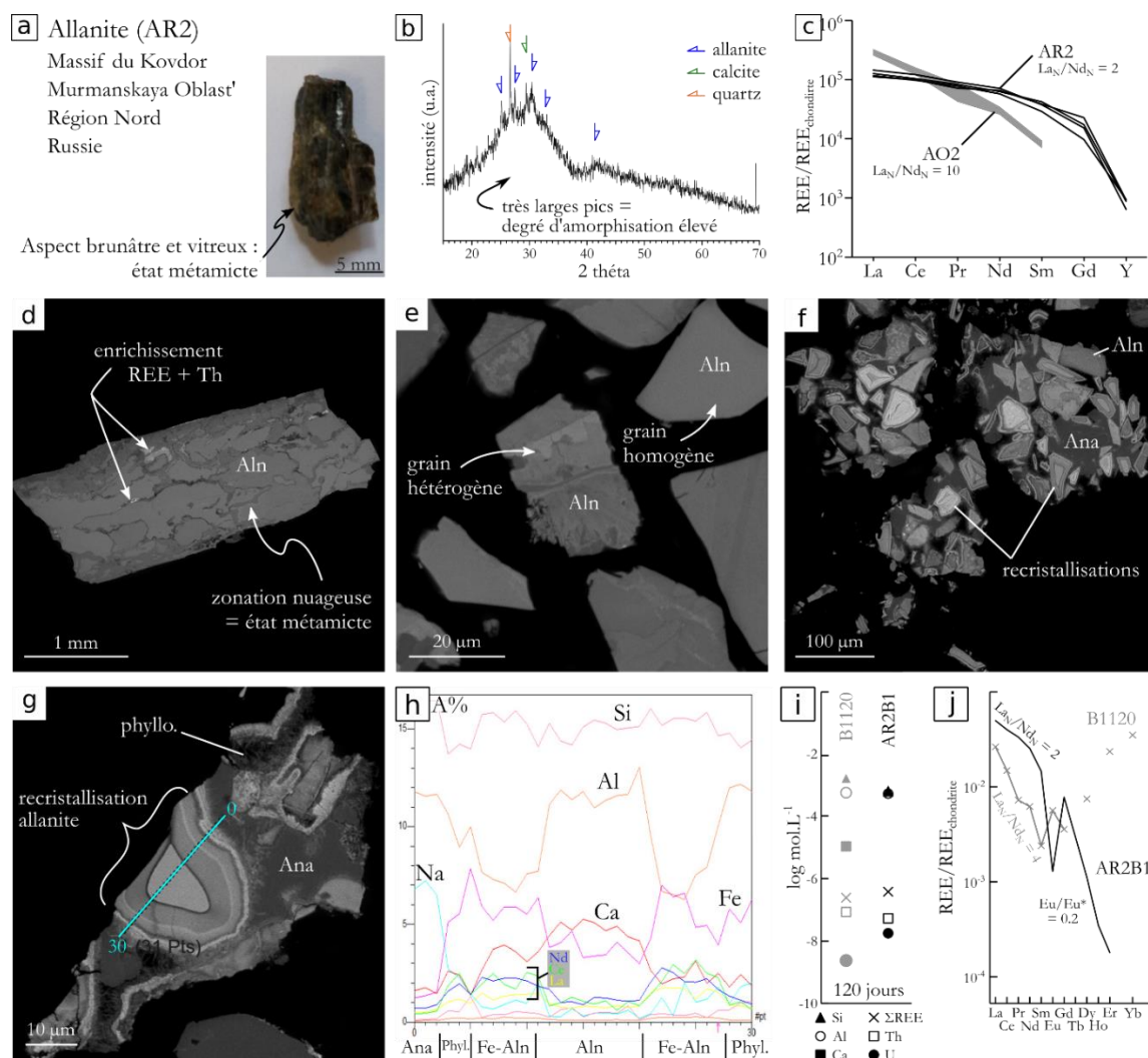
Figure D.1. Allanite métamict AR2 : photographie optique (a) ; diffractogramme (b) ; spectre REE normalisés aux chondrites (noir) comparé à celui de l'allanite cristalline AO2 (gris) par EPMA (c) ; images BSE d'une coupe de AR2 initiale (d) et des grains (20-50 \mu m ) broyés et décarbonatés (e). Résultats de l'altération hydrothermale en réacteur (200°C, 120 jours, fluide = H_2O + CO_2 + NaF ) : image BSE des produits secondaires avec de l'allanite (Aln) non altérée, recristallisée en couches concentriques, de l'analcime (Ana) et des phyllosilicates (Phyllo.) sur les bordures d'allanite (f et g) ; composition en pourcentage d'atome (A%) des recristallisations d'allanite (h). La section analysée est montrée en bleu (g). Compositions des fluides expérimentaux (ICP-MS) : concentrations en Si, Al, REE, Th et U similaires aux expériences B1120 (i). Le Ca est tamponné par la précipitation de calcite + fluorite ; spectre REE normalisé aux chondrite (j) montrant un fractionnement identique à celui de AR2 initiale, mais différents des autres expériences en conditions similaires. Les méthodes XRD, EPMA, MEB et ICP-MS sont similaires à celles décrites dans le chapitre 4.
