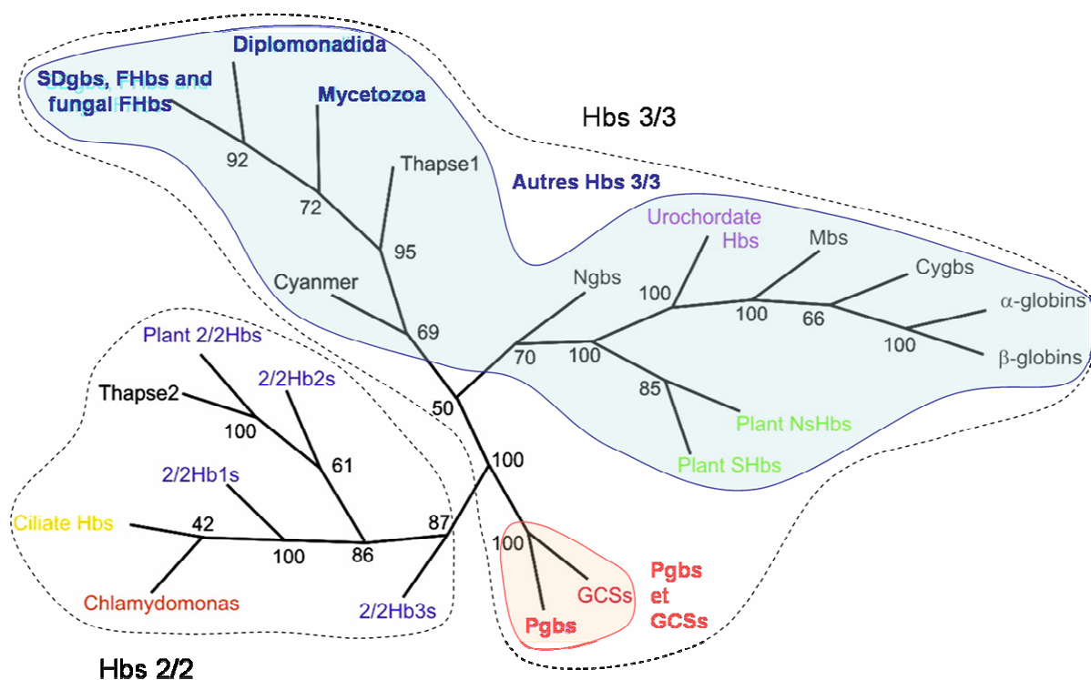
Figure 8 : Arbre phylogénétique présentant les groupes majeurs de globines au sein des trois domaines du vivant. D'après Vinogradov et al. 2005 (Vinogradov et al. 2005).
