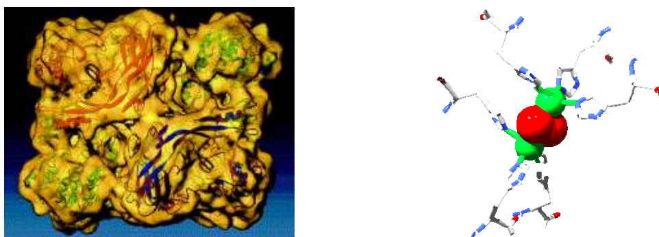
Figure 3 : A gauche : Reconstruction 3D de l'unité de base (Hexamère) de l'hémocyanine de l'arthropode Palinurus elephas : les différents monomères sont colorés en rouge, bleu et vert (Meissner et al. 2003). A droite : Structure du site de liaison à l'oxygène des hémocyanines. Les atomes de cuivre sont représentés en vert, l'oxygène en rouge.
