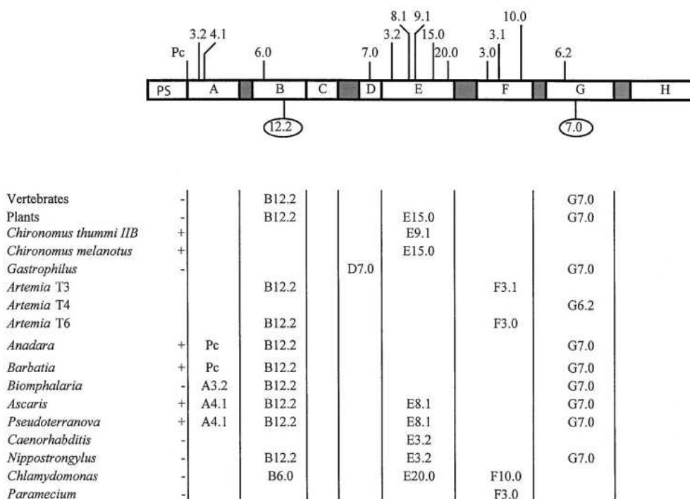
Figure 17: Diversité des positions d'introns au sein des gènes de globines. Les hélices sont désignées de A à H. PS, peptide signal, PC, intron précédant la séquence codante. + et - indiquent la présence ou non d'un peptide signal. B12.2 correspond ainsi à une insertion après le 2 e nucléotide du 12 e codon de l'hélice B. D'après Dewilde et al. (Dewilde et al. 1998).
