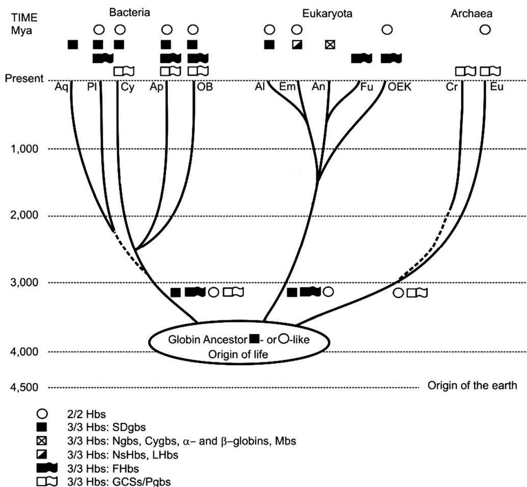
Figure 19 : Distribution des trois lignées de globines au sein des trois domaines du vivant (Archaea, Bacteria et Eukaryota). Les lignes pointillées indiquent des événements dont la date est incertaine. Aq, Aquificales, Cy, Cyanobactérie, Ap, α-protéobactérie, OB, autres bactéries, Al, Algues, Em, Embryophyte, An, Animaux, Fu, Champignons, OEK, Autres Eucaryotes, Cr, Crenarchaeota, Eu, Euryarchaeota. D'après Vinogradov et al. (Vinogradov et al. 2005).
