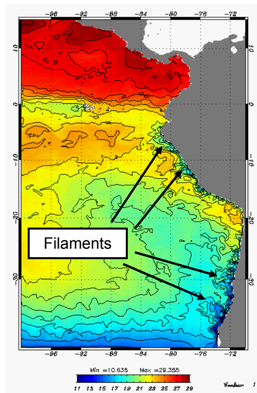
Fig. 1.6: Filaments de sub-mésoéchelle indiqués sur une carte de TSM dans le Pacifique Sud-Est établie à partir de données satellite AVHRR Pathfinder (Vazquez et al., 1995) pour le 1 er janvier 1992. L'unité est le °C. L'intervalle de contour est de 1°C.
