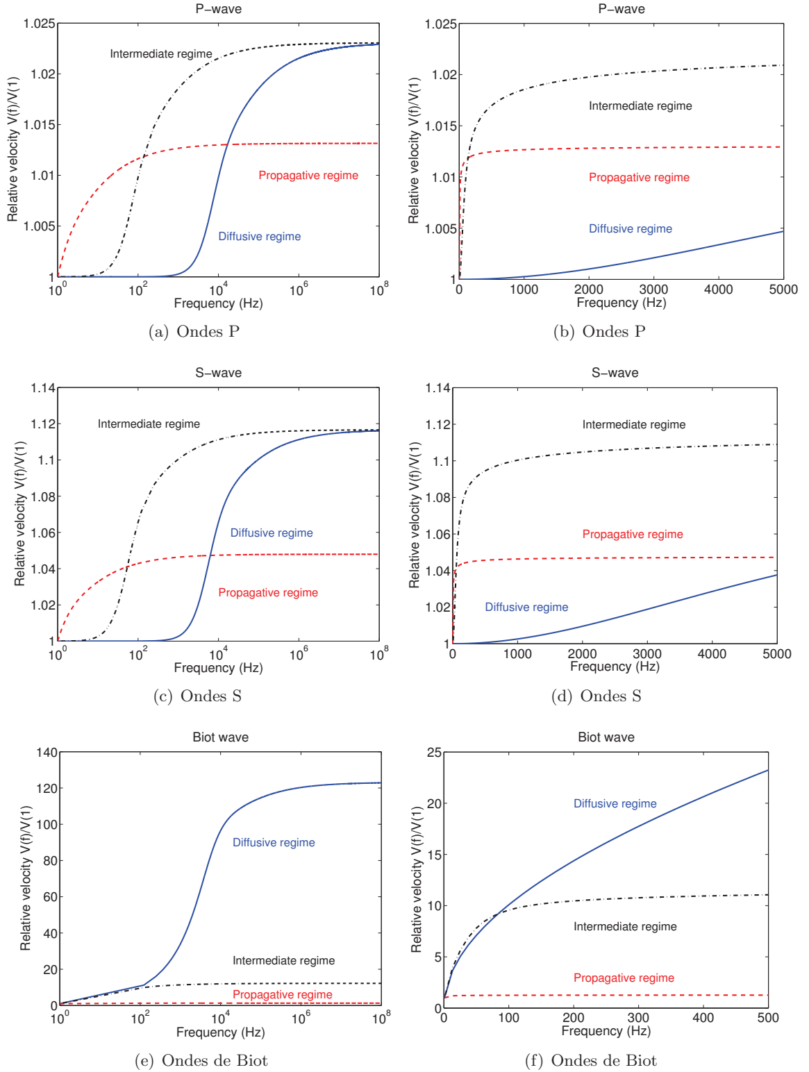
FIGURE 1.2 – Vitesses de propagation relatives à la vitesse à 1\text{ Hz} des ondes P (a,b), S (c,d) et Biot (e,f) en fonction de la fréquence. Les graphiques (b,d,f) sont des zooms entre 1 et 5000\text{ Hz} ( 500\text{ Hz} pour l'onde de Biot) afin d'observer le comportement dispersif à basse fréquence.
