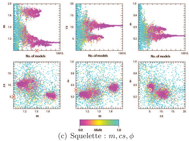
FIGURE 4.8 – Inversion des paramètres poroélastiques à partir des données V_P , V_S , Q_P , Q_S et \rho . (a) Paramètres de la phase fluide : K_f (en GPa ), \eta (en Pa.s ) et \rho_f (en kg/m^3 ), (b) Paramètres de la phase solide : K_s (en GPa ), G_s (en GPa ) et \rho_s (en kg/m^3 ), (c) Paramètres du squelette : m , cs et \phi . Le modèle vrai est représenté par la croix rouge. Chaque graphique représente les valeurs des modèles calculés dans l'espace des paramètres (ou en fonction du nombre de modèles calculés et donc, du nombre d'itérations). La couleur des points dépend de la valeur de misfit obtenue pour le modèle considéré.
