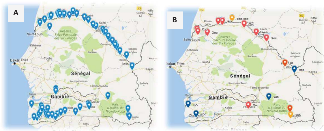
Figure 26 : Carte du Sénégal montrant : A les sites d'échantillonnage et B les sites où Xoo, Xoc et de Xo ont été détectés au Sénégal de 2016 à 2017
