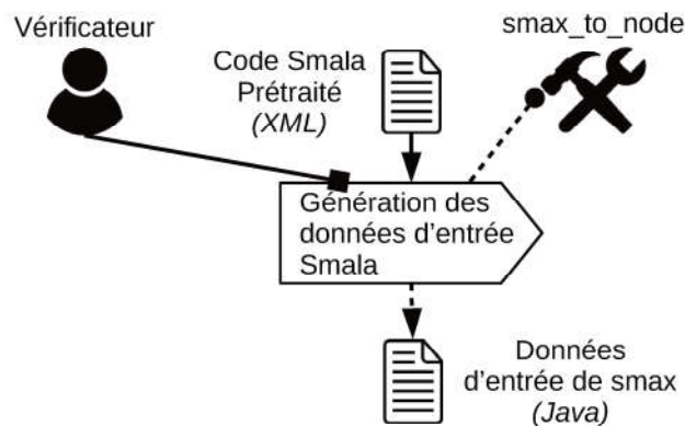
FIGURE 5.5 – Génération des données d'entrée Smala
