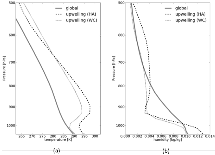
FIGURE 1.9 – Profils de température (a) et d’humidité spécifique (b) moyens dans deux régions d’upwelling (courbes pointillées) au large de la côte californienne (“WC”) et de la Mauritanie en Afrique de l’Ouest (“HA”), et comparaison avec les profils de température et d’humidité moyens globaux sur océan (courbes continues).
