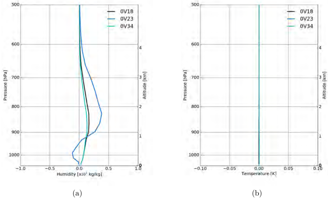
FIGURE 3.15 – Profils de différences sur l’humidité (a) et la température (b) entre l’ébauche et l’analyse 1D-Var, en assimilant successivement chaque fréquence à 18.7 GHz, 23.8 GHz et 34 GHz. Les différences sont moyennées sur l’ensemble des profils et paramètres de surface de la base de données de situations géophysiques.
