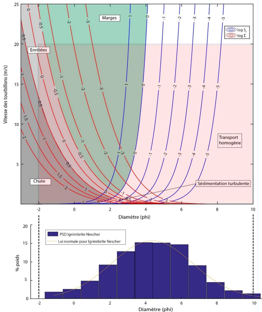
Figure 6.7 : Domaines de stabilité de l'ignimbrite déterminés en calculant le nombre de Stokes et le nombre de Stabilité (Burgisser et Bergantz, 2002). Les conditions explorées dans les expériences (estimations) sont représentées par la zone rose. A partir des travaux de Burgisser et Bergantz (2002) cinq comportements différents des particules dans un fluide en mouvement peuvent être décrits et leurs domaines respectifs ont été représentés.
