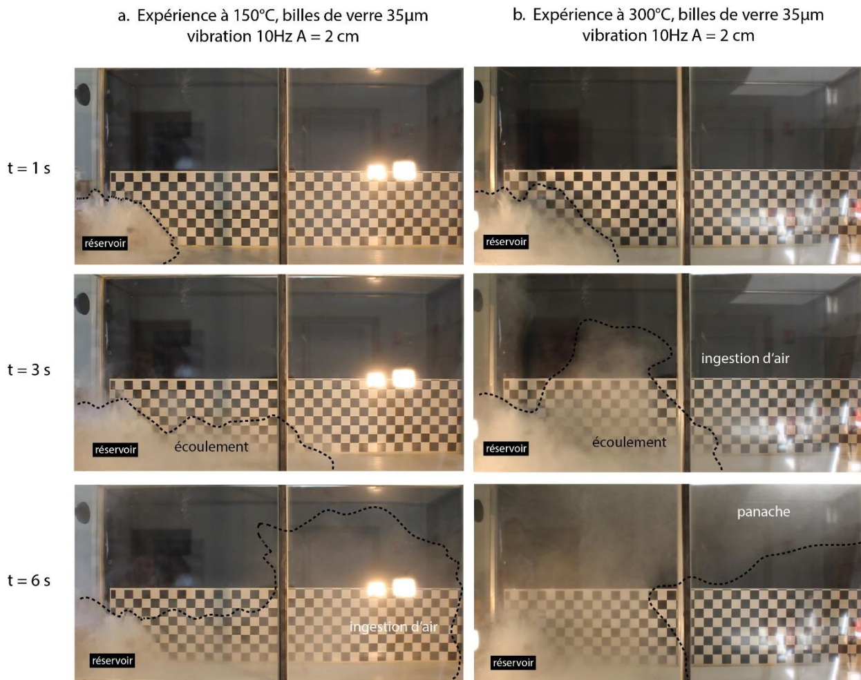
Figure 6.34 : Séquences d'images enregistrées par l'appareil photo à 1, 3 et 6 s après le début des vibrations pour 2 expériences réalisées avec des billes de verre de 35 µm chauffées à des températures différentes : 150°C pour la a. et 300°C pour la b. Pour une meilleure visibilité, les contours des écoulements sont matérialisés par des pointillés noirs.
