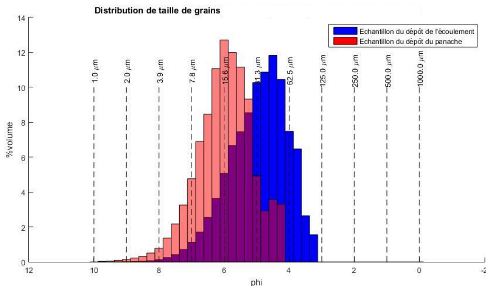
Figure 6.36 : Distribution de taille de grain effectuée à l'aide de l'analyseur G3 pour un échantillon du dépôt du panache (en rouge) et un échantillon du dépôt de l'écoulement (en bleu).
