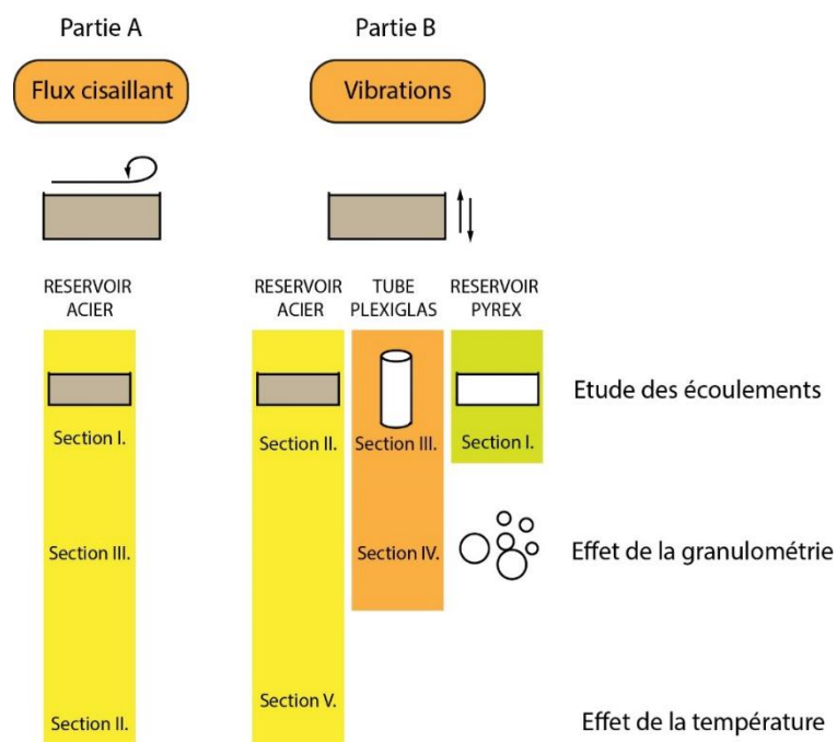
Figure I.1 : Schéma récapitulatif des différents réservoirs utilisés pour étudier les mécanismes de formation des déferlantes. Chacun de ces réservoirs est utilisé pour étudier une partie du mécanisme, précisée sur la partie droite.
