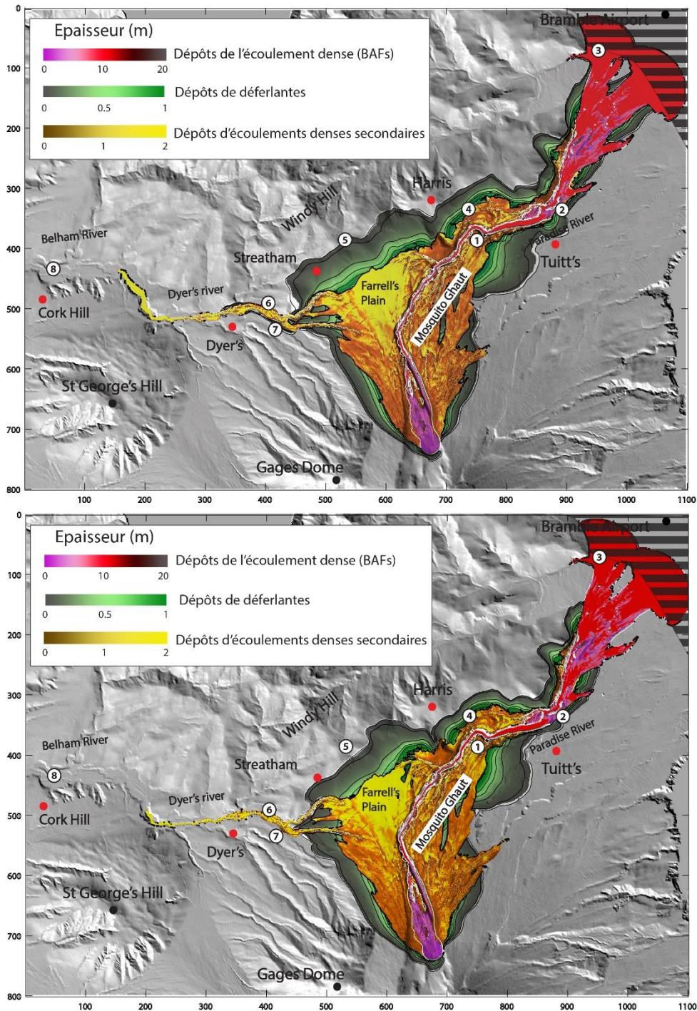
Figure 7.5 : Résultats des simulations pour l'éruption du 25 juin 1997 avec la loi au cube en haut (c.f. chapitre 5), puis la loi à seuil en bas. Pour les deux cas de figure, l'écoulement dense est simulé par une rhéologie plastique. Les principaux paramètres contrôlant la dynamique sont compilés dans les tableaux sur la partie gauche.
