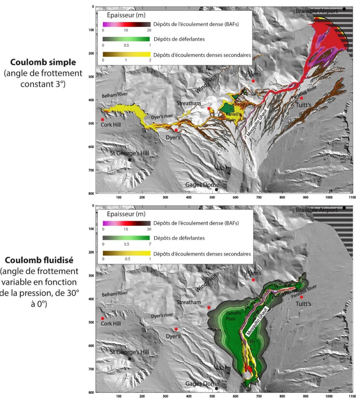
Figure 7.7 : Comparaison des résultats de simulation pour l'éruption du 25 juin 1997 à Montserrat avec en haut une rhéologie de Coulomb simple (réalisée au chapitre 5) et en bas avec la rhéologie de Coulomb fluidisé réalisée dans la partie précédente
