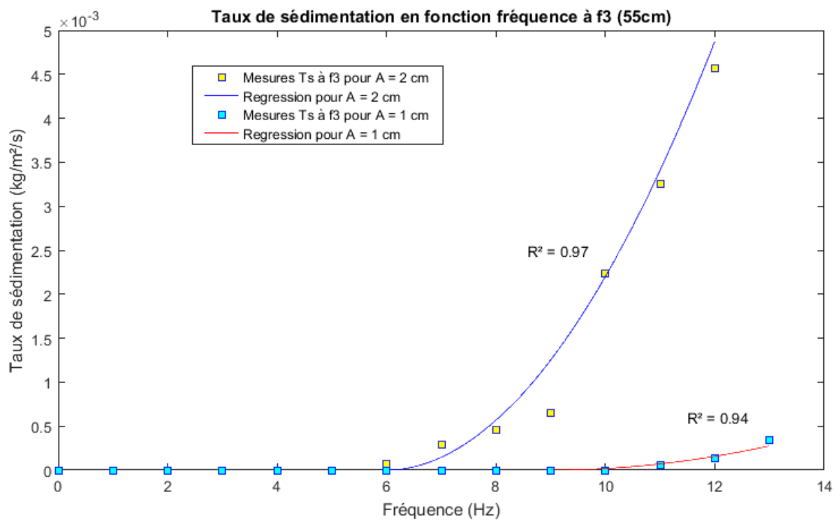
Figure 6.27 : Evolution du taux de sédimentation sur la feuille n°3 à 50 cm du réservoir, en fonction de la fréquence. Les courbes bleues et rouges correspondent à la loi empirique imitant l'allure générale des mesures, pour respectivement A=2 cm et A=1 cm.
