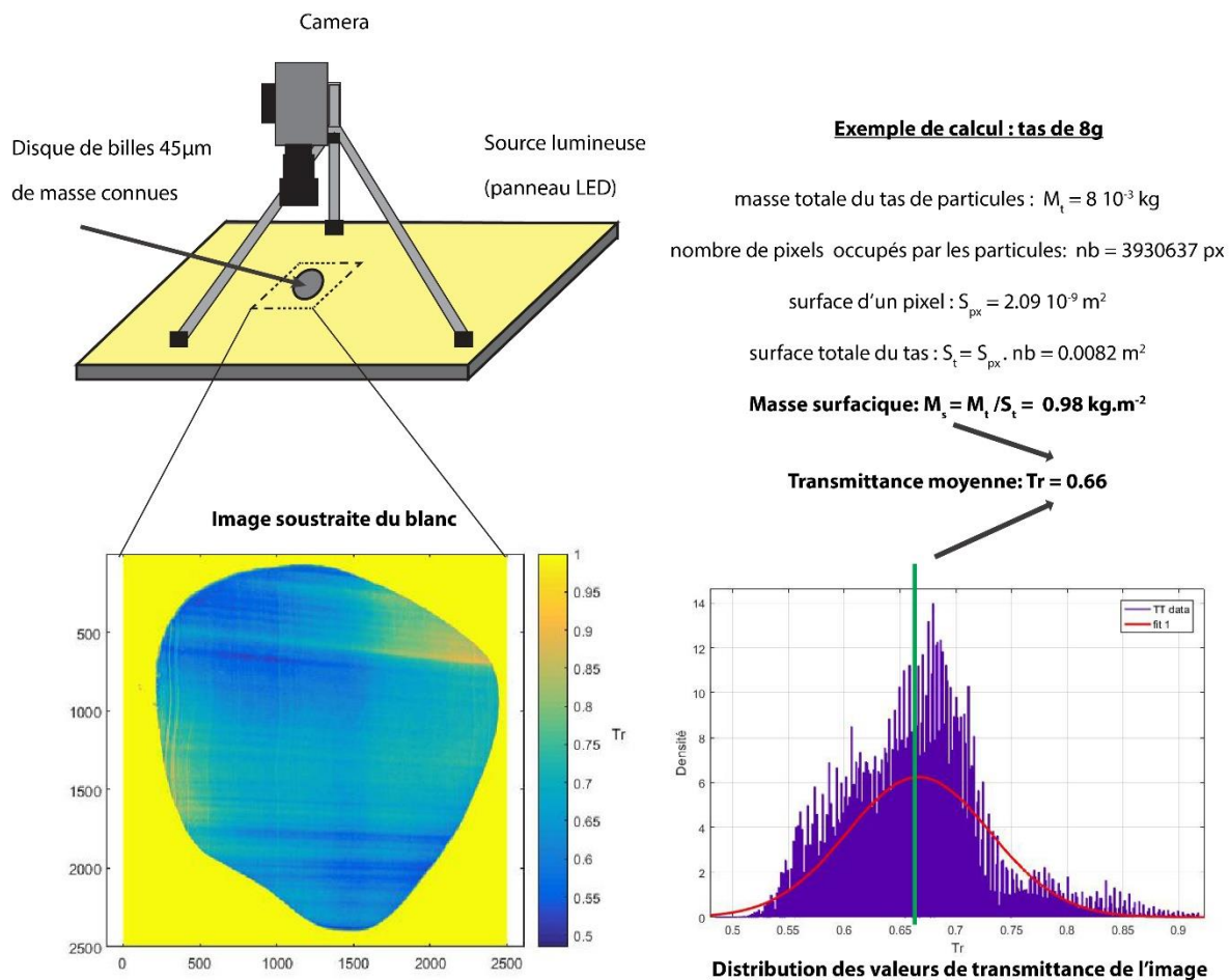
Figure 3.8 : Schéma de la méthode d'étalonnage. Le schéma en haut à gauche montre le positionnement de l'appareil photo par rapport au tas de particule. L'image de ce tas obtenue est traitée pour obtenir les transmittances (en dessous) dont leur distribution statistique est approchée par une loi normale (en bas à droite). La moyenne de la loi donnera la valeur de transmittance du tas associée à la masse surfacique moyenne du tas (en haut à droite).
