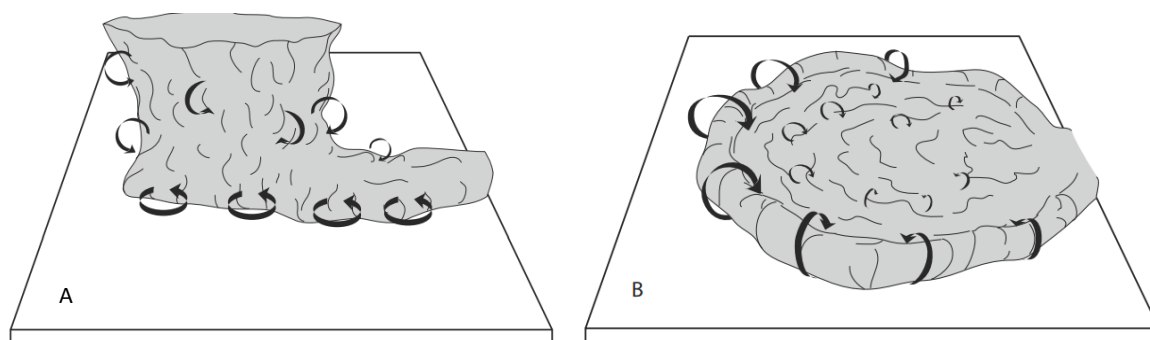
Figure 3.2 : Schéma des expériences de Andrews (2014) pour un écoulement chaud qui s'élève (en A) et un écoulement froid qui s'étale radialement (en B).
