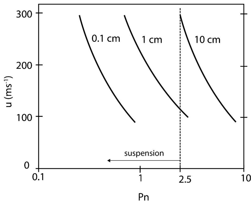
Figure 2.4 : Diagramme d'évolution du nombre de Rouse en fonction de la vitesse d'un écoulement de gravité pour 3 tailles de particules : 0.1 cm, 1 cm, et 10 cm. Le seuil de suspension théorique est symbolisé par la ligne pointillée ( Pn = 2.5 ). Modifié d'après Valentine (1987).
