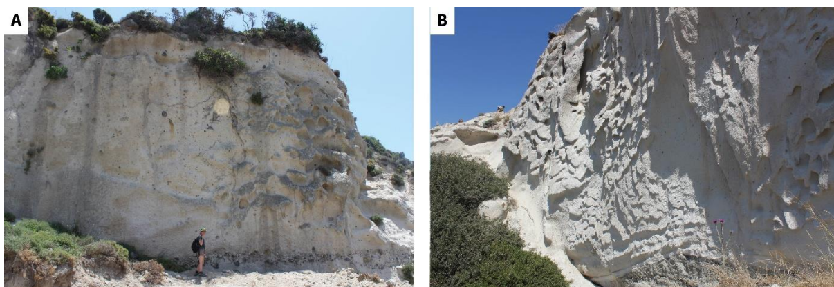
Figure 1.5 : Ignimbrite de l'île de Kos (Kos Plateau Tuff) en Grèce avec en A la partie supérieure de l'ignimbrite (couche 2) et en B la base de l'ignimbrite (première unité, début de la couche 2) dont le contact avec le sol est visible. (Photo 2017 VG).
