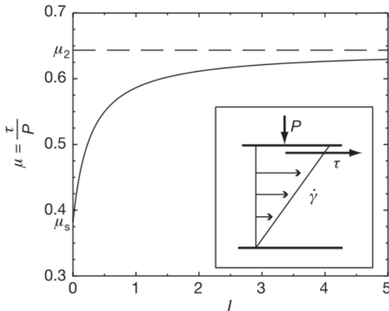
Figure 2.8 : Coefficient de friction \mu(I) en fonction du nombre d'inertie I . L'orientation de la contrainte normale P et de la contrainte cisailante \tau est aussi représentée dans le carré central. La variation de vitesse sur l'épaisseur correspond au taux de cisaillement \dot{\gamma} . D'après Jop et al. (2006).
