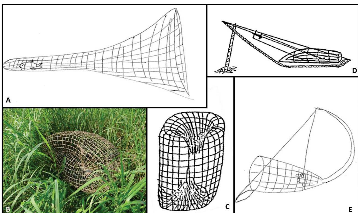
Planche photographique 3-4. Une grande diversité de nasses (n°2)
