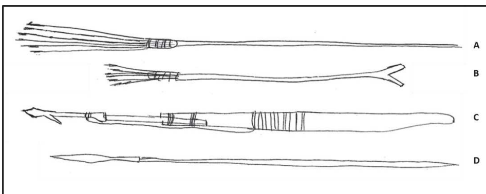
Planche photographique 3-7. Une grande diversité des harpons (n°2)
