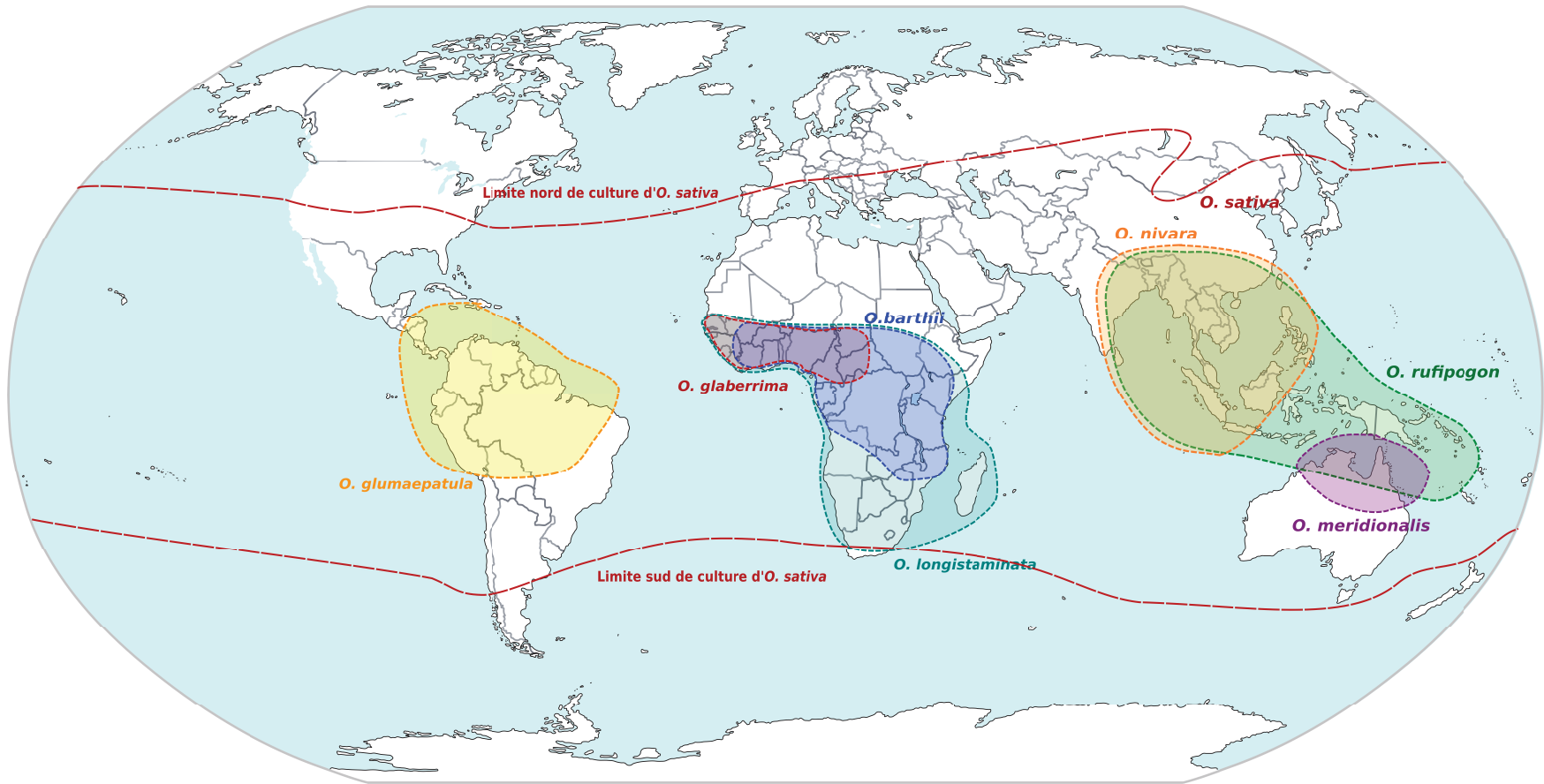
FIGURE 1.14 – Distribution mondiale des espèces du génome AA du genre Oryza (adapté Ashikari and Matsuoka (2006)).
