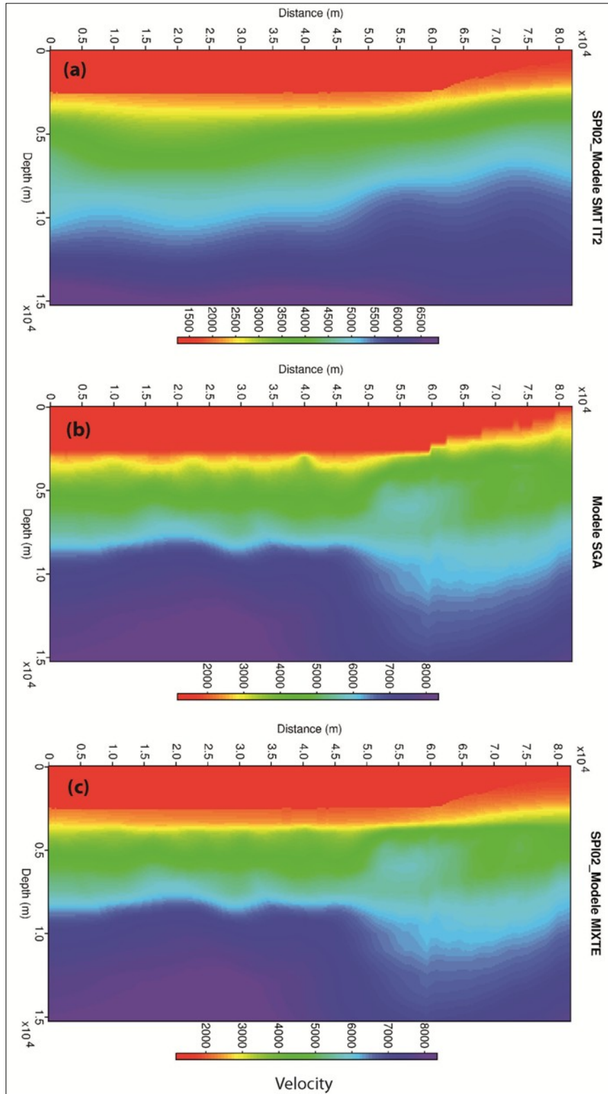
Figure IV.3 : (a) Macro-modèle de vitesse (MV2) après correction de (MV1) via une analyse de vitesse dans le domaine profondeur. (b) Macro-modèle de vitesse (MV_OBS) par inversion des temps d'arrivées (voir la section inversion des données OBS). (c) Macro-modèle de vitesse mixte (MV_MIX).
