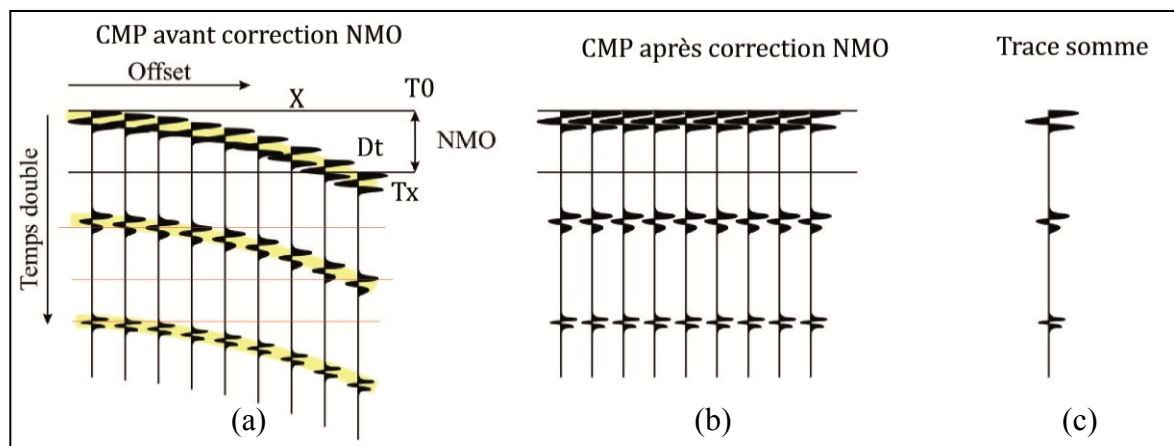
Figure II.18 : Schéma illustratif du principe des corrections NMO (Mari et al., 2001 modifié).
