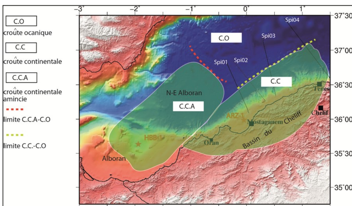
Figure V.17. Carte schématique simplifiée des zones potentiellement prospectives pour l'exploration pétrolière. Les deux zones sont entourées en blanc et concernent : (1) en mer la partie Nord-Est du bassin d'Alboran et la partie croûte continentale du secteur de Mostaganem définie en partie sur le modèle tomographique de vitesse calculé sur le profil de grand angle Spi02 et étendue sur les profils SMT Spi01, Spi03, Spi04 2. (2) à terre, la zone concerne le bassin du Chélif. HBB-1 : puits Habibas, ARZ-1 : puits stratigraphique au large d'Arzew. La limite C.O- C.C.A est d'après Medaouri et al. 2014.
