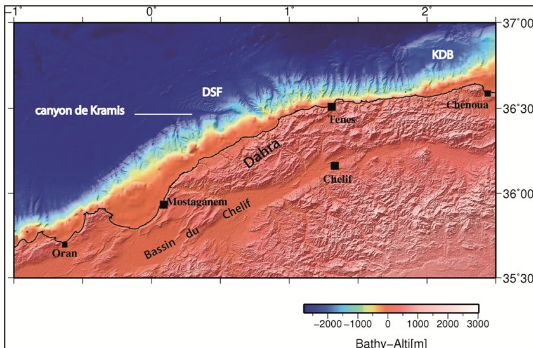
Figure I.2 : Carte morpho-bathymétrique de la marge algérienne dans le secteur de Mostaganem. KDB: banc de Khayr-Al-Din. DSF=Deep-Sea-Fan de Kramis.
