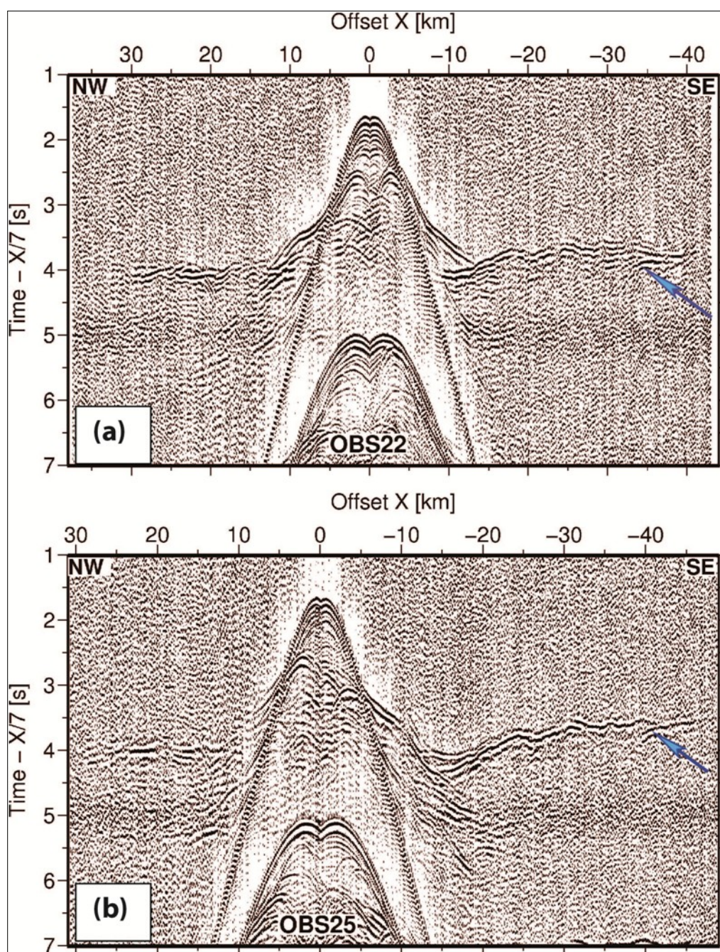
Figure III.9 : Exemples de sections sismiques grand angle (composantes hydrophones) (a) OBS-22 (b) OBS-25, montrant les ondes réfléchies au Moho (flèches bleues).
