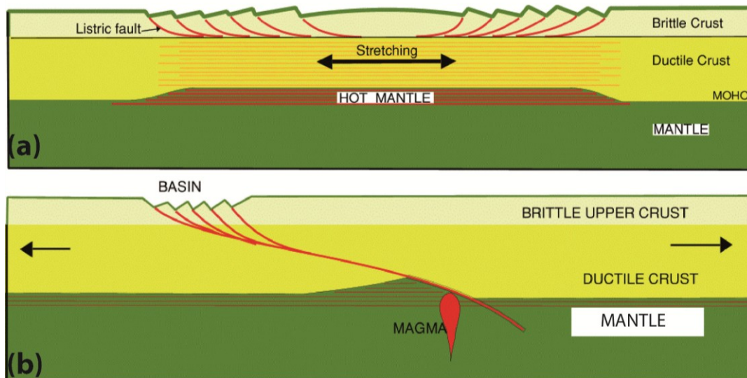
Figure 3. Modèles de rifting : (a) modèle de cisaillement symétrique (McKenzie, 1978), (b) cisaillement simple (Wernicke, 1985). (Repris de HDR, F. Klingelhoef, 2009).
