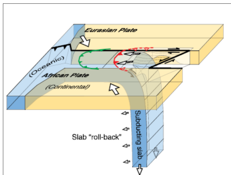
Figure I.12 : Modèle géodynamique pour la mer d’Alboran. (D’après Gutscher (2004)).
