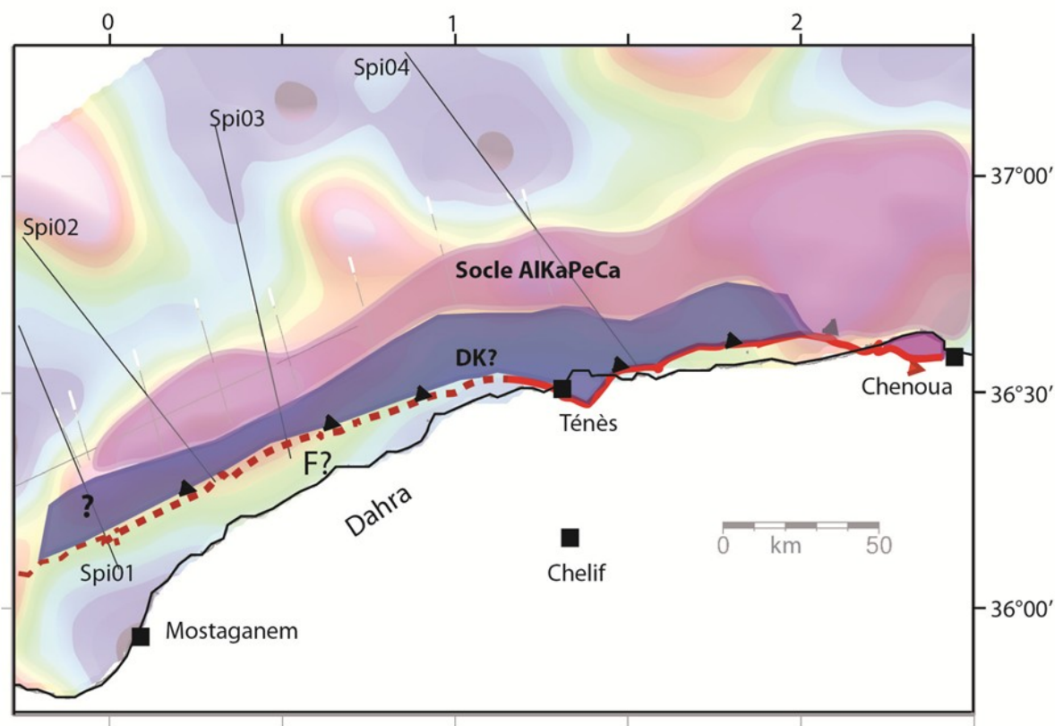
Figure V.7. Carte magnétique montrant le domaine AlKaPeCa dans le secteur de Mostaganem (le socle en mauve et la dorsale en bleu). La ligne rouge illustre la limite du domaine AlKaPeCa et zones externes, DK= dorsale kabyle, F=Flyschs.
