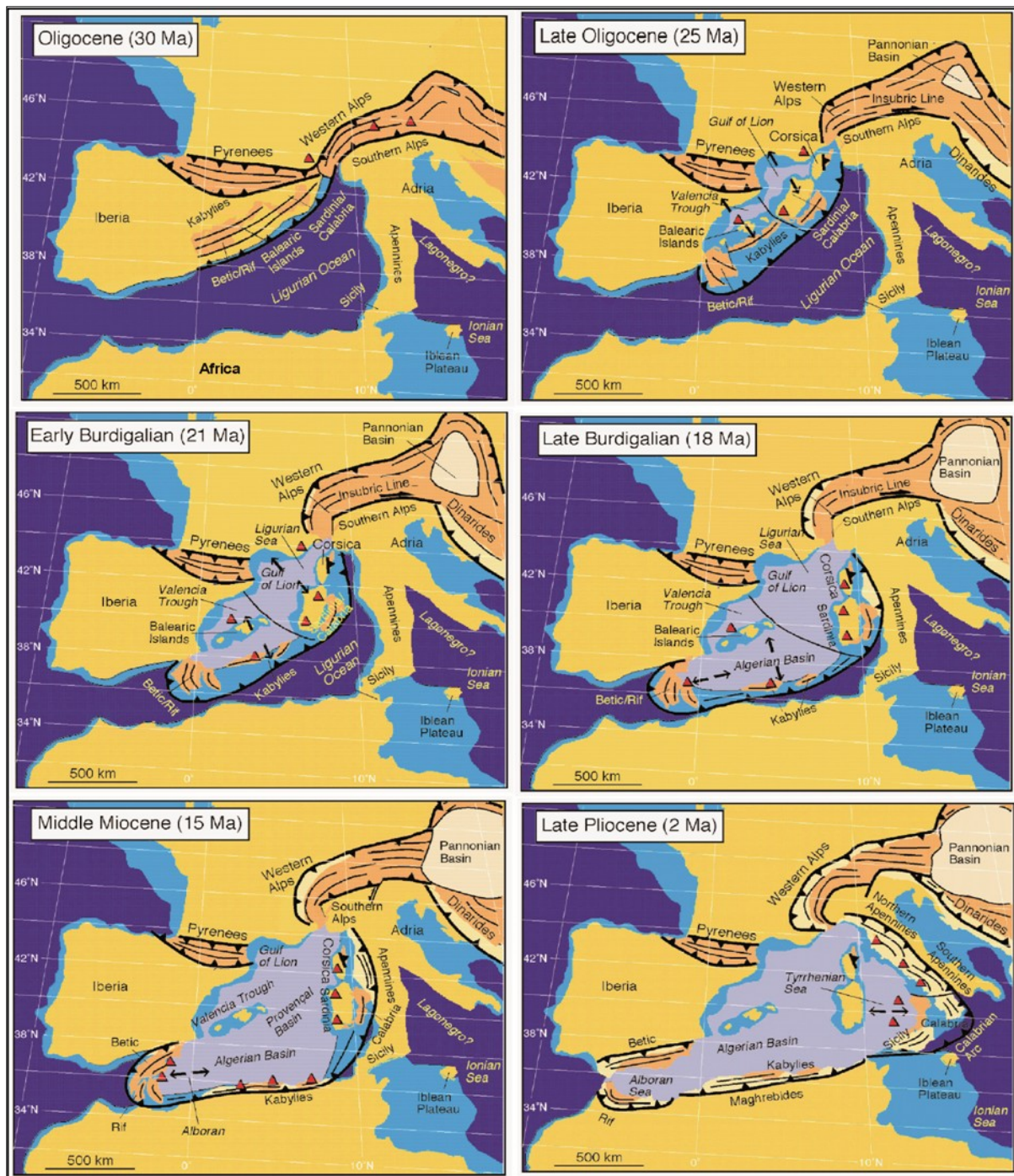
Figure I.10 : Reconstitution paléogéographique de la méditerranée occidentale depuis l'Oligocène, montrant la migration des subductions, l'ouverture des bassins arrière-arc et l'évolution spatiale du domaine ALKaPeCa (d'après Rosenbaum et al. 2002).
