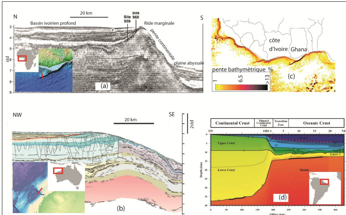
Figure 5. (a) exemples de caractéristiques des marges transformantes (a) coupe sismique sur la marge de Côte d'Ivoire-Ghana montrant une pente continentale raide et le développement d'une ride marginale (modifié d'après Basile et al., 1998), (b) coupe sismique sur la marge nord-ouest d'Australie montrant un analogue de ride marginale (modifié d'après TOTAL S.A.), (c) marge de Côte d'Ivoire Ghana montrant une pente bathymétrique abrupte et forte (modifié d'après Mercier de Lépinay 2012, communication personnelle), (d) modèle de vitesses sismiques V_p sur la marge de la Guyane-Est, montrant un amincissement crustal rapide avec une zone de transition étroite entre les croûtes continentale et océanique (modifié d'après Greenroyd et al., 2008).
