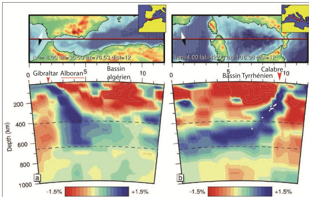
Figure I.11 – Images tomographies à travers (a) le détroit de Gibraltar, la mer d’Alboran et le bassin algérien et (b) le bassin Liguro-Provençal, la Corse, la bassin Tyrrhénien et la Calabre (d’après Spakman and Wortel, 2004).
