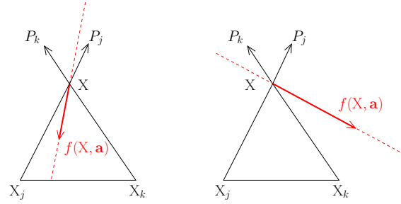
FIGURE 3.6 – Exemple d'un cas où le nœud X peut être évalué à partir des nœuds X_j et X_k (cas de gauche) et d'un cas où il doit être évalué à partir d'un autre triangle (cas de droite). La direction de la caractéristique f(X, \mathbf{a}) ne pointe pas à l'intérieur du triangle, le principe de causalité ne peut pas alors être vérifié.
