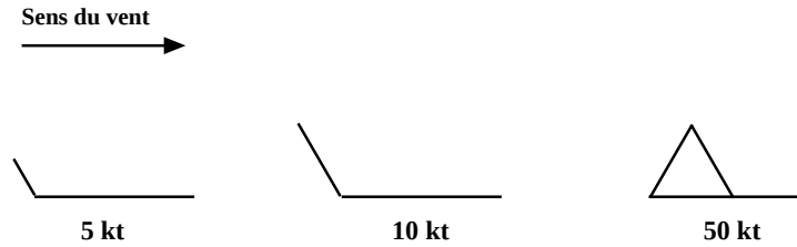
FIGURE 4.8 – Légende du vent : la hampe indique la direction d'où vient le vent. Les barbes indiquent la vitesse en nœud.
