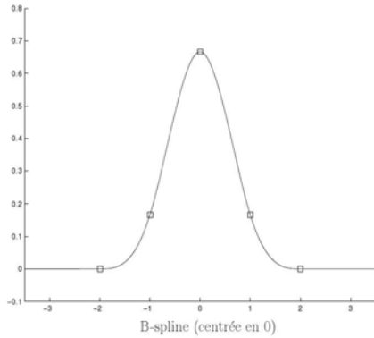
FIGURE 2.1 – Fonction de base B_0
