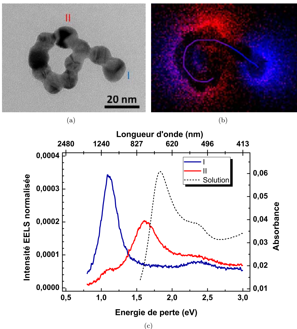
FIGURE V.11 – (a) Image TEM d'un motif de chaîne fusionné de 10 particules. (b) Superposition de deux images EELS SI enregistrées à 1.6 eV (pixels rouges) et à 1.1 eV (pixels bleus). (c) Spectres EELS mesurés en deux endroits différents du motif, identifiés par les chiffres romains sur la figure (a). Les spectres EELS sont normalisés de manière à ce que l'intensité du pic de perte nulle soit égale à 1. Ligne pointillée : rappel du spectre d'absorption des chaînes en solution de la FIGURE V.3.
