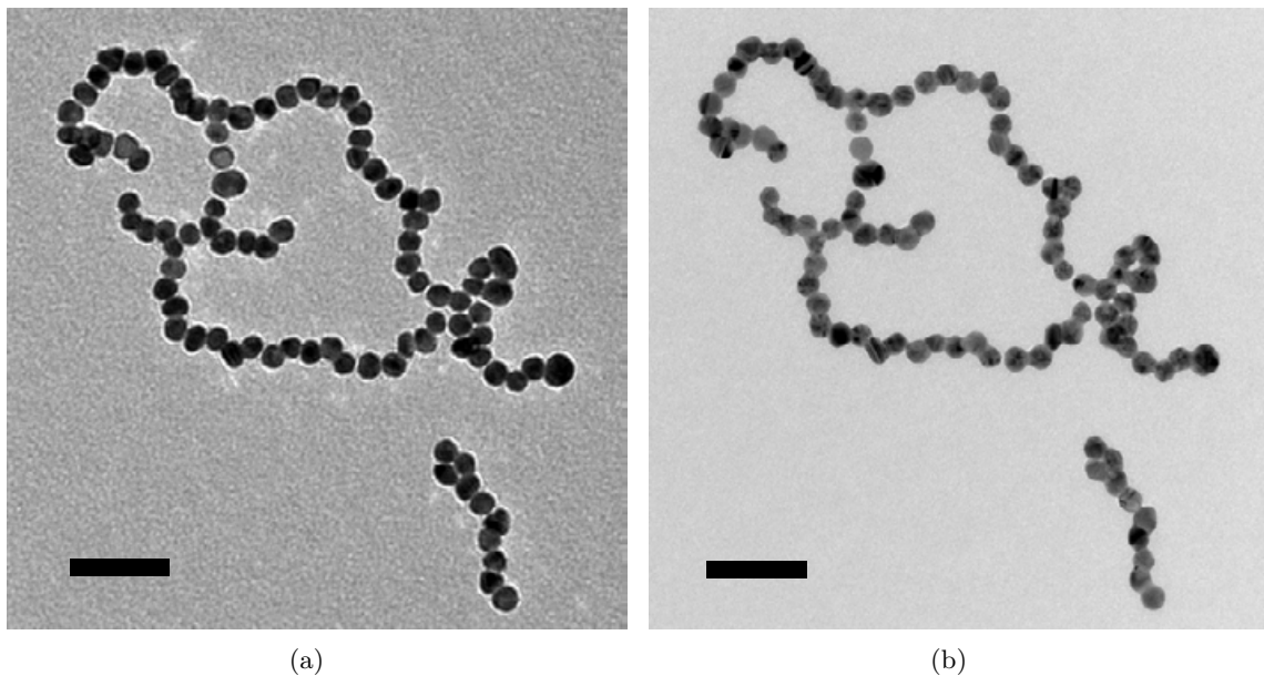
FIGURE V.10 – TEM d'un réseaux de nanoparticules auto-assemblées imagé dans un premier temps avec une tension d'accélération de 100 kV (a), puis de 200 kV (b). Barres d'échelle : 50 nm.
