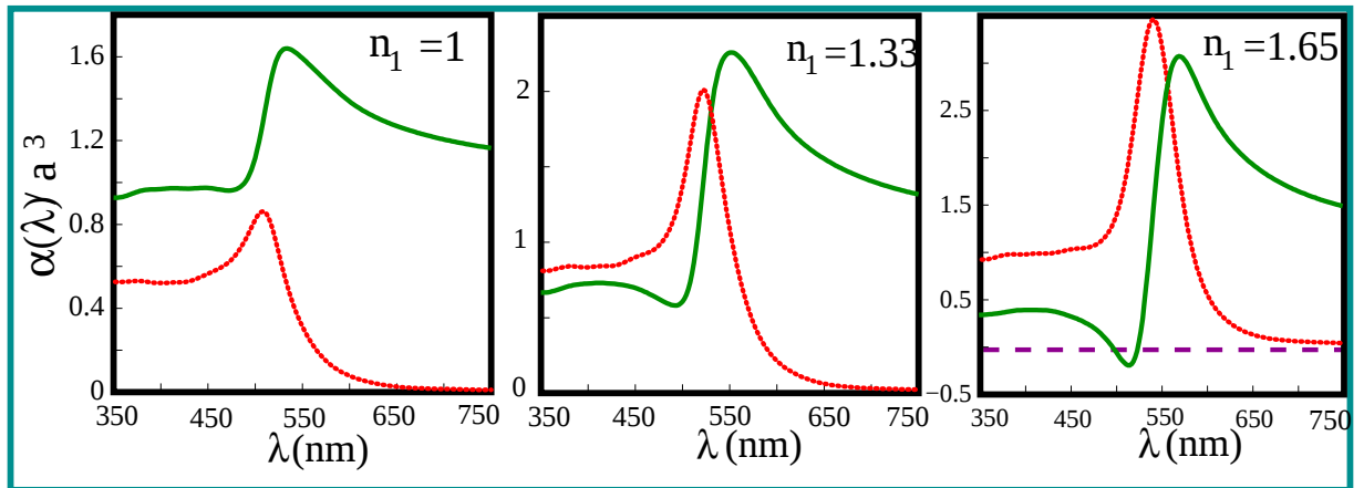
FIGURE II.5 – Polarisabilité dipolaire d'une sphère d'or isolée de volume unité, pour trois valeurs différentes de l'indice du milieu environnant. La partie réelle est en vert et la partie imaginaire en rouge. La ligne pointillée sur le troisième graphe indique où la partie réelle de la polarisabilité s'annule.
