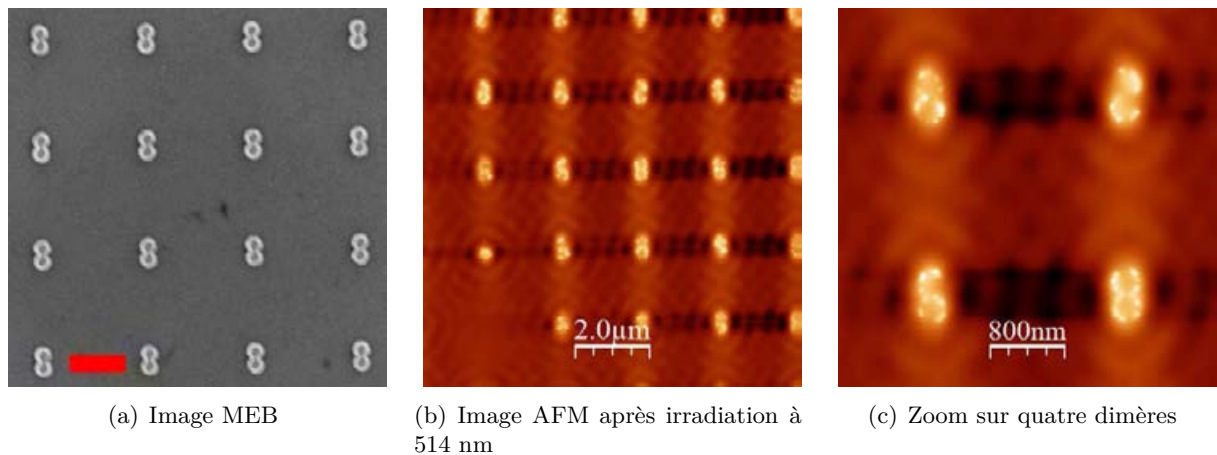
FIGURE II.14 – Dimères de disques lithographiés. La polarisation incidente est parallèle à l'axe des dimères. La barre d'échelle en (a) représente 1 \mu m .
