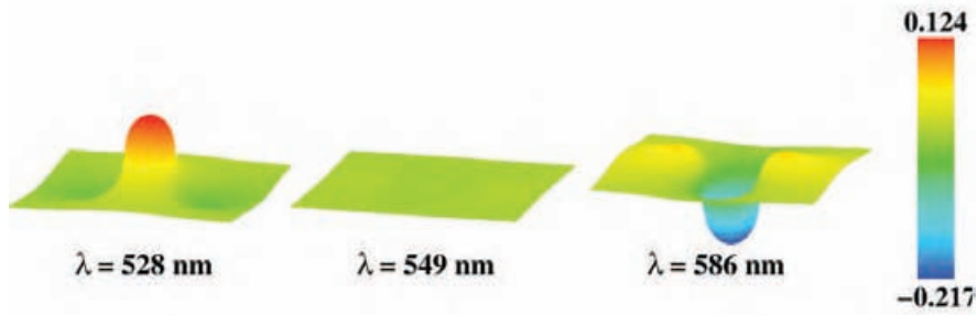
FIGURE II.8 – Carte du contraste optique au-dessus d'une sphère de 20 nm de diamètre pour 3 longueurs d'onde d'excitation.
