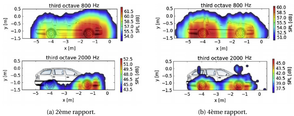
FIGURE 2.2 – Carte du niveau de bruit d'une voiture à essence passant à 50 km/h pour deux bandes de tiers d'octave différentes - De Ballestero et al. [17]
