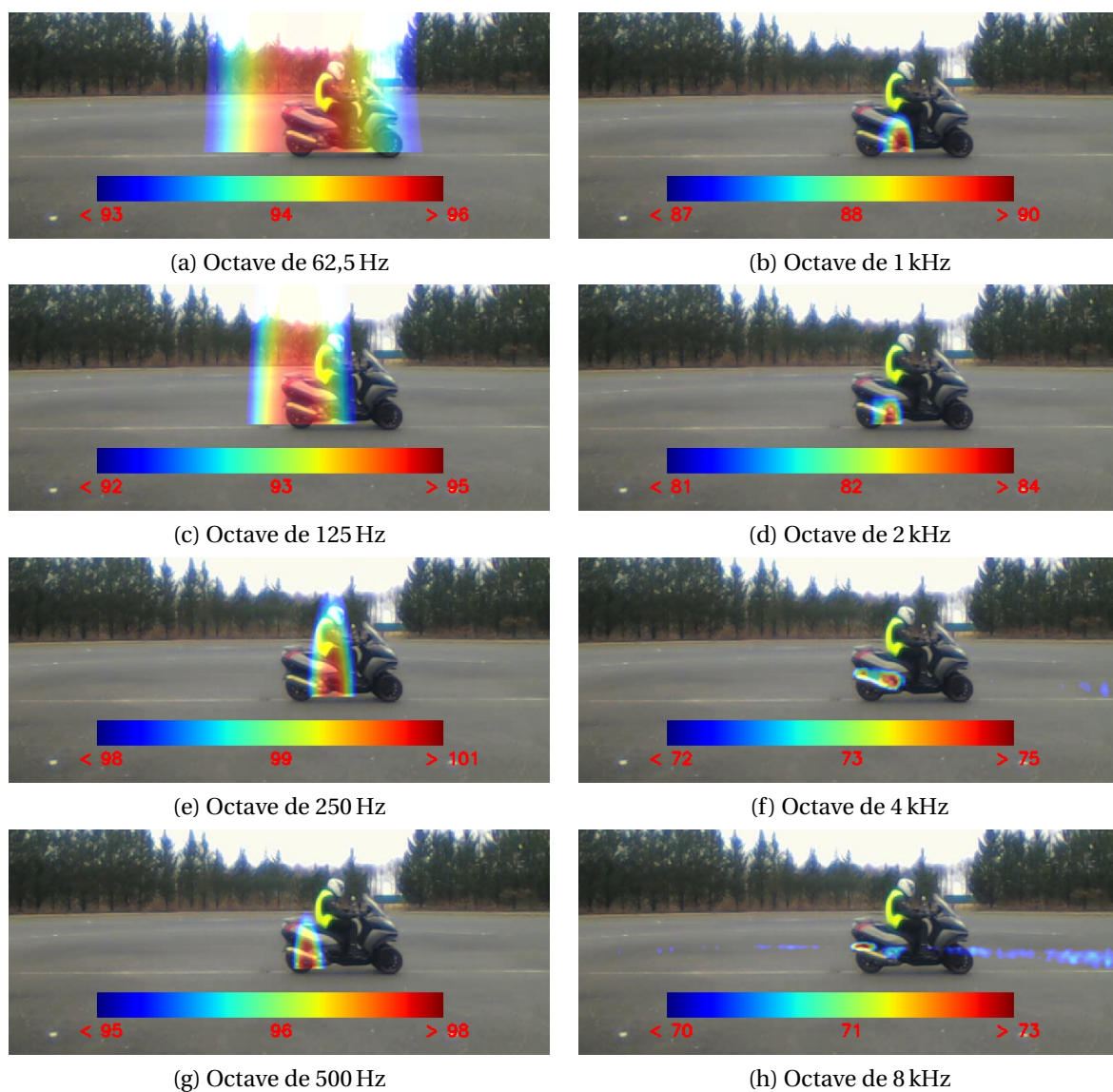
FIGURE 22 – Images acoustiques sur plusieurs bandes d'octaves du DR-Es-2 ( 400 \text{ cm}^3 ) – Accélération – Dynamique : 3 dB.
