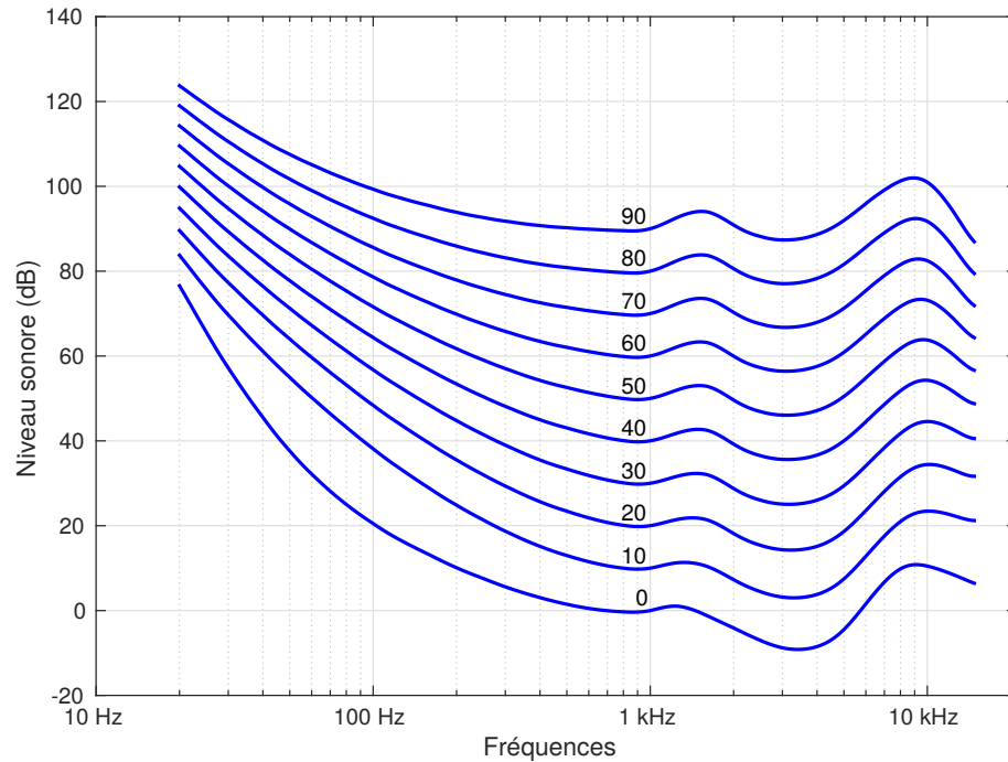
FIGURE 1.1 – Courbes d'isophonie de Fletcher - Niveau sonore perçu équivalent exprimé en phones en fonction du niveau acoustique et de la fréquence du son - ISO 226 [55].
