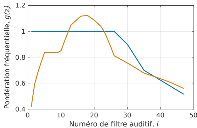
FIGURE 4.6 – Pondération fréquentielle g(z_i) en fonction du numéro de filtre auditif i utilisé dans le modèle de rugosité de García León (en orange) et de Osses Vecchi et al. (en bleu).
