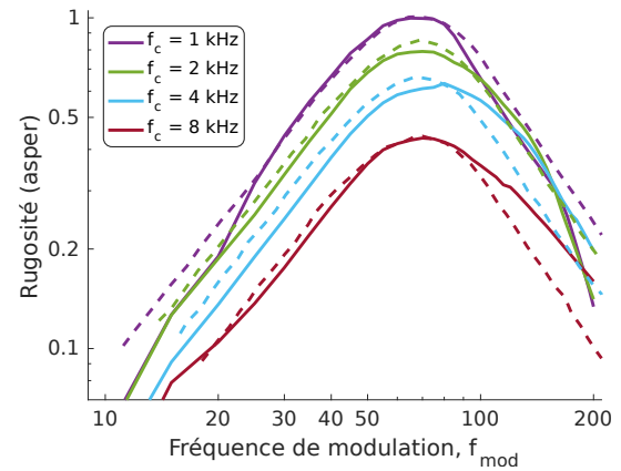
(b) Evolution de la rugosité en fonction de la fréquence de modulation et de la fréquence centrale du signal – De 1 à 8 kHz - m = 1 .
