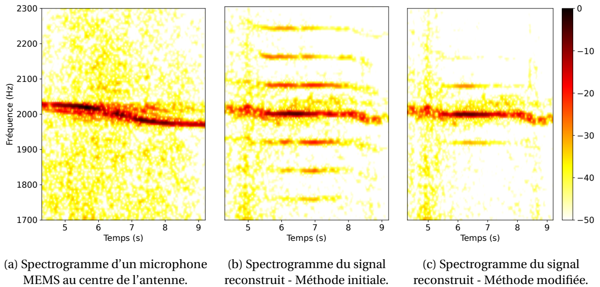
FIGURE 2.25 – Application de la méthode de reconstruction du signal à une source harmonique se déplaçant à vitesse constante ( V = 20 km/h) - Dynamique : 50 dB.
