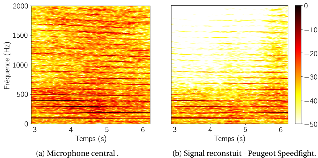
FIGURE 2.28 – Spectrogrammes des signaux du microphone central de l’antenne et ceux reconstitués du DR-Es-1 - Vitesse : 25 km/h.
