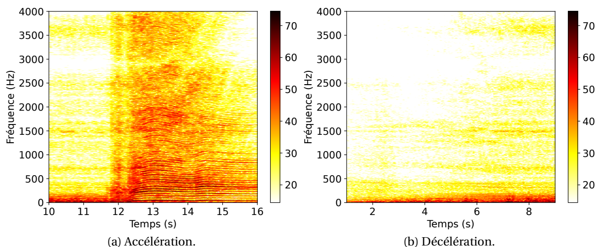
FIGURE 21 – Spectrogramme du microphone de référence lors du passage du DR-Es-2 ( 400 \text{ cm}^3 ) en accélération et décélération – Dynamique : 60 dB.
