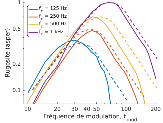
(a) Evolution de la rugosité en fonction de la fréquence de modulation et de la fréquence centrale du signal – De 125 Hz à 1 kHz - m = 1 .
