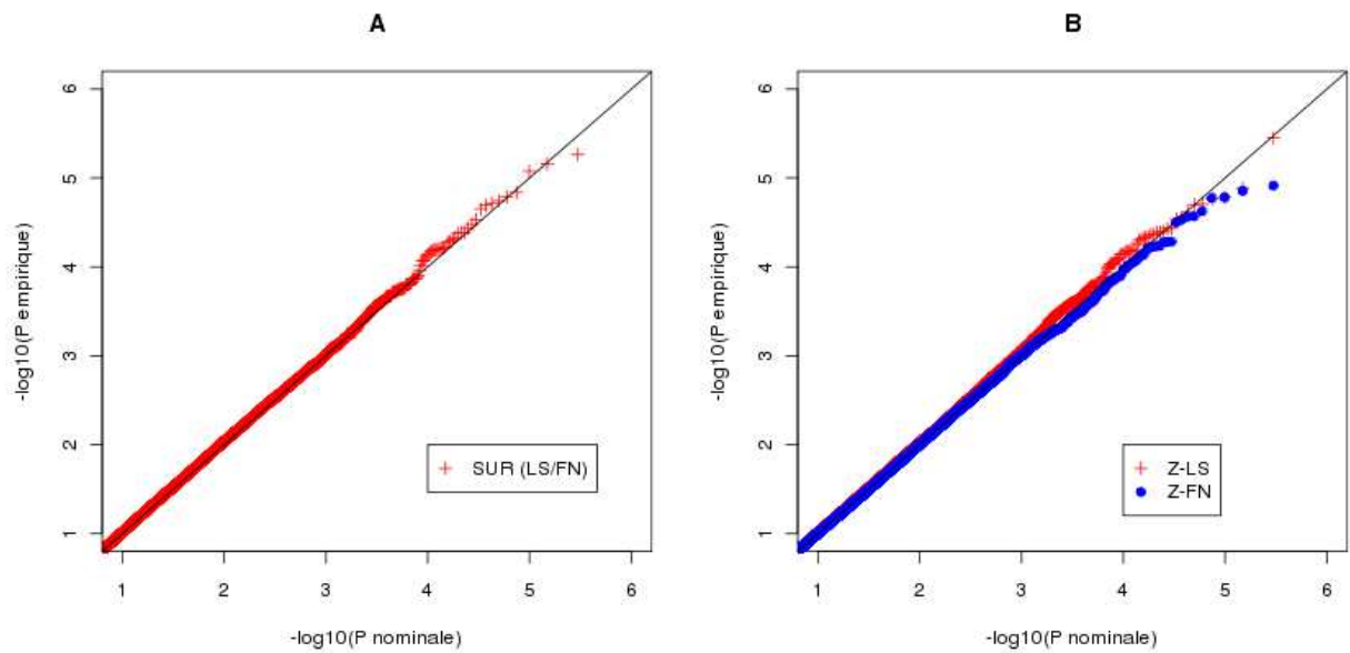
Figure 17 : Graphes quantiles contre quantiles des tests d'association bivariés basé sur le modèle SUR (A) et univariés de Z-LS et FN (B).
