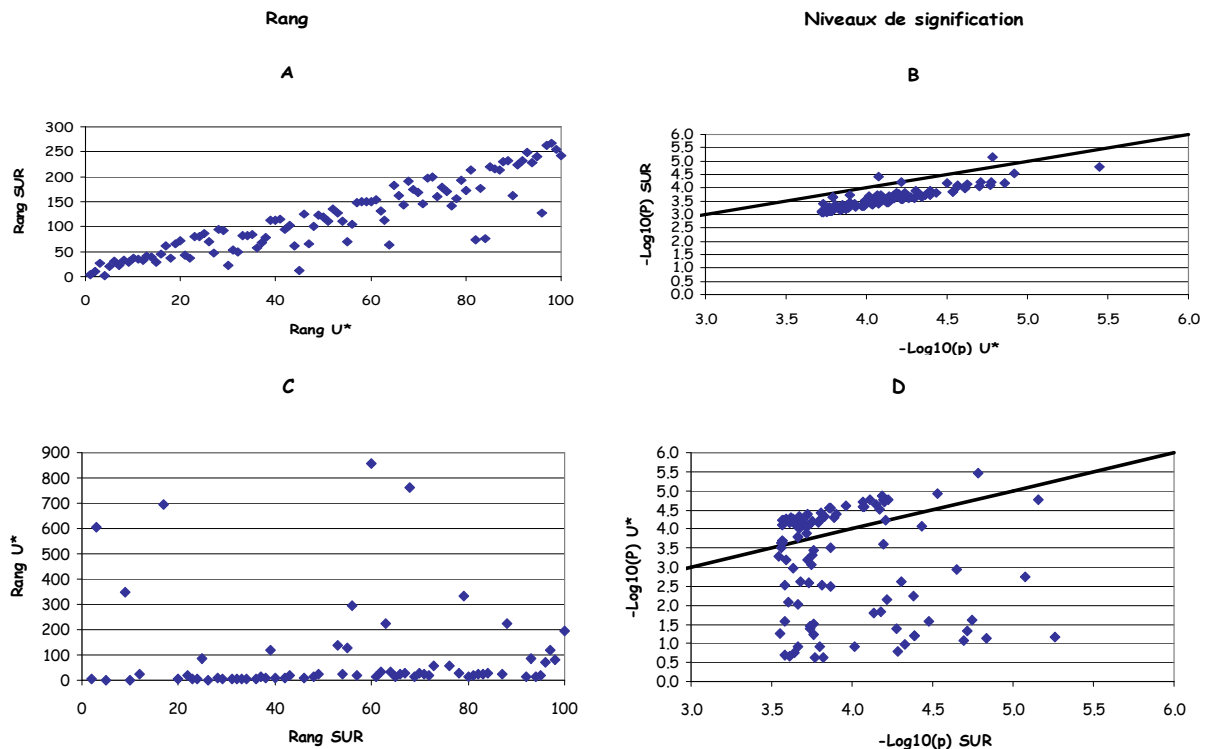
Figure 19 : Rangs et niveaux de signification des analyses univariées ( U^* ) et bivariées (SUR) pour les 100 SNPs les plus associés.
