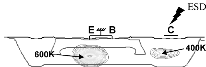
Figure 2-20. Localisation du maximum de température dans la Structure2 pour de fort courant I_{TLP}
