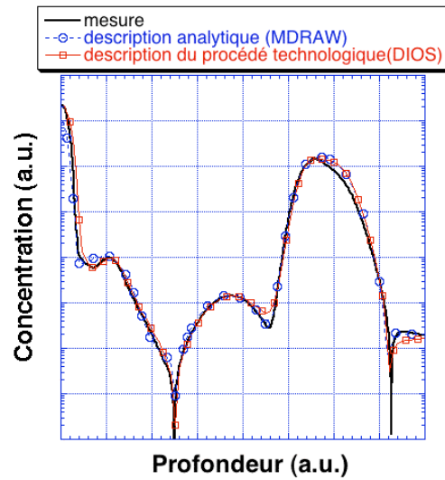
Figure 2-7. Profils de dopage suivant AA'
