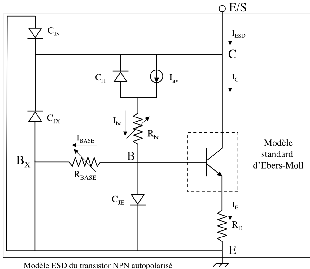
Figure 1-18. Schéma électrique du transistor bipolaire NPN autopolarisé
