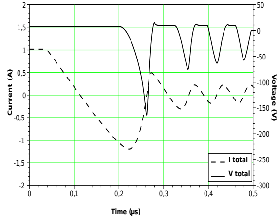
(b) Résultats de simulation du modèle VHDL-AMS de la diode PIN sous Questas-ADMS pour \tau=99 ns à T=400 K
