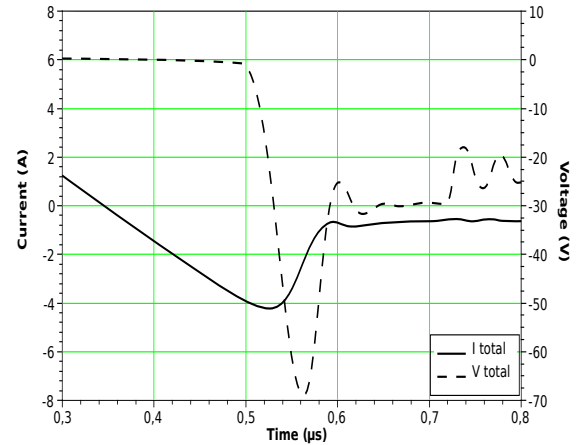
(b) Résultats de simulation du modèle VHDL-AMS de la diode PIN sous Questas-AMS à T=400 K
