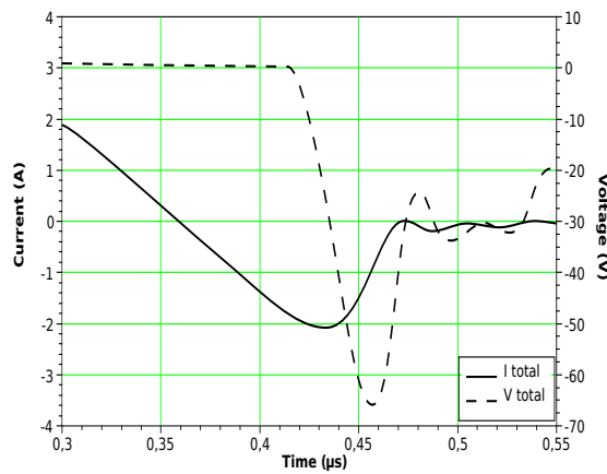
(a) Résultats de simulation du modèle VHDL-AMS de la diode PIN sous Questas-AMS pour à T=300 K
