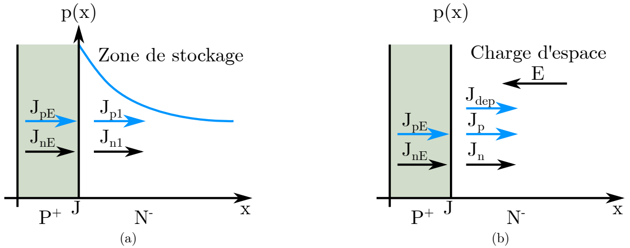
FIGURE 3.1 – (a) Continuité des courants et du produit pn à l'interface émetteur P + /zone de stockage des porteurs. (b) Continuité des courants à l'interface émetteur P + /zone de charge d'espace.
