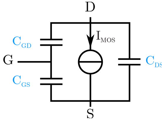
FIGURE 2.6 – Schéma équivalent de la section MOS.
