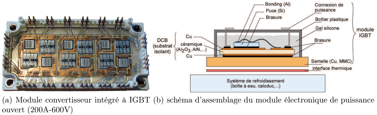
FIGURE 1.1 – Exemple de module IGBT utilisé dans la traction ferroviaire [Inrets 10].
