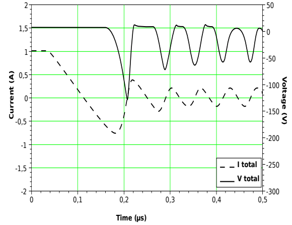
(b) Résultats de simulation du modèle VHDL-AMS de la diode PIN sous Questas-ADMS pour \tau=41 ns à T=400 K
