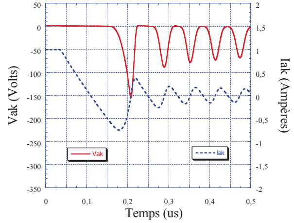
(d) Résultats de simulation du modèle MAST de la diode PIN sous SABER pour \tau=41 ns à T=400 K
