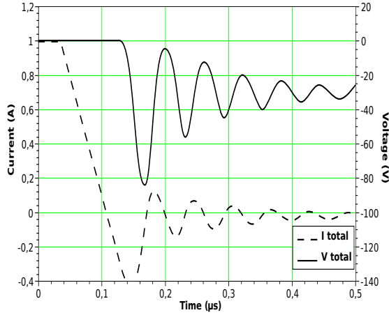
(a) Résultats de simulation du modèle VHDL-AMS de la diode PIN sous Questas-ADMS pour \tau=41 ns à T=300 K
