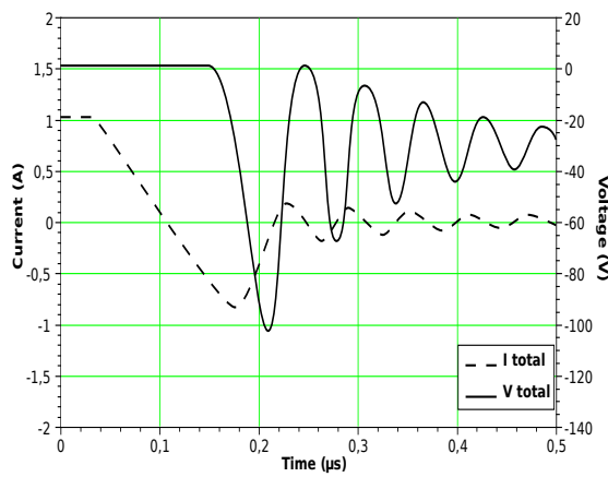
(a) Résultats de simulation du modèle VHDL-AMS de la diode PIN sous Questas-ADMS pour \tau=99 ns à T=300 K
