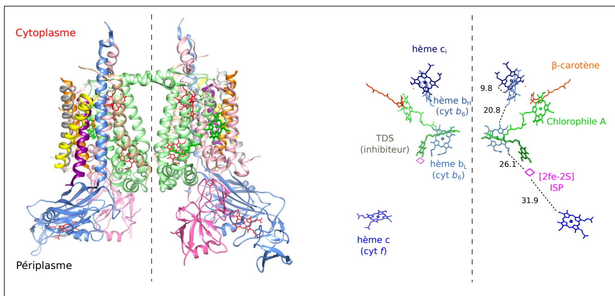
FIGURE I.10 – Structure et organisation des cofacteurs au sein du complexe cytochrome b 6 f . Gauche : Structure d'un dimère de cytochrome b 6 f en vue transversale à la membrane. Rieske : bleu ; SU IV : rose ; cyt b 6 : vert. Les hèmes sont représentés en rouge. Droite : Organisation des cofacteurs au sein du dimère. Les distances entre les centres métalliques (centres à centres) sont indiquées en Å. Modèle PDB : 1Q90.
