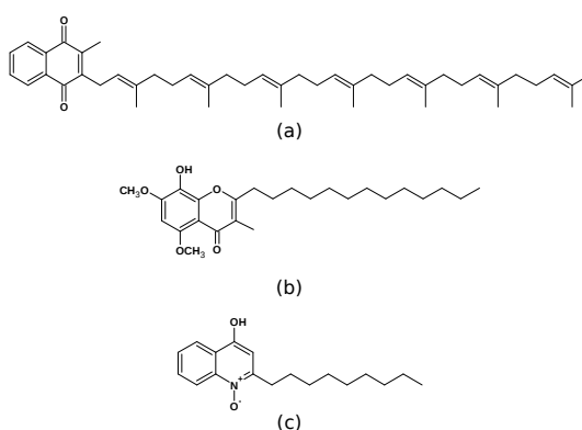
FIGURE III.29 – Quinones et analogues de quinones (a) Ménaquinone 7 (MK-7). (b) Tridécylstigmatelline (TDS), nom IUPAC : 8-Hydroxy-5,7-Dimethoxy-3-Méthyl-2-Tridécy-4H-Chromen-4-One. (c) NQNO (nonyl-4-hydroxyquinoline-N-oxide), nom IUPAC : 1-Hydroxy-2-Nonylquinolin-4-One.
