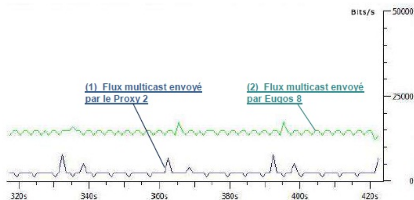
Figure 4.27: Courbes du trafic échangé entre un proxy DDS et un subscriber sur EuQoS8
