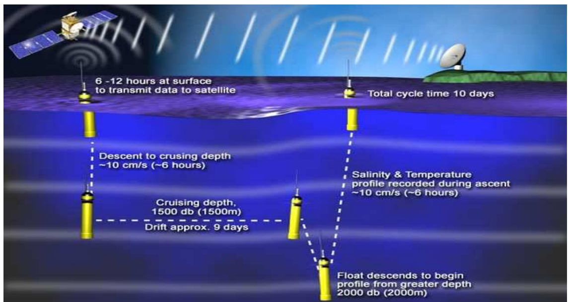
Figure 4.3 – Schéma montrant le cycle typique d'un flotteur ARGO.
