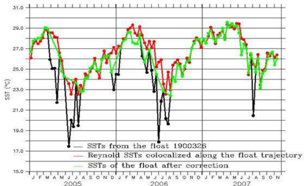
– Figure 4.4 : Comparaison le long de la trajectoire des SSTs pour le flotteur 1900326 avant élimination (en noir) et après (vert) avec les SSTs ((author?) [11]) (en rouge).
