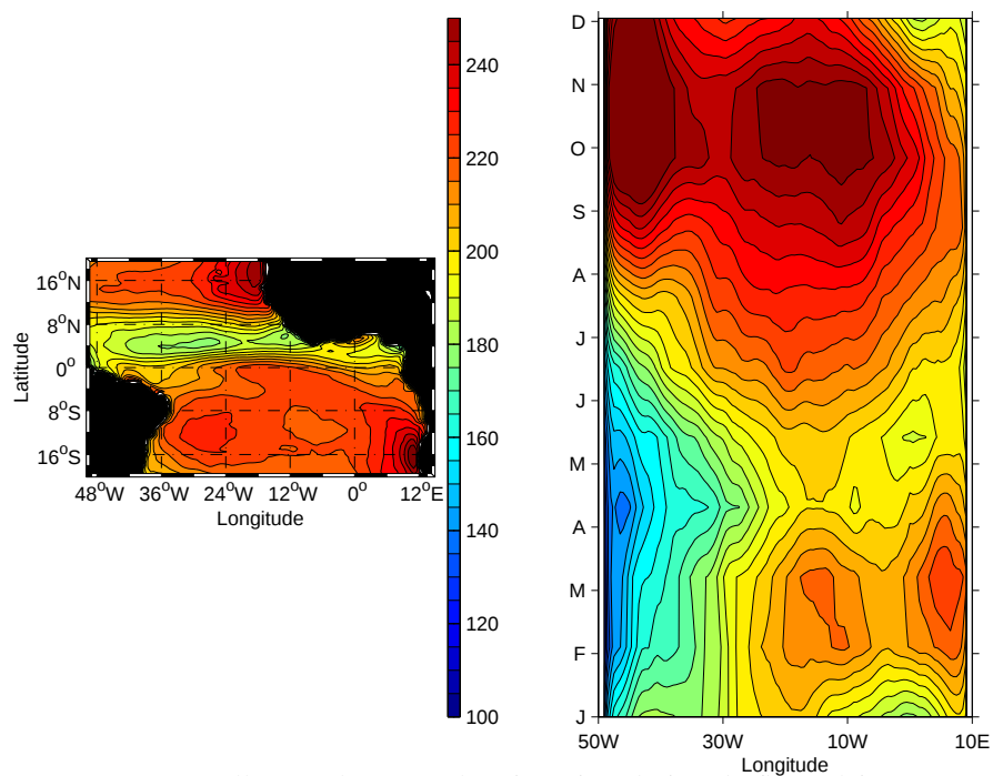
Figure 2.6 – Moyenne annuelle (gauche) et cycle saisonnier (droite) du flux solaire ( \text{W/m}^2 ) le long de l'équateur, source : ré-analyses du CEPMMT.
