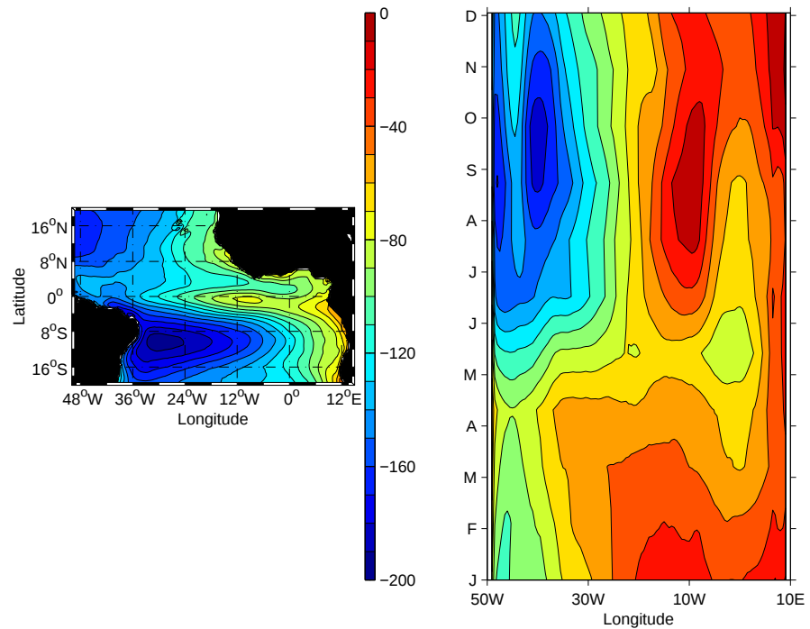
Figure 2.4 – Moyenne annuelle (gauche) et cycle saisonnier (droite) du flux latente ( \text{W/m}^2 ) le long de l'équateur, source : ré-analyses du CEPMMT.
