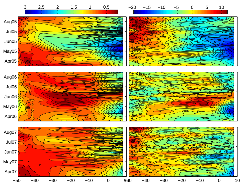
Figure 3.8 – Diagrammes Hovmöller des anomalies de température (°C) (panneau de gauche) et des anomalies la thermocline (m) (panneau de droite) des années 2005, 2006 et 2007 moyennées sur la bande 3°S-3°N.
