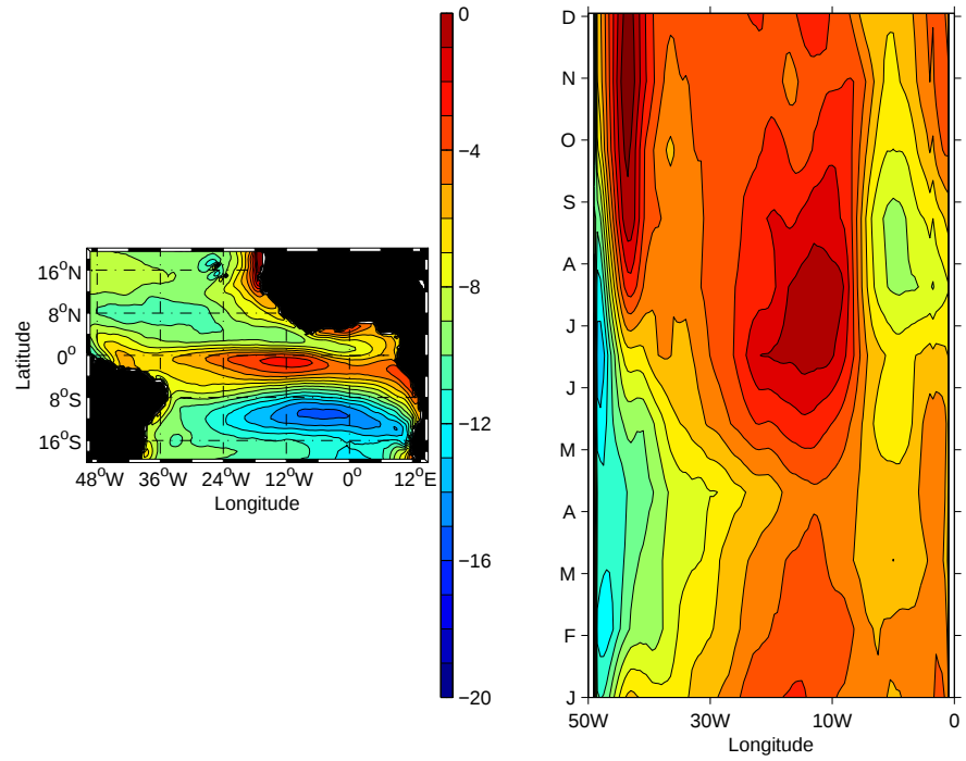
Figure 2.3 – Moyenne annuelle (gauche) et cycle saisonnier (droite) du flux sensible ( \text{W/m}^2 ) le long de l'équateur, source : ré-analyses du CEPMMT.
