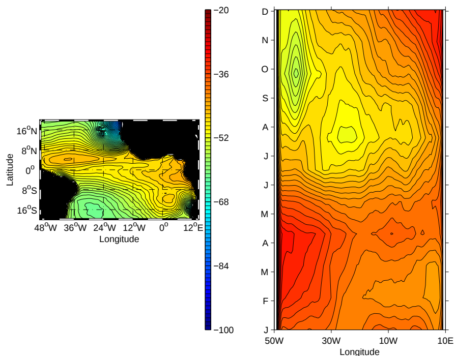
Figure 2.5 – Moyenne annuelle (gauche) et cycle saisonnier (droite) du flux infra-rouge ( \text{W/m}^2 ) le long de l'équateur, source : ré-analyses du CEPMMT.
