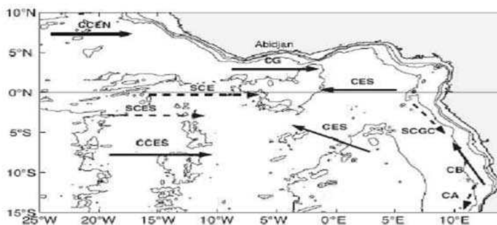
– Figure 2.12 : Schéma de circulation superficielle et sub-superficielle dans l'Atlantique équatorial et le Golfe de Guinée. Courants de surface (flèches avec traits pleins) : Contre Courant Equatorial Nord (CCEN) ; Courant de Guinée (CG) ; Contre Courant Equatorial Sud (CCES) ; Courant Equatorial Sud (CES) ; Courant du Benguela (CB). Courants de sub-surface (flèches avec traits tiretés) : Sous Courant Equatorial Nord (CSEN) ; Sous Courant Equatorial (SCE) ; Sous Courant Equatorial Sud (SCES) ; Sous Courant du Gabon-Congo (SCGC) ; Courant d'Angola (CA) ; Bourlès et Caniaux, 2004 1 .
