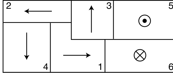
Figure 2.2 – Configuration magnétique schématisée dans une situation quelconque, en l'absence de rotations
