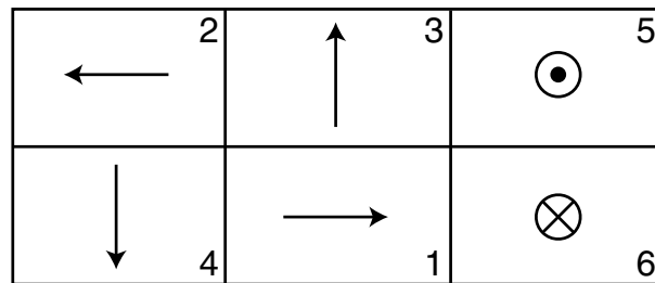
Figure 2.3 – Configuration magnétique (schématisée) de référence à l'état désaimanté
