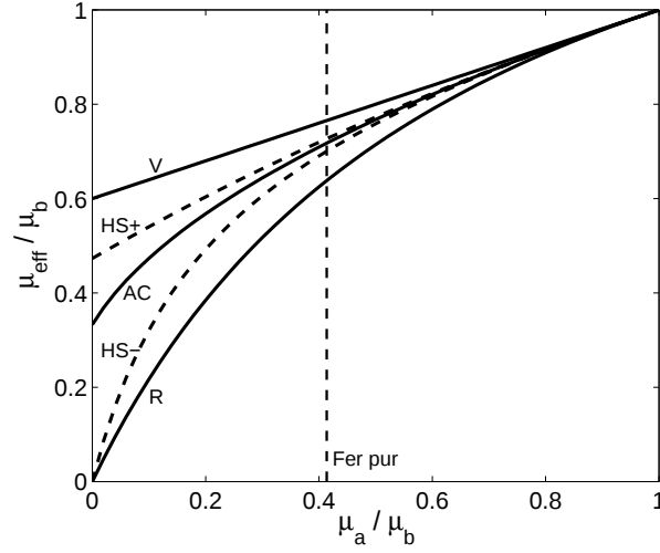
Figure B.1 – Différentes estimations du comportement effectif en fonction de l'anisotropie du monocristal - Estimations de Voigt (V) et Reuss (R), de Hashin et Shtrikman (HS+ et HS-) et autocohérente (AC)
