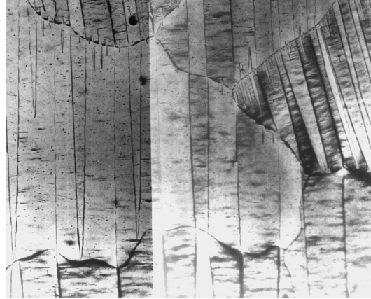
Figure 5.5 – Observation de domaines magnétiques à la surface d'une tôle GO, d'après [Hug, 1995]
