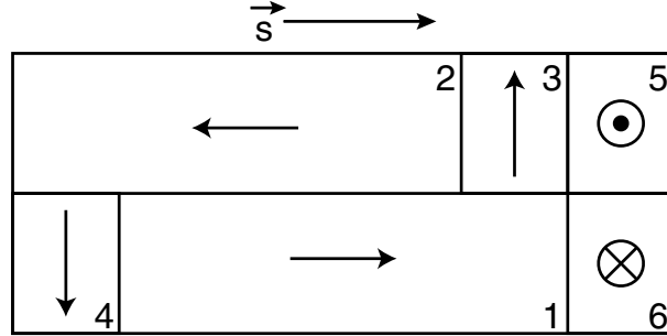
Figure 2.5 – Configuration magnétique (schématique) pour une contrainte de traction uniaxiale dans la direction \vec{s}
