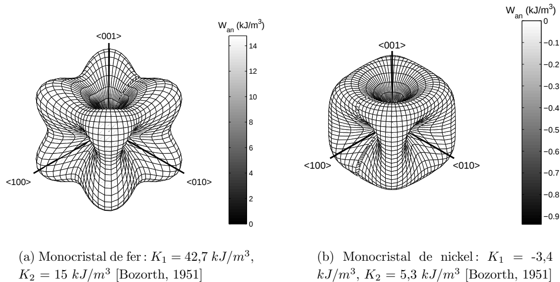
Figure 1.4 – Représentation spatiale de l'énergie d'anisotropie magnétocristalline
