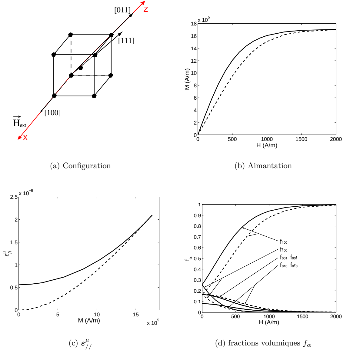
Figure 4.7 – Résultats pour la configuration 3 - Calculs avec (lignes) et sans (pointillés) prise en compte de l'effet de surface
