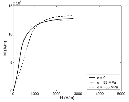
(b) Résultats expérimentaux [Kuruzar et Cullity, 1971]
