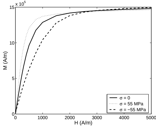
(a) Résultats numériques
