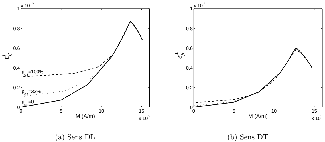
Figure 4.12 – Courbes de magnétostriction du polycristal de fer à 3% de silicium - influence de la proportion de grains de surface - résultats pour 33 et 100% - N_s = 1000 \text{ J/m}^3
