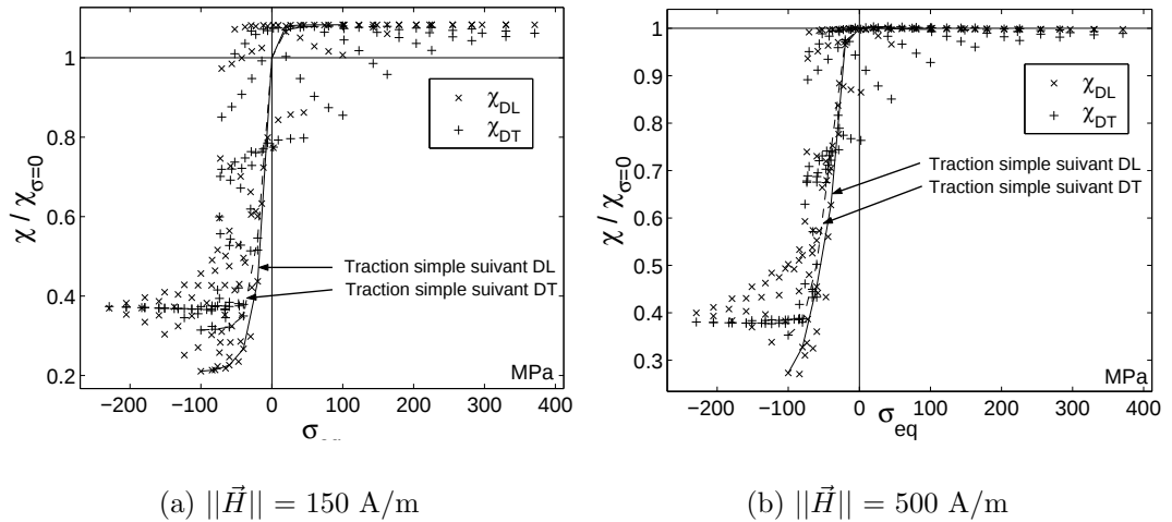
Figure 5.23 – Susceptibilités magnétiques relatives en fonction de la contrainte équivalente - Fe-3%Si NO - Résultats de calcul
