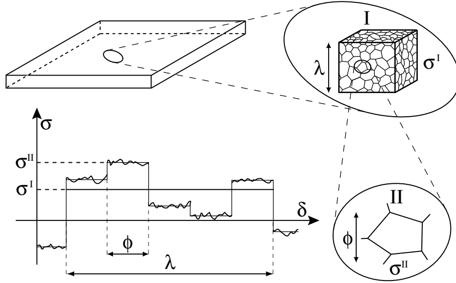
Figure 4.19 – Définition schématique des contraintes résiduelles d'ordre 1 ( \sigma^I ) et d'ordre 2 ( \sigma^{II} ) dans un matériau polycristallin - \lambda désigne la longueur caractéristique du VER et \phi la taille moyenne des grains
