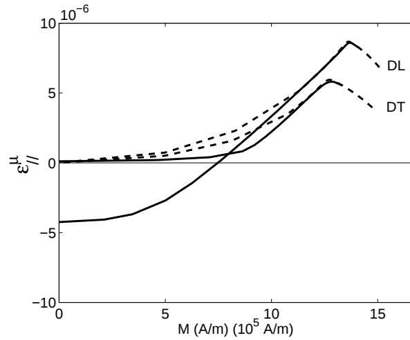
Figure 5.26 – Influence d'un état de contraintes résiduelles d'origine plastique ( \varepsilon_{11}^p \simeq 1,2 \cdot 10^{-4} ) sur la déformation de magnétostriction anhystérétique (lignes) et comparaison avec un état libre de contraintes résiduelles (pointillés) - Directions DL et DT - Résultats de calcul - Fe-3% Si NO
