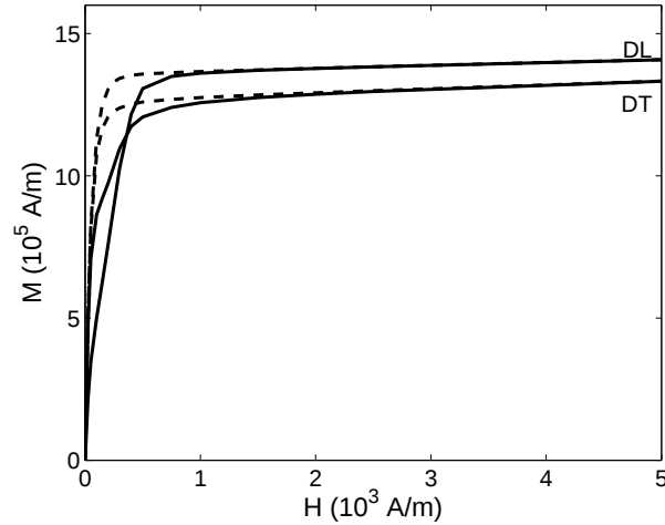
Figure 5.25 – Influence d'un état de contraintes résiduelles d'origine plastique ( E_{11}^p \simeq 1,2 \cdot 10^{-4} ) sur la courbe d'aimantation anhystérique (lignes) et comparaison avec un état libre de contraintes résiduelles (pointillés) - Directions DL et DT - Résultats de calcul - Fe-3% Si NO
