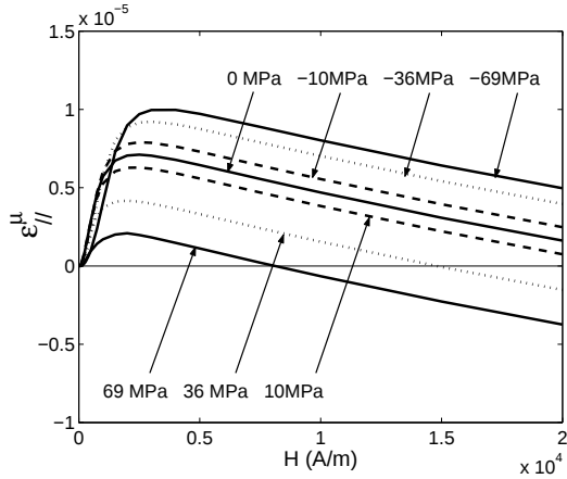
(a) Résultats numériques
