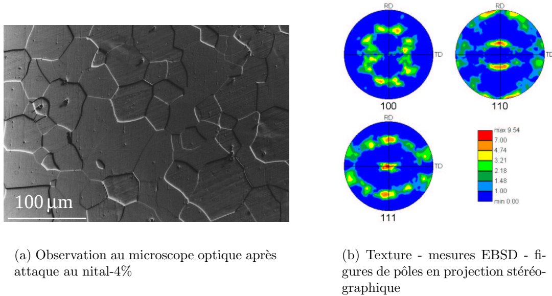
Figure 3.12 – Caractérisation du Fe-3%Si NO
