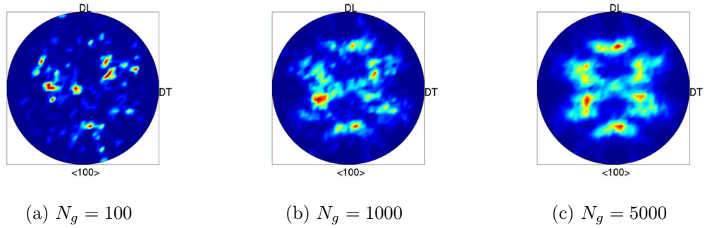
Figure C.15 – Figures de pôles \langle 100 \rangle pour le M330 - Influence de la taille de la FDO
