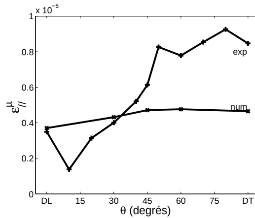
Figure 4.14 – Anisotropie magnétostrictive dans le plan de tôle - comparaison des résultats expérimentaux et numériques avec prise en compte d'un effet de surface - \|\vec{M}_m\| = 1,2 \cdot 10^6 \text{ A/m} - Fe-3%Si NO
