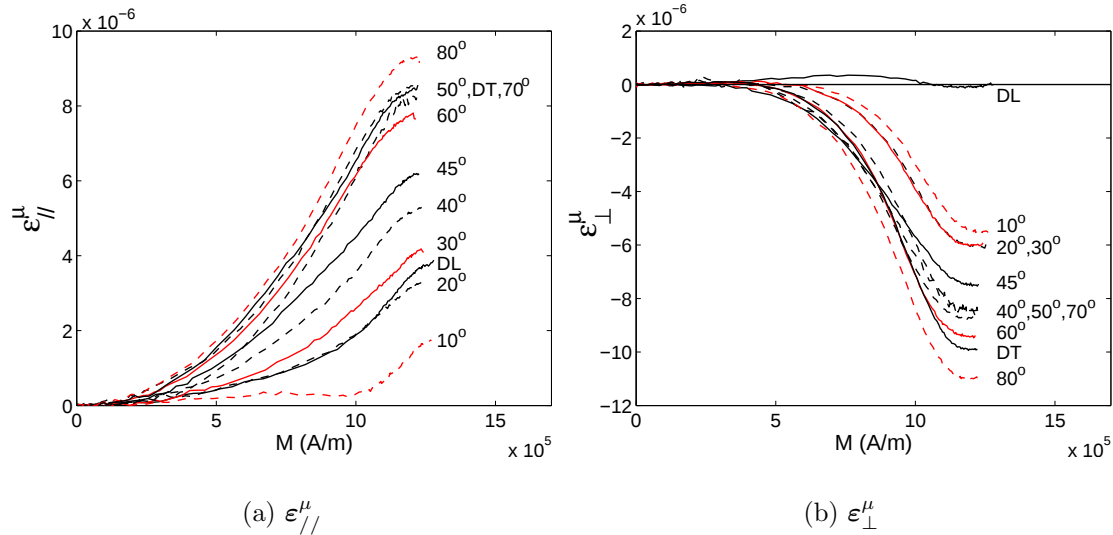
Figure 3.22 – Mesure de la déformation de magnétostriction pour un champ magnétique appliqué suivant différentes directions du plan de tôle - FeSi 3% NO - [Hubert et al., 2002]
