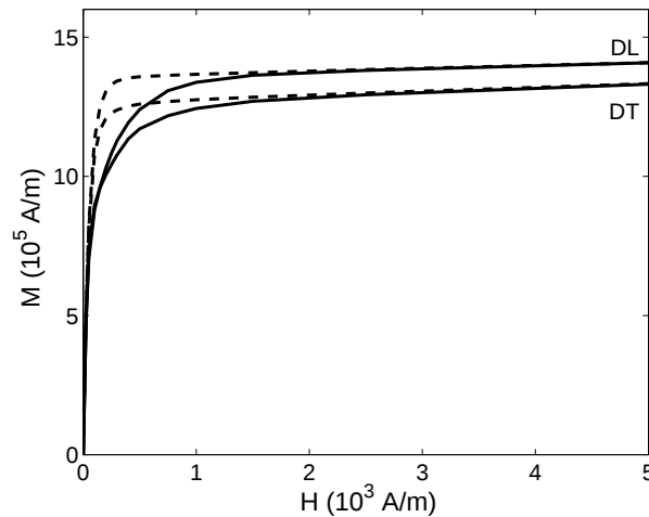
Figure 4.21 – Influence d'un état de contraintes résiduelles (figure 4.20) sur la courbe d'aimantation anhystérétique (lignes) et comparaison avec un état libre de contraintes résiduelles (pointillés) - Directions DL et DT - Résultats de calcul - Fe-3% Si NO
