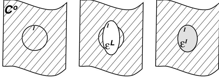
Figure 2.9 – Problème d'Eshelby
