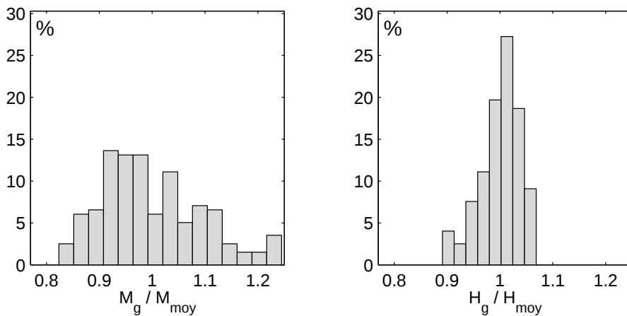
Figure 4.3 – Distribution par grains de la norme de l'aimantation et du champ magnétique dans le matériau - \|\vec{H}_{\text{ext}}\| = 150 A/m - Résultats de calcul avec prise en compte du champ démagnétisant
