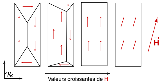
Figure 1.5 – Principe du processus d'aimantation dans un monocristal
