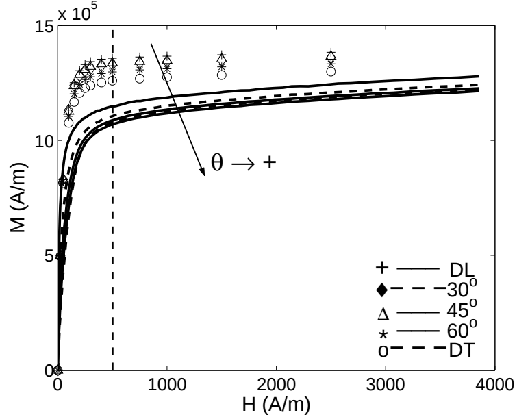
Figure 3.31 – Courbes d'aimantation anhystérétique - comparaison des résultats expérimentaux (lignes) et numériques (points) - Fe-3%Si NO
