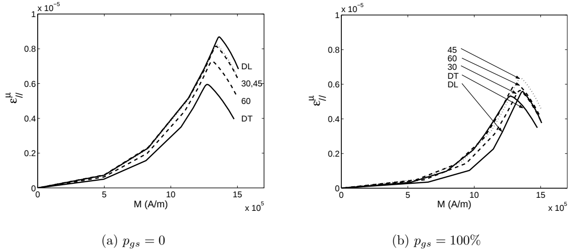
Figure 4.13 – Courbes de magnétostriction du polycristal de fer à 3% de silicium - N_s = 1000 \text{ J/m}^3
