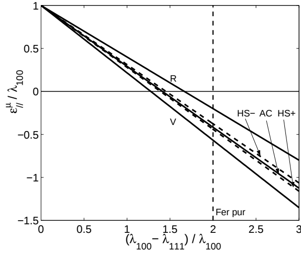
Figure B.3 – Différentes estimations pour la déformation de magnétostriction à saturation en fonction de l'anisotropie magnétostrictive du monocristal - Estimations de Voigt (V) et Reuss (R), de Hashin et Shtrikman (HS+ et HS-) et autocohérente (AC)
