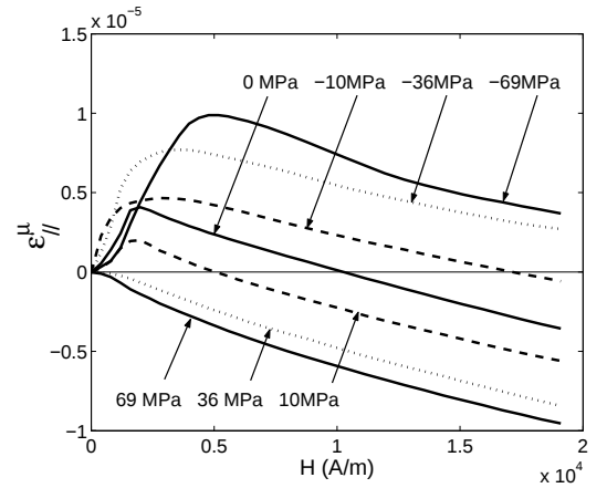
(b) Résultats expérimentaux [Kuruzar et Cullity, 1971]
