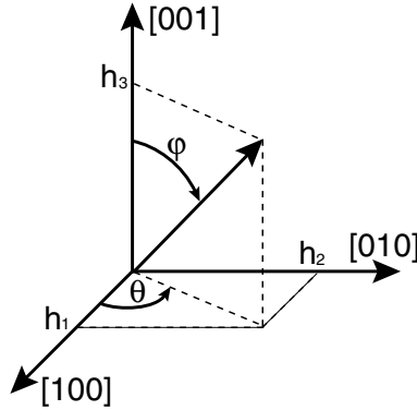
Figure 3.8 – Coordonnées du champ magnétique \vec{H}^{\mathbf{I}} dans le repère du monocristal
