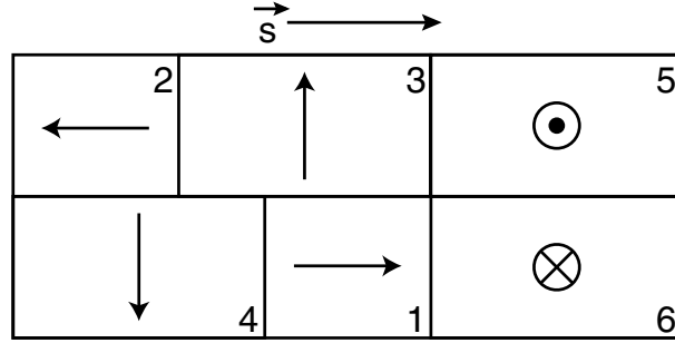
Figure 2.6 – Configuration magnétique (schématique) pour une contrainte de compression uniaxiale dans la direction \vec{s}
