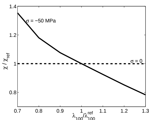
Figure C.8 – Influence d’une variation du coefficient magnétostrictif \lambda_{100} du monocristal sur la prévision de la susceptibilité (sécante) sous contrainte uniaxiale du polycristal à 500 A/m - sens DL - Fe3%Si NO
