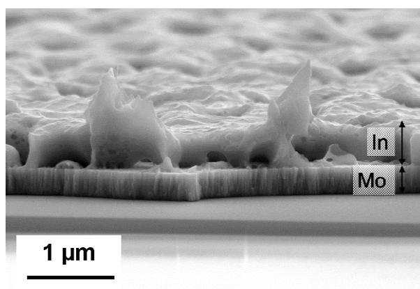
Figure 3.2.11. Microscopie en coupe (MEB) d'In électrodéposé sur substrat Mo à -1,6 V/MSE pendant 30 min à partir d'une solution de 0.13 M de sulfate de sodium (pH 2,15) avec 0,9 mM de \text{In}_2(\text{SO}_4)_3 .
