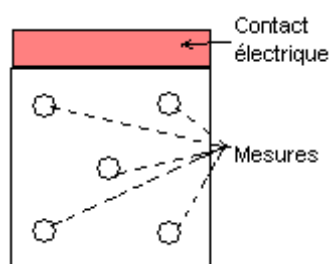
Figure B.4. Position des points de mesures pour l'analyse par fluorescence X sur substrat 2,5 \times 2,5 \text{ cm}^2 et position du contact électrique.
