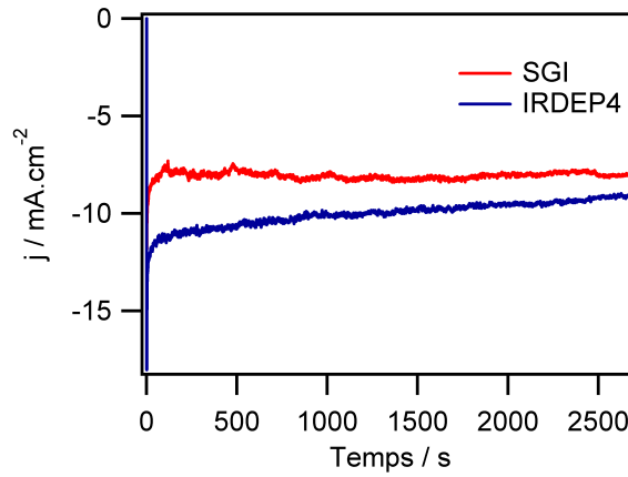
Figure 3.4.13. Transitoires de courant lors de l'électrodepôt de Cu-In-Ga à -1,5 V pendant 45 min sur substrats Mo_SGI et IRDEP.
