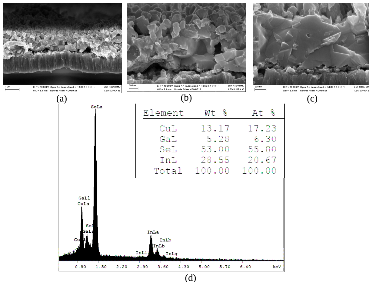
Figure 4.2.19. (a)(b)(c) Micrographies en coupe d'un précurseur Cu-In-Ga (SP8) sélénié par suite d'un dépôt en bain chimique et d'un recuit rapide à 620°C et (d) résultats de l'analyse EDS correspondant à l'image (c).
