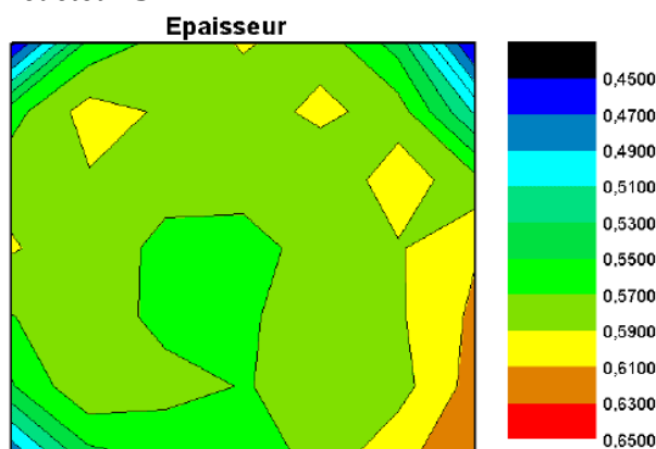
Figure B.10. Cartographie d'épaisseur en microns. Electrodeposition 45 min à -1,6 \text{ V/MSE} , avec agitation peigne. L'épaisseur moyenne est 0,57 \mu\text{m} avec un écart-type de 0,04 et un coefficient de variation de 6,7\%
