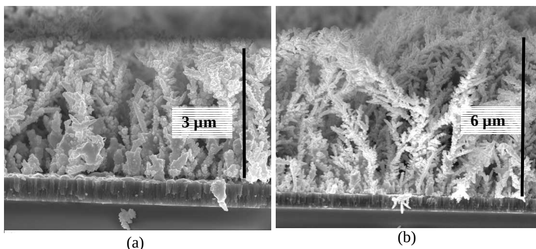
Figure 3.4.3. Micrographies MEB en coupe du précurseur électrodéposé avec un électrolyte support sulfate El-1 (a), et un électrolyte chlorure El-2 (b) pour une même composition de dépôt.
