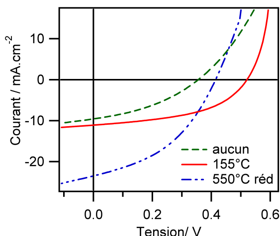
Figure 5.1. Caractéristiques courant-tension des cellules solaires formées à partir de précurseurs Cu-In-Ga ayant subi trois recuits intermédiaires différents, avec une même composition ( \text{Ga}/(\text{In}+\text{Ga}) = 0,42 ) et une même sélénisation rapide à 600^\circ\text{C} .
