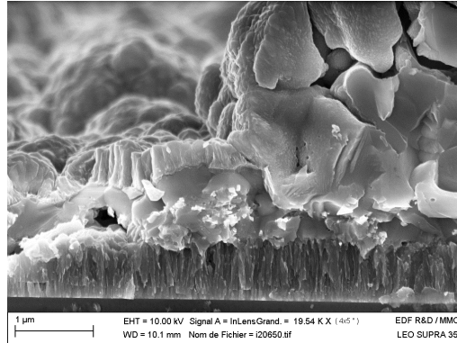
Figure 4.2.18. Micrographie d'un précurseur Cu-In-Ga avec dépôt en bain chimique de Se et recuit « standard » à 450°C pendant 50 min (échantillon SP7).
