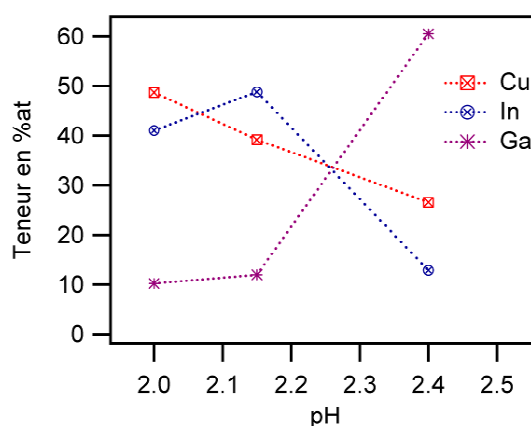
Figure 3.4.12. Evolution de la composition en fonction du pH (El-3 avec 0,8 mM de \text{In}_2(\text{SO}_4)_3 , à -1,6 \text{ V/MSE} , avec agitation peigne, 220 \text{ min}^{-1} ). Le tracé entre les points est juste précisé pour guider les yeux.
