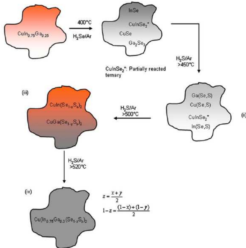
Figure 1.22. Représentation schématique des réactions à l'état solide conduisant à la formation de chalcopyrites homogènes \text{Cu}(\text{In,Ga})(\text{S,Se})_2 [146]. Pour des raisons de clarté, le chemin réactionnel est divisé en 4 étapes.
