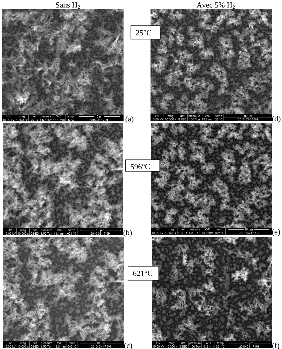
Figure 4.1.4. Micrographies en surface d'un précurseur Cu-In-Ga (a) (d) tel qu'électrodéposé à 25°C ; (b) (e) recuit à 595°C ; (c) (f) recuit à 621°C ; (a)(b)(c) sous atmosphère inerte \text{N}_2 ; (d)(e)(f) sous atmosphère réductrice \text{N}_2 + 5\%\text{H}_2 .
