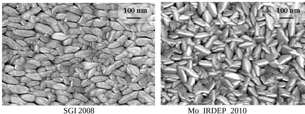
Figure 2.1. Micrographie de la surface des substrats Mo/verre SGI 2008 et Mo_IRDEP_2010.
