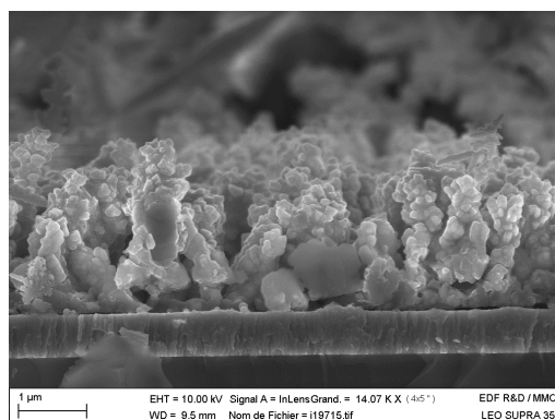
Figure 3.3.12. Morphologie d'un dépôt avec un rapport Cu/Ga=1 : électrodepôt réalisé à -1,4 V/MSE, avec un électrolyte contenant 2 mM Cu(II), 8 mM Ga(III), 0,4 M NaCl; à pH 2,2, sans citrate.
