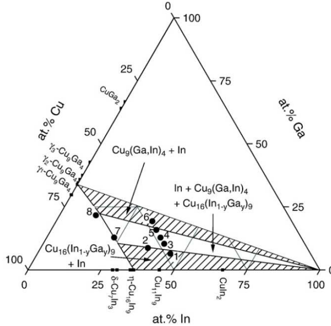
Figure 4.1.2. Diagramme de phases du système Cu-In-Ga : projection à température ambiante des relations de phase évaluées à 350°C, d'après Purwins et al. [4]
