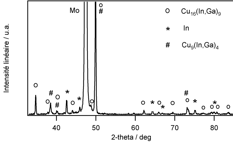
Figure 4.1.14. Diffractogramme d'un précurseur après recuit intermédiaire à 550°C pendant 6 min (anode en cobalt, \lambda_{\text{K}\alpha 1} = 0,1789 \text{ nm} ). La composition de l'échantillon est : \text{Cu}/(\text{In}+\text{Ga}) = 0,87 et \text{Ga}/(\text{In}+\text{Ga}) = 0,19 .
