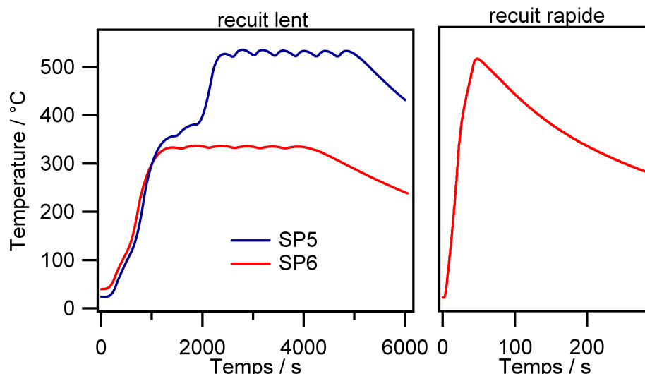
Figure 4.2.15. Profils de température pour la sélénisation des précurseurs Cu-In-Ga : Echantillon SP5 : 2 paliers : 340-380°C 13 min puis 530°C 50 min. Echantillon SP6 : 2 recuits : 1 ère sélénisation dans le four tubulaire à 335°C (24 mg Se pour 5 x 5 cm 2 ), 2 e sélénisation dans le four à recuit rapide à environ 530°C (8 mg Se pour 2,5 x 2,5 cm 2 )
