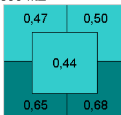
Figure B.9. Cartographie d'épaisseur d'un échantillon (en microns). Electrodeposition 45 min à -1,6 \text{ V/MSE} , avec agitation peigne. L'épaisseur moyenne est 0,55 \mu\text{m} .
