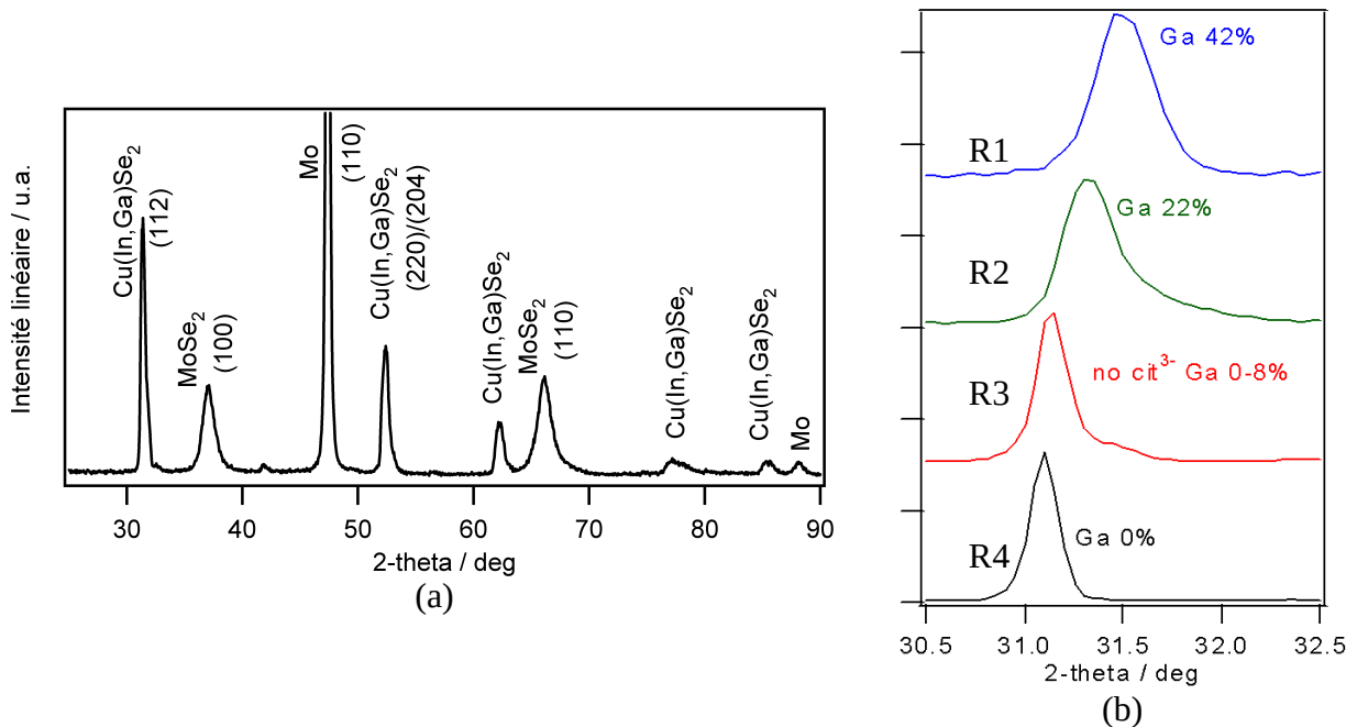
Figure 4.2.4. (a) Diffractogramme d'un échantillon sélénisé (R1), correspondant à une chalcopyrite de composition moyenne \text{CuIn}_{0.58}\text{Ga}_{0.42}\text{Se}_2 . (b) Elargissement d'échelle autour du pic (112) de la chalcopyrite. Les valeurs indiquées sont les rapports \text{Ga}/(\text{Ga}+\text{In}) en % calculés en utilisant une extrapolation linéaire des paramètres de maille indiqués par les fiches JCPDS. Anode en cobalt : \lambda_{\text{K}\alpha 1} = 0,1789 \text{ nm} .
