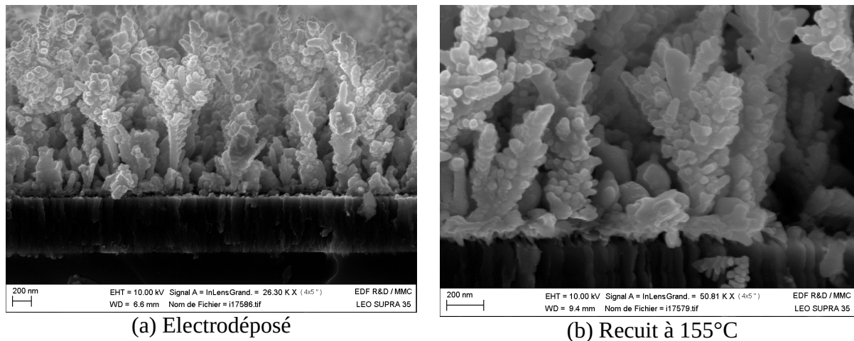
Figure 4.1.3. Micrographies en section d'un précurseur Cu-In-Ga dendritique sur substrat Mo (500 nm) sur verre (a) tel qu'électrodéposé ; (b) après un recuit de 30 min à 155°C.
