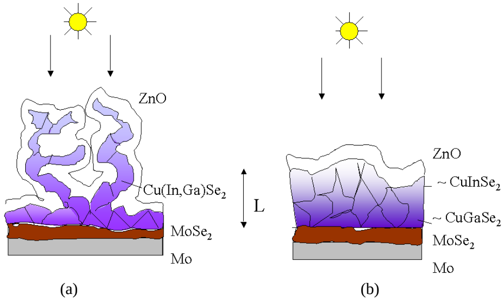
Figure 5.3. Schéma des cellules solaires obtenues dans le cas d'un précurseur Cu-In-Ga (a) sans recuit intermédiaire ou avec un recuit intermédiaire à 155^\circ\text{C} ; (b) avec un recuit intermédiaire réducteur à 550^\circ\text{C} . La couleur de l'absorbeur est modulée en fonction de la teneur en Ga (plus foncée pour une teneur en Ga plus élevée). L représente la longueur de diffusion des électrons. La fine couche de \text{CdS} (50 nm) entre l'absorbeur et le \text{ZnO} n'est pas représentée.
