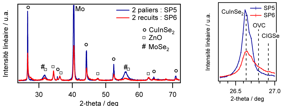
Figure 4.2.16. (a) Diffractogrammes des échantillons de Cu-In-Ga sélénisés en deux étapes et recouverts de CdS et ZnO. (b) élargissement autour du pic (112). En pointillés est représentée la position du pic pour différentes phases d'après les fiches JCPDS. OVC = \text{CuIn}_3\text{Se}_5 . CIGSe = \text{CuIn}_{0.7}\text{Ga}_{0.3}\text{Se}_2 . Anode en cuivre : \lambda_{\text{K}\alpha 1} = 0,15406 \text{ nm} .
