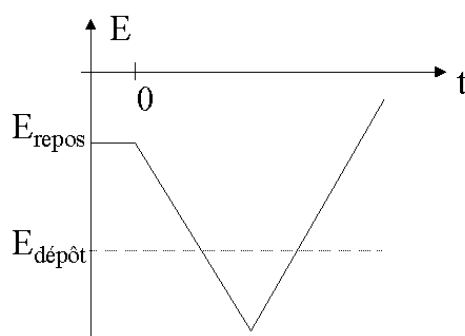
Figure 2.4. Evolution du potentiel au cours d'une voltammétrie cyclique
