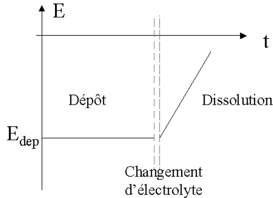
Figure 3.4.17. Potentiel appliqué pour la méthode d'analyse par dpôt/réoxydation avec changement d'électrolyte.
