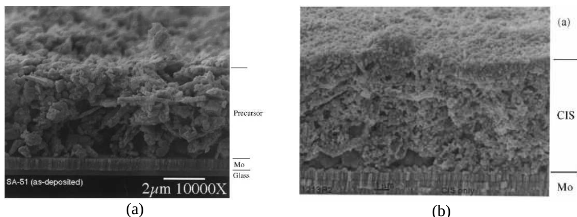
Figure 1.16. Coupe transverse vue au MEB (a) d'un précurseur composé de particules Cu-In déposé par spray ; (b) précurseur sélénisé qui forme un absorbeur \text{CuInSe}_2 comparable à celui ayant conduit à une cellule à 10,6% de rendement [49].
