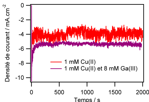
Figure B.1. Chronoampérogrammes à -1,4 V/MSE avec et sans espèces Ga(III) dans l'électrolyte. Electrolyte 0,4 M NaCl à pH 2,2 .
