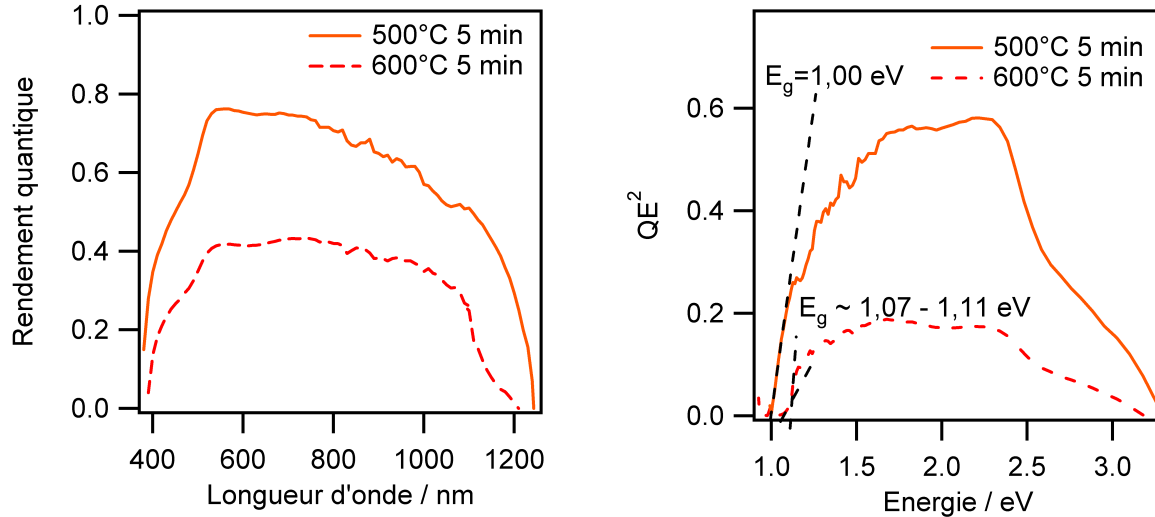
Figure 5.9. (a) Réponse spectrale (QE) des cellules solaires réalisées avec des précurseurs Cu-In-Ga sélénisés à 500^\circ\text{C} et 600^\circ\text{C} ; (b) Détermination de la largeur de bande interdite par le tracé QE^2 = f(E) . Cas d'une sélénisation avec une montée en température en 5 min, palier de 5 min.
