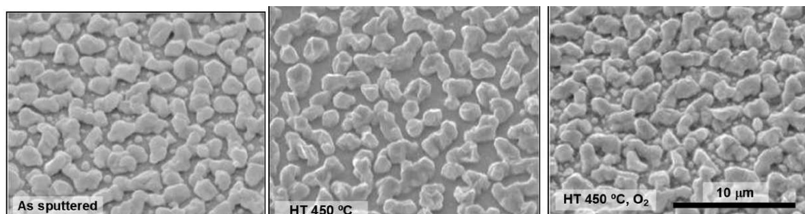
Figure 1.20. Micrographies MEB de précurseurs \text{Cu}_{0,81}\text{Ga}_{0,19} / \text{In} . HT indique un traitement thermique de 10 min dans 1 atm Ar; \text{O}_2 indique 0,0035% \text{O}_2 dans le flux d'Ar [128].
