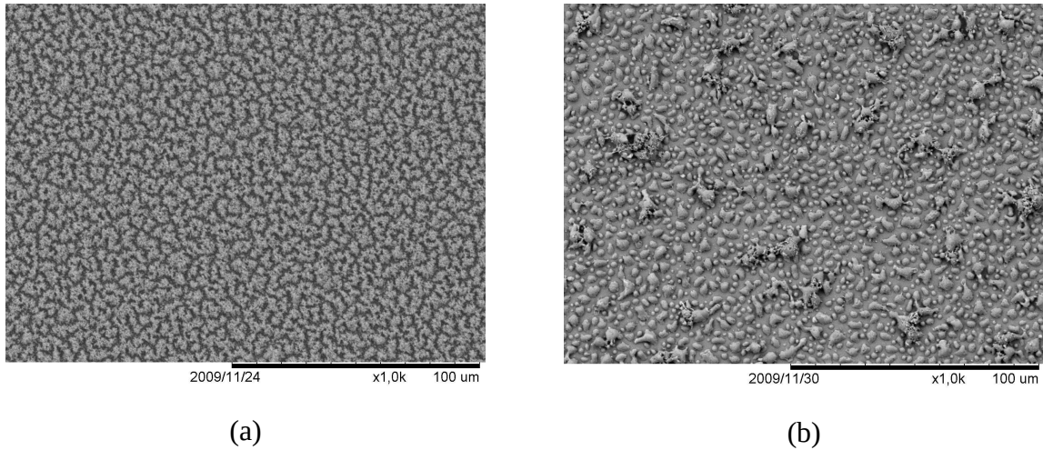
Figure 4.1.9. Micrographie de précurseurs Cu-In-Ga sur substrat Mo SGI (a) avant et (b) après recuit réducteur
