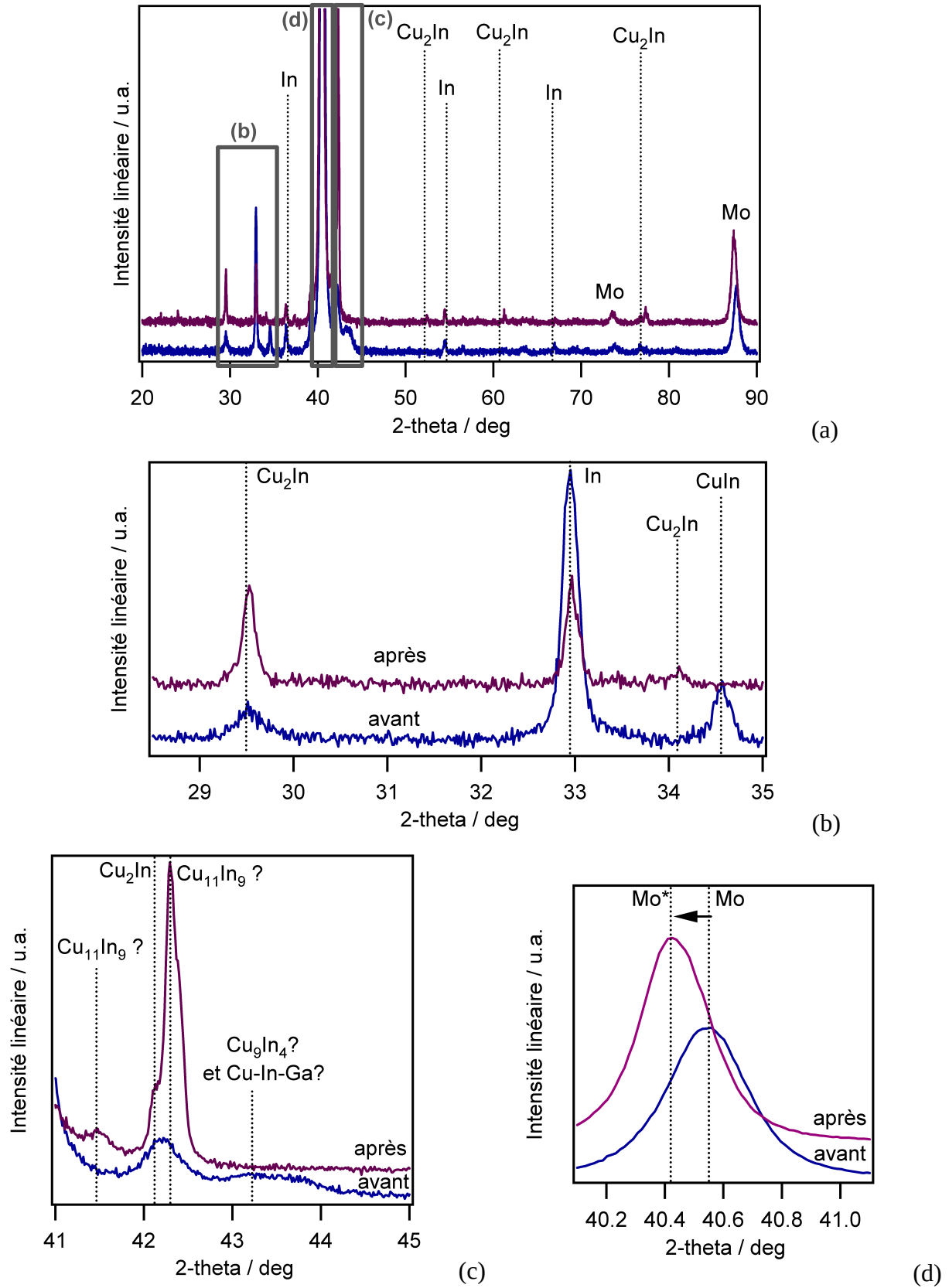
Figure 4.1.6. Diffractogrammes du précurseur avant et après recuit intermédiaire (anode en \text{Cu} : \lambda_{\text{K}\alpha 1} = 1,5406 \text{ \AA} ) : (a) global ; (b) agrandissement d'échelle pour 2\theta = 28\text{-}35^\circ ; (c) agrandissement d'échelle pour 2\theta = 41\text{-}45^\circ ; (d) agrandissement d'échelle pour 2\theta = 39\text{-}41^\circ . L'astérisque * indique que les paramètres de maille ont été modifiés (cf. tableau 4.1.2).
