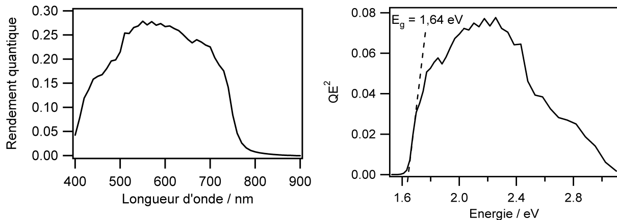
Figure 5.7. (a) Réponse spectrale (QE) d'une cellule solaire à base de CuGaSe 2 ; (b) Détermination de la largeur de bande interdite par le tracé QE^2 = f(E) .
