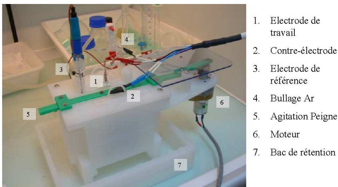
Figure 2.3. Photographie du réacteur utilisé.
