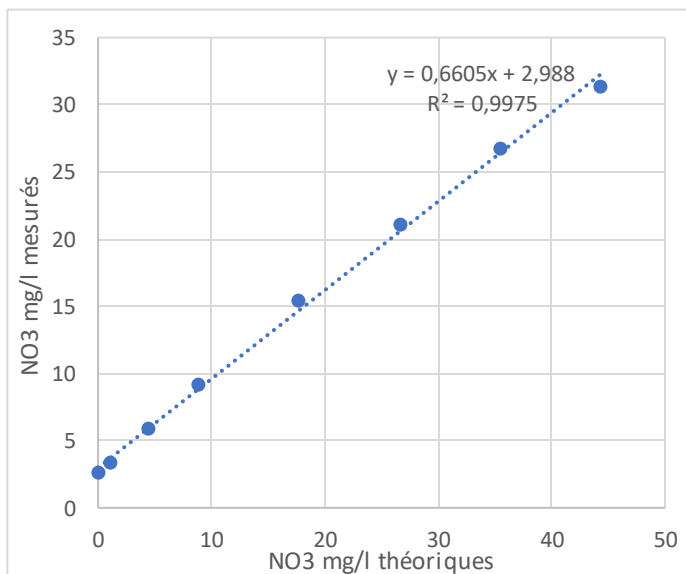
Figure 4 : Courbe d'étalonnage de la sonde s::can
