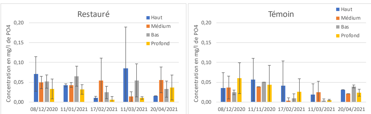
Figure 16 : Concentrations en orthophosphates, par campagne, sur le site de La Haie et son témoin
