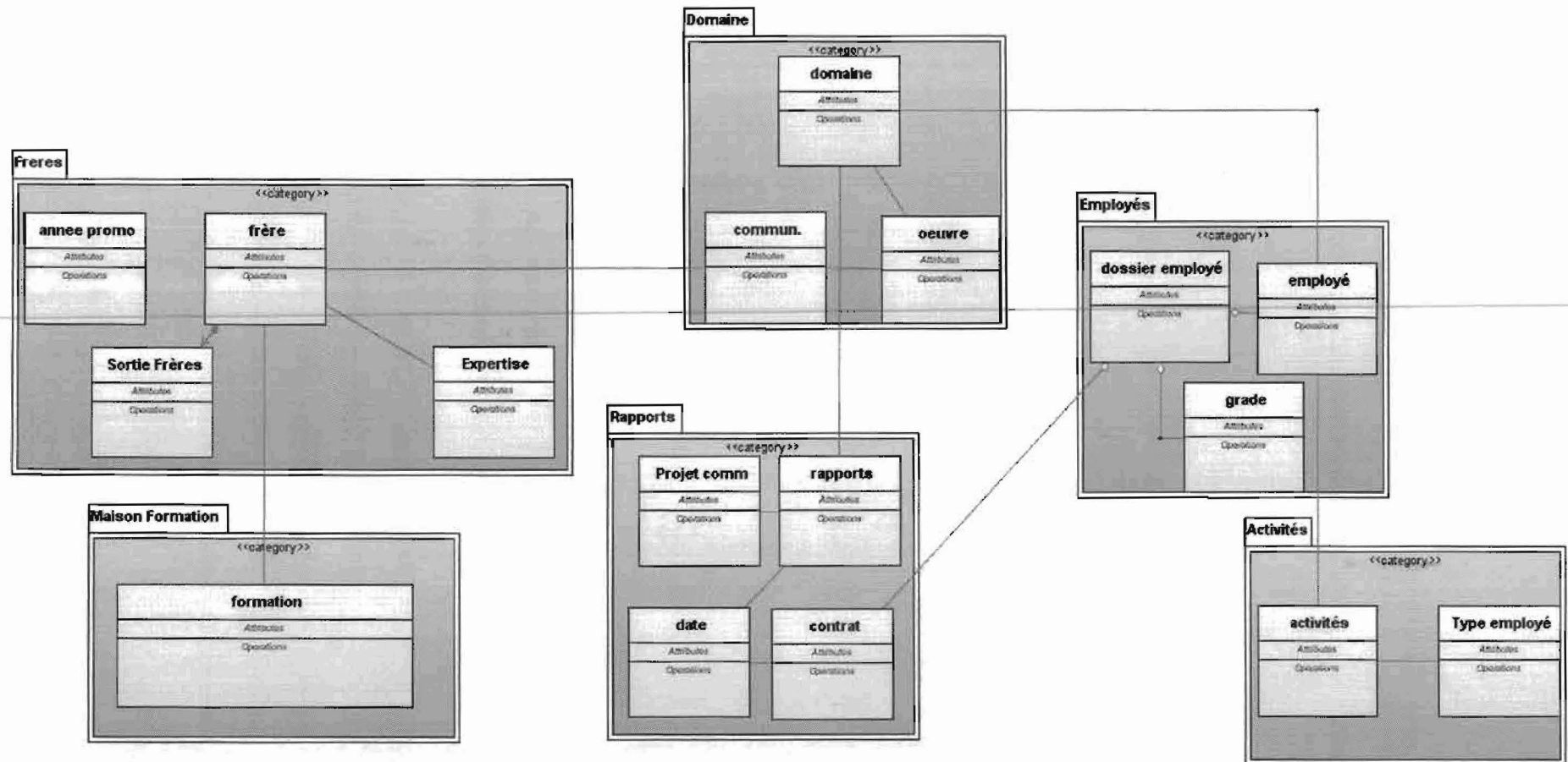
Figure 10: diagramme de paquetages
