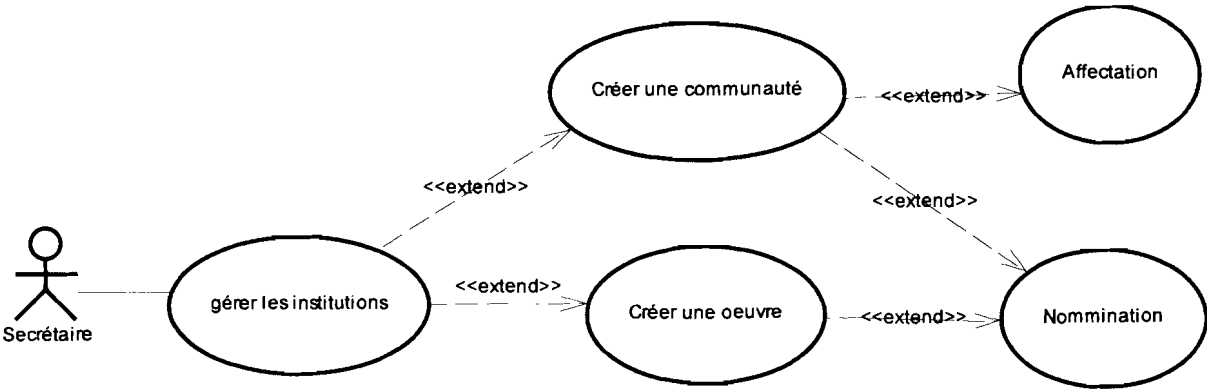
Figure 28: Raffinement de cas d’utilisation : GERER LES INSTITUTIONS
