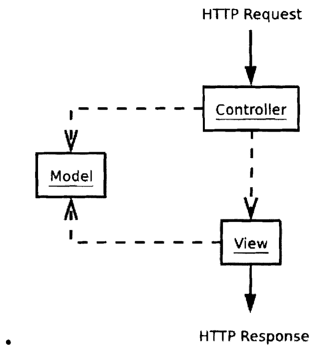
Figure 18: Modèle MVC Global
