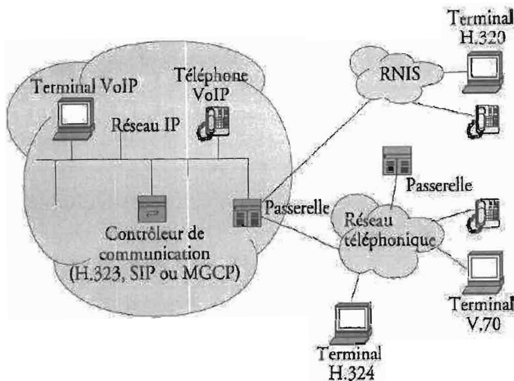
Figure II.1 : architecture de la VoIP en entreprise [1]
