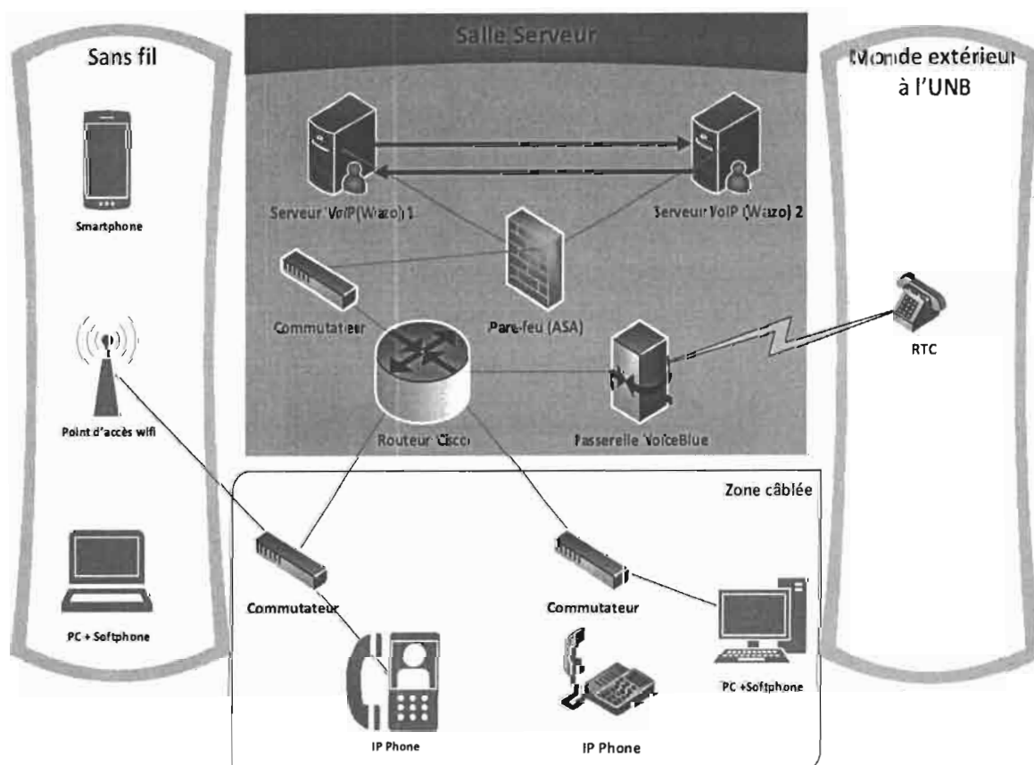
Figure IV.4 : architecture de mise en œuvre de la solution
