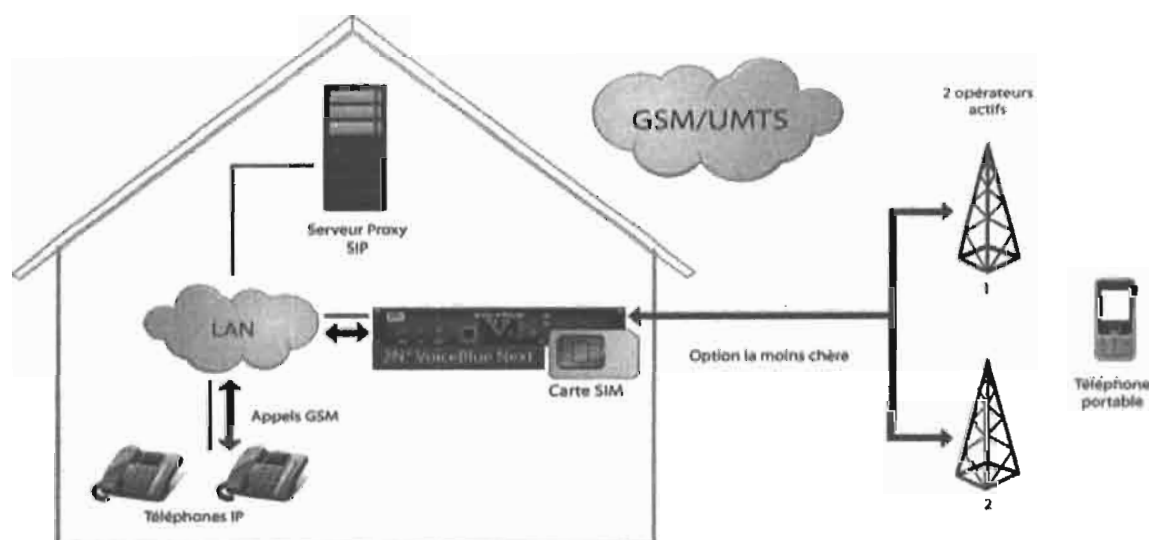
Figure IV.3 : architecture de déploiement de 2N® VoiceBlue
