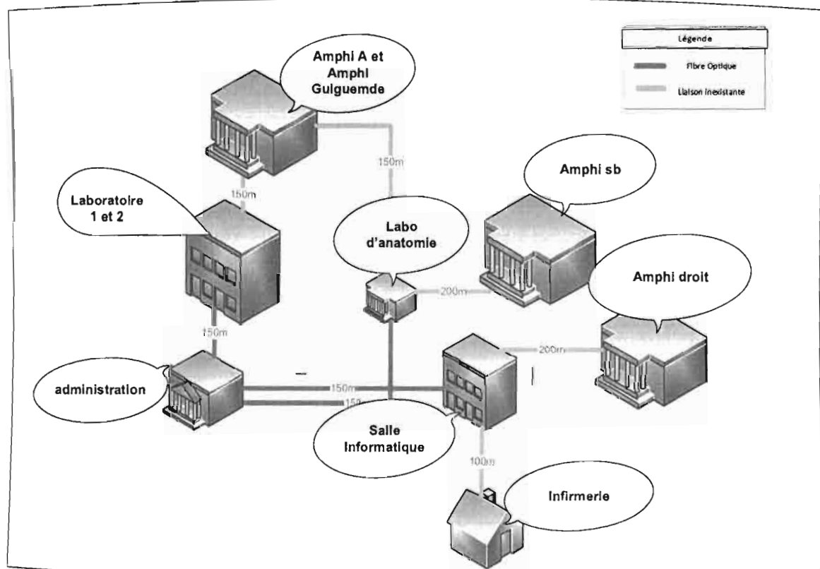
Figure III.2 Architecture réseau de l'INSSA
