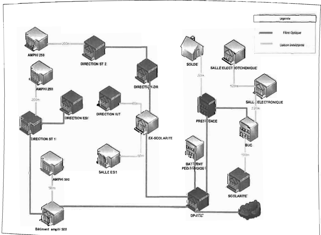
Figure III.1 Architecture réseau de Nasso
