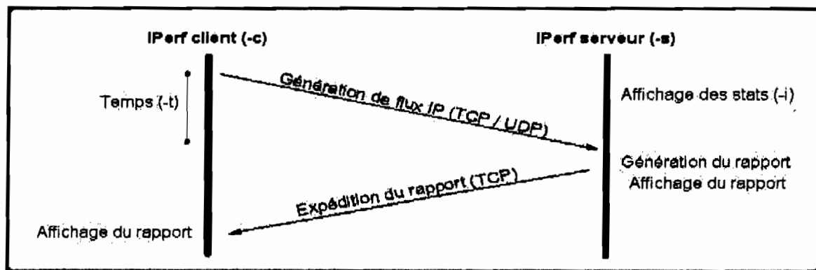
Figure V.4 : principe de fonctionnement d'IPerf
