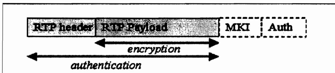
Figure VI.1 : le format d'un paquet SRTP
