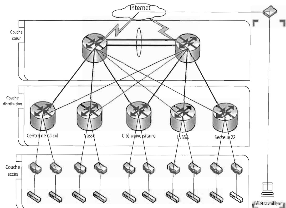
Figure IV.2 : proposition d'architecture logique de la couche cœur du réseau de l'U.N.B.
