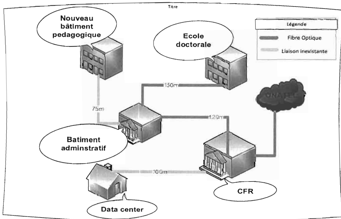
Figure III.3 Architecture réseau du centre de calcul
