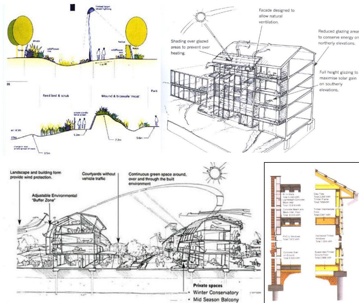
Aspects constructifs et approche bioclimatique – Millennium Village. Source: Don Barker (2001).
