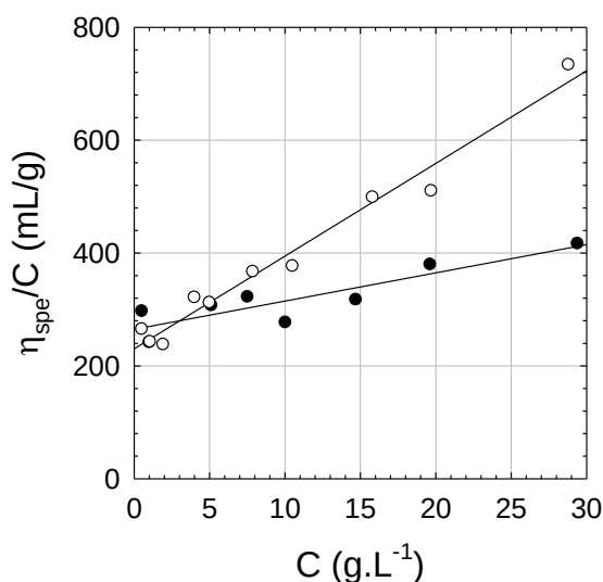
Figure 3 : Variation de la viscosité spécifique réduite (\eta - \eta_0)/(\eta_0 C) à T=20 °C en fonction de la concentration en PAM- g -PNIPAM-A10-b. \eta et \eta_0 sont respectivement la viscosité de la solution de polymère et celle du solvant. (○) pH = 3 ; (●) pH = 11.
