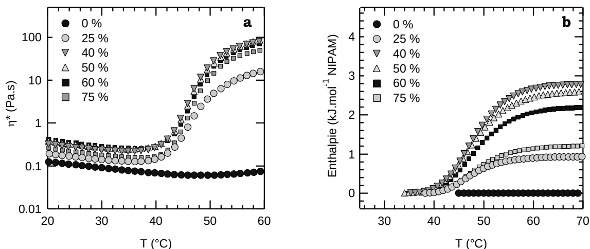
Figure 35 : Evolution de la viscosité (a) et de l'enthalpie (b) en fonction de la température pour des mélanges de copolymères PAM- g -PNIPAM-A10- c ( C_p = 80 \text{ g.mol}^{-1} ) et PNIPAM-M10- c à pH 7.
