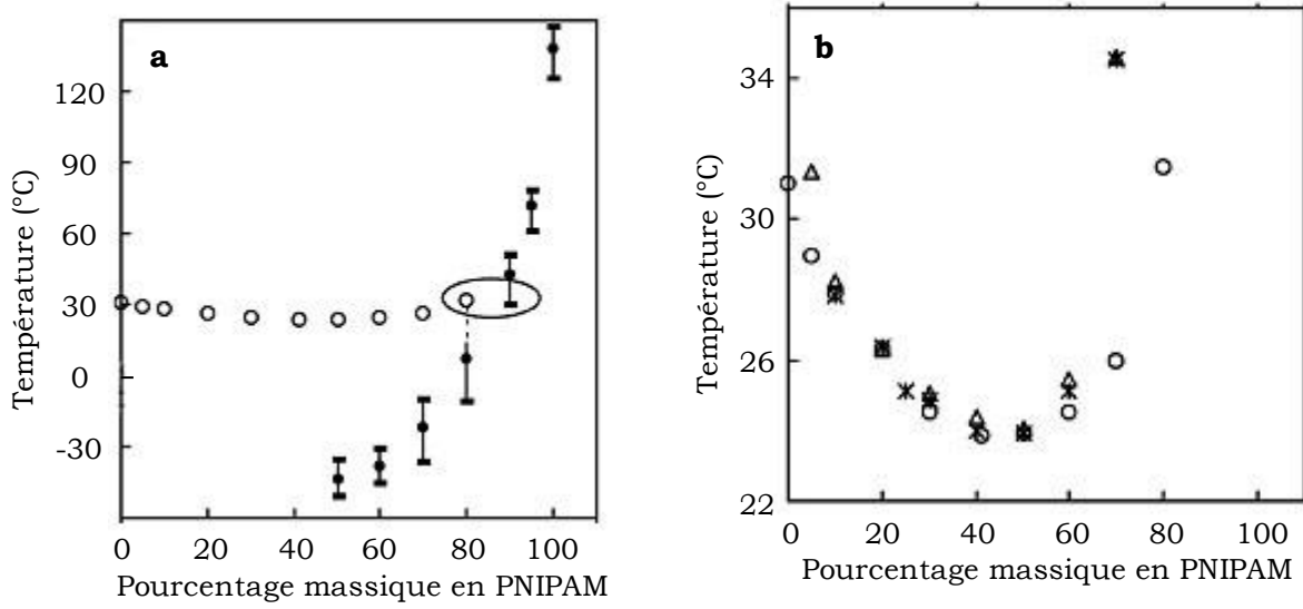
Figure 6 : Diagrammes de phase du mélange binaire PNIPAM/eau. a : Courbes de démixtion (O) et transition vitreuse de solution de PNIPAM (M = 74 kg/mol) - b : Courbes de démixtion de solutions aqueuses de PNIPAM de masses différentes : M = 18 kg/mol (Δ); M = 74 kg/mol (O) et M = 187 kg/mol). D'après Van Durme et al 34 .
