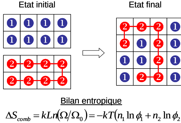
Figure 7 : Représentation schématique du calcul de \Delta S_{comb} pour un mélange solvant/polymère avec k la constante de Boltzmann, \Omega et \Omega_0 le nombre de configurations différentes respectivement dans l'état final et initial, n_1 et n_2 le nombre de molécules (1) et de macromolécules (2), \phi_1 et \phi_2 leurs fractions volumiques respectives.
