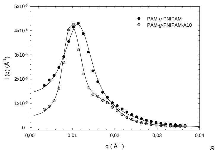
Figure 18 : Spectres de diffusion des solutions de PAM- g -PNIPAM-b et PAM- g -PNIPAM-A10-c à 60 ^{\circ}\text{C} ( C_p = 80 \text{ g.L}^{-1} ). A chaque courbe expérimentale correspond une courbe calculée (en trait plein).
