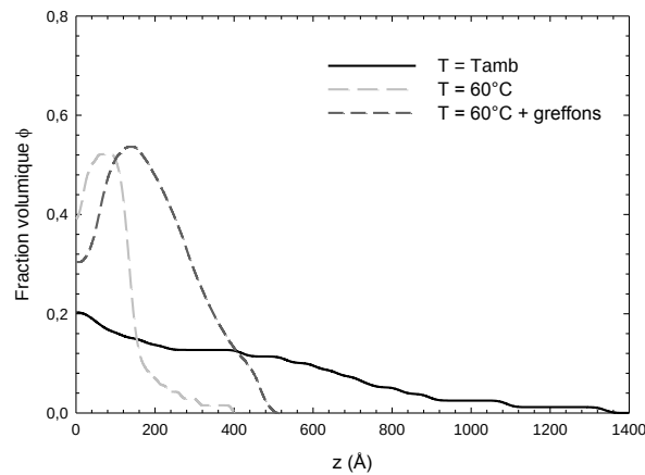
Figure 25 : Profils de fraction volumique d'une brosse de PNIPAM ( M_n = 121\,000\text{ g.mol}^{-1} et \sigma = 7,76.10^{-4}\text{ Å}^{-2} ) à température ambiante, à 60^\circ\text{C} et en présence de greffons PNIPAM-A10-b ( C_p = 0,1\% ) à 60^\circ\text{C} .
