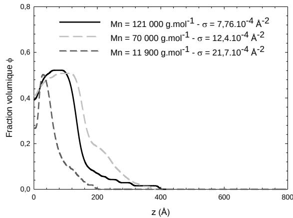
Figure 20 : Profils de fraction volumique de brosses de PNIPAM de longueurs de chaînes différentes ( M_n = 121\,000 , 70\,000 et 11\,900\text{ g.mol}^{-1} ) dans l'eau lourde à pH 7 et à 60°C.
