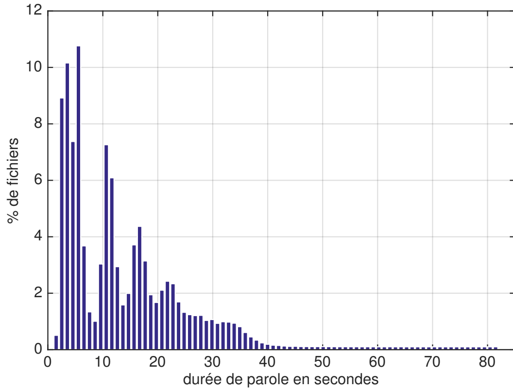
FIGURE 1.12 – Distribution des segments audio dans le jeu de test officiel de LRE15 en fonction de la durée de parole.
