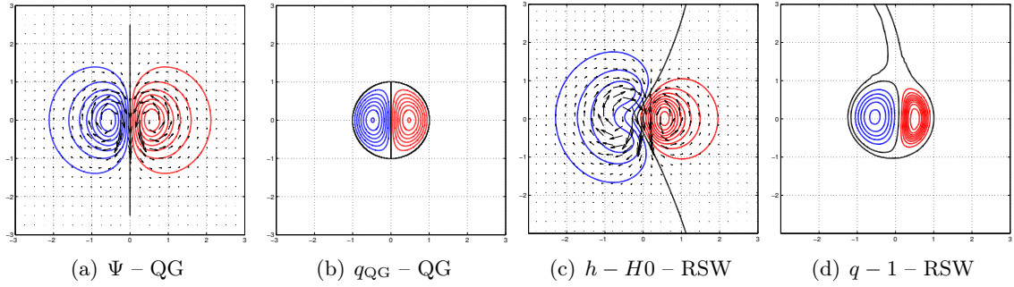
FIGURE 3.1 – Comparaison du champ d'anomalie de pression ( \Psi en QG, h - H_0 en RSW, grandeurs adimensionnées) avec le champ de vitesse superposé, et d'anomalie de vorticit  potentielle entre la solution dipolaire QG et la solution ag ostrophique dans le mod le RSW obtenue par simulations num riques. Isolignes donn es   intervalle \pm 0.04 pour la pression/hauteur (adimensionn es respectivement par gH_0 et H_0 ) et \pm 0.5 pour l'anomalie de PV (adimensionn e par f/H_0 ). Rouge : cyclone, bleu : anticyclone, noir : anomalie nulle. Param tres du modon : Ro = 0.2 , Bu = \Lambda^{-2} = 1 .
