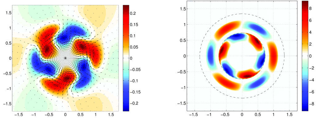
FIGURE 2.23 – Représentation de la structure du mode le plus instable pour le cyclone de catégorie 3. A gauche : champ de pression (couleurs) et de vitesse (vecteurs). A droite : champ de vortacité relative. Les cercles tiretés représentent les niveaux critiques. Les amplitudes sont normalisées par le maximum d'amplitude des champs du mode considéré. (Ici, \max(|V|) \simeq 0.8 .)
