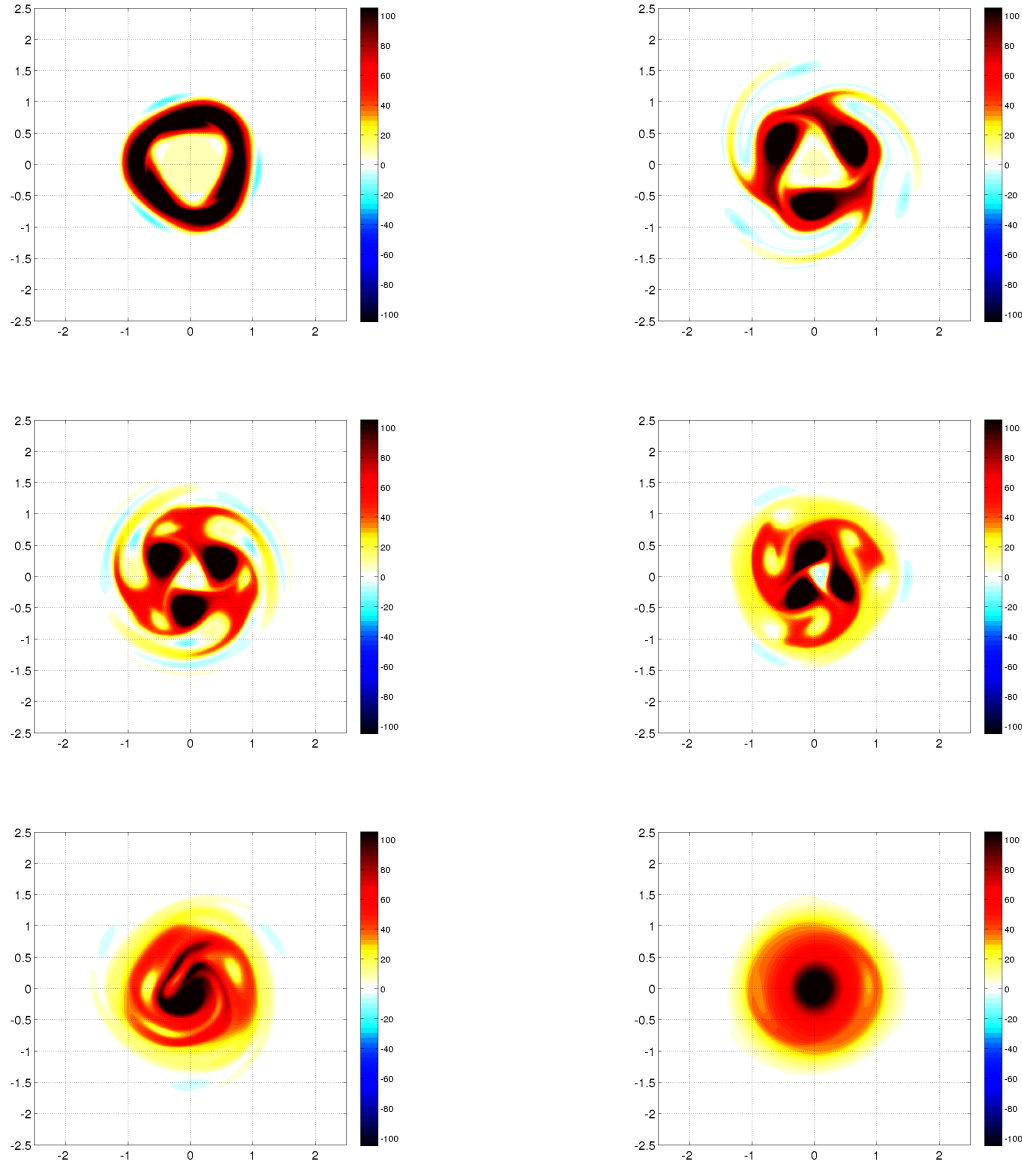
FIGURE 2.26 – Evolution de l’anomalie de vorticité potentielle au cours de la saturation non linéaire de l’instabilité du cyclone tropical de catégorie. Mode le plus instable : l = 3 . De gauche à droite et de haut en bas : t = 0, 0.5, 1, 1.5, 2 et 4 f^{-1} . Une petite portion seulement du domaine numérique est montrée. Les coordonnées spatiales sont adimensionnée par la taille typique du vortex, et la vorticité potentielle est adimensionnée par f/H_0 .
