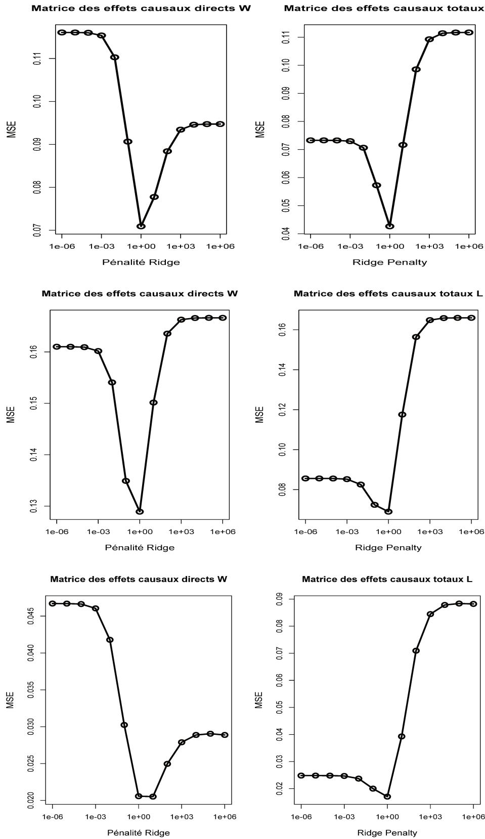
FIGURE 4.6 – Quelques résultats pour différentes simulations. Les résultats en haut et au centre sont issus d'un graphe à 10 noeuds, le dernier d'un graphe à 100 noeuds.
