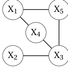
Grphe non-orienté associé à \Sigma^{-1}
