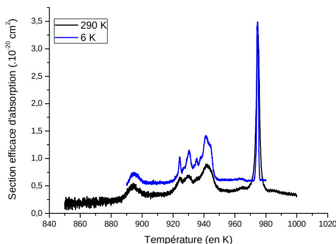
Figure B - 4 : Sections efficaces d'absorption d'une céramique Yb : Sc 2 O 3 dopée 10 at. % à 290 K (courbe noire) et à 6 K (courbe bleue).
