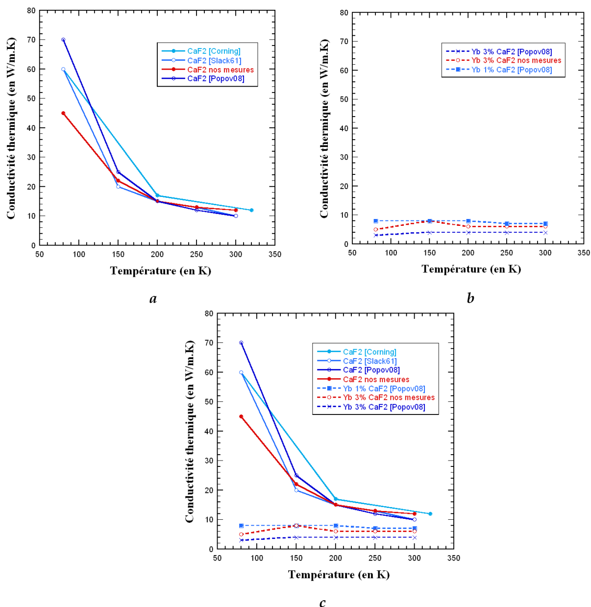
Figure IV - 31 : Conductivités thermiques obtenues pour des cristaux CaF2 non dopé (a) et dopé ytterbium (b) à basse température. Ensemble des résultats regroupés (c).
