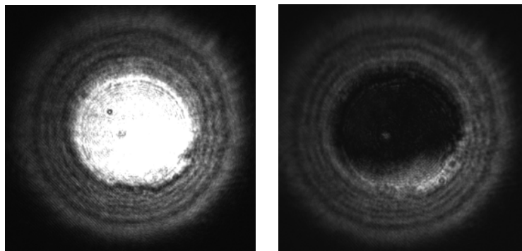
Figure III - 24 : Photo de la figure d'interférence obtenue en configuration de la teinte plate dans le cas d'un échantillon cylindrique.
