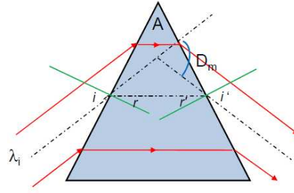
Figure III - 4 : Schéma de propagation dans un prisme.
