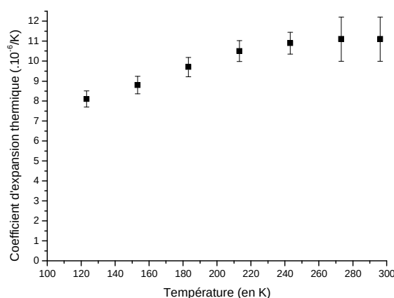
Figure III - 19 : Coefficients d'élongation thermique du verre phosphate dopé 4 at. % néodyme, LHG-8, Hoya, à basse température.
