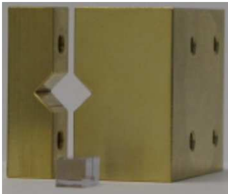
Figure III - 22 : Photo du support échantillon en laiton avec un échantillon de verre phosphate dopé néodyme.
