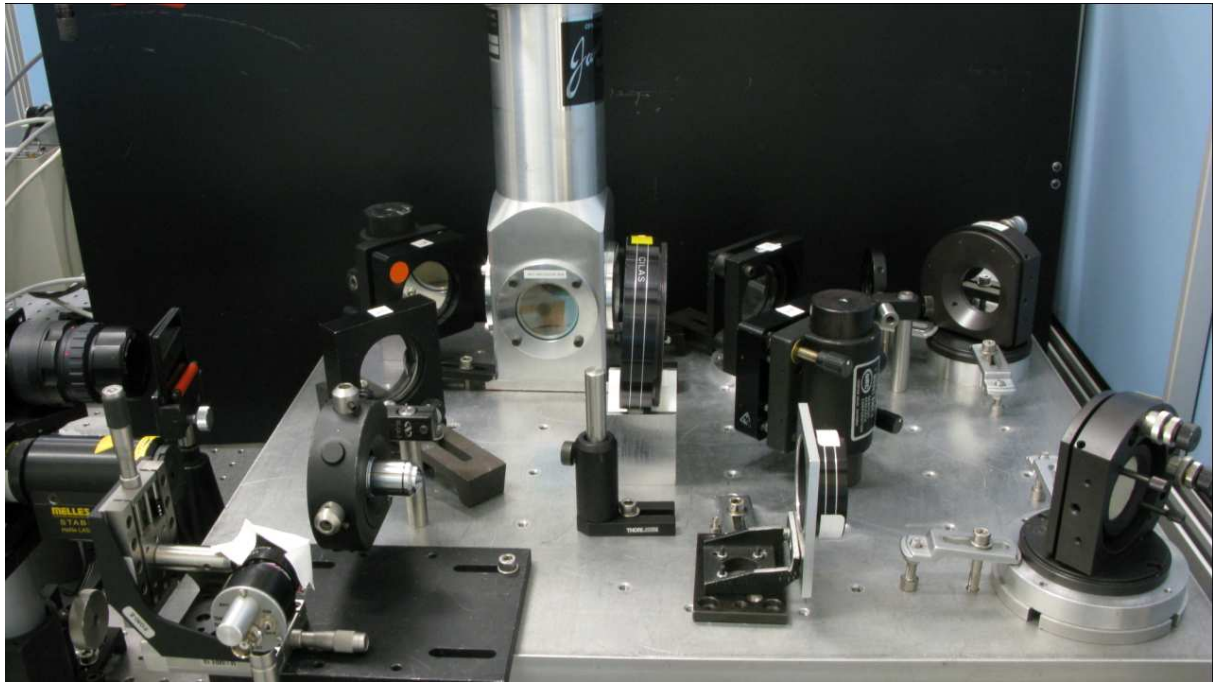
Figure III - 21 : Photo de l'interféromètre type Mach-Zehnder.
