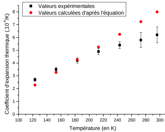
Figure III - 17 : Coefficients d'élargissement thermique d'un cristal de YAG non dopé à basse température. Comparaison avec les valeurs d'élargissement thermique calculées par la régression de Fan et al. [Fan 98].
