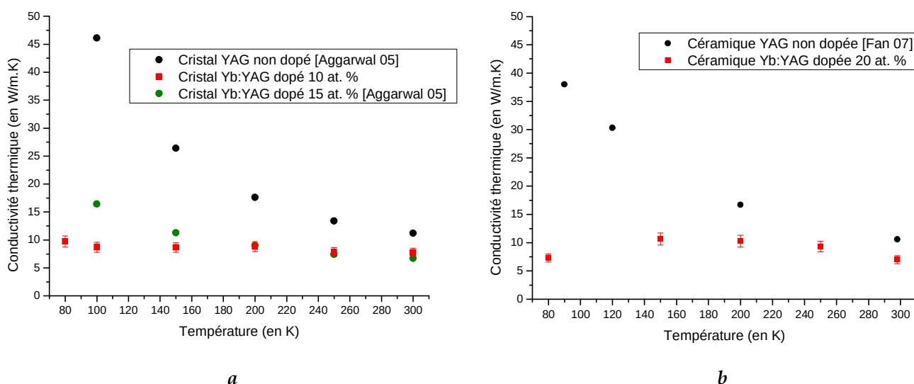
Figure IV - 28 : a : Conductivités thermiques obtenues pour un cristal Yb : YAG dopé 10 at. % à basse température. b : Conductivités thermiques obtenues pour une céramique Yb : YAG dopée 20 at. % à basse température. Comparaison avec les conductivités thermiques mesurées sur des cristaux / céramiques YAG [Aggarwal 05], [Fan 07].
