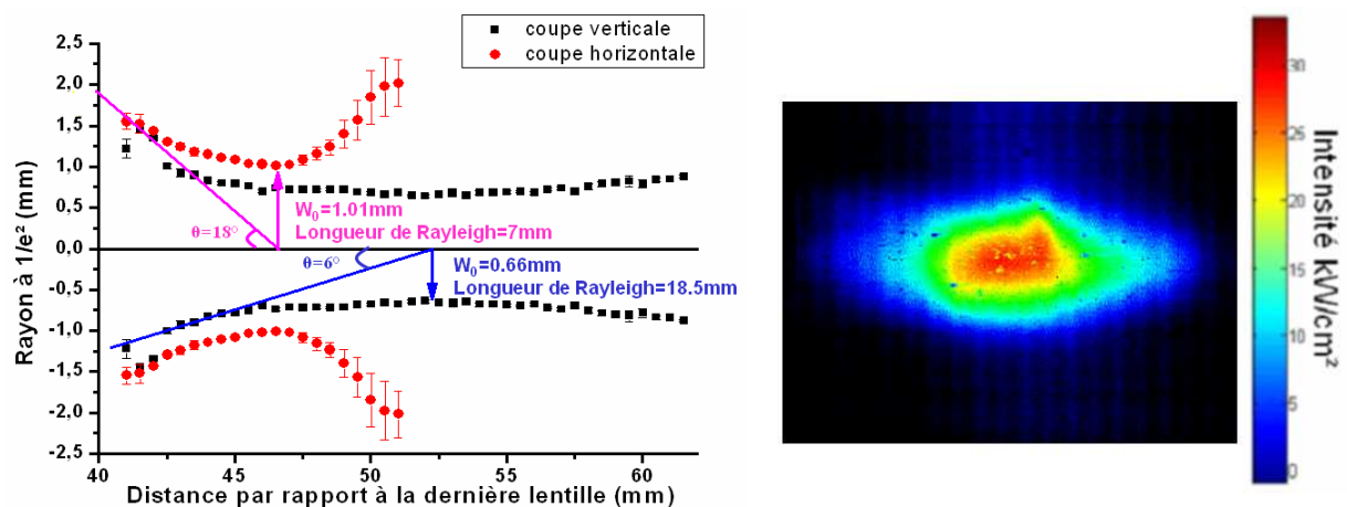
Figure II - 7 : Caustique du faisceau de pompe et représentation en 2 dimensions de la tache focale au meilleur foyer pour une cadence de 10 Hz, une durée d'impulsion de 1 ms, un courant d'alimentation de 30 A et une température du système de refroidissement de 20^\circ\text{C} .
