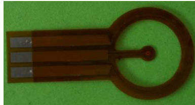
Figure IV - 18 : Photo de la sonde annulaire.
