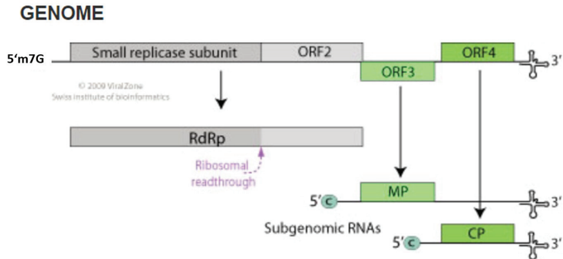
Figure 11: Génome du tobacco mosaic virus (TMV) représentatif des tobamovirus
