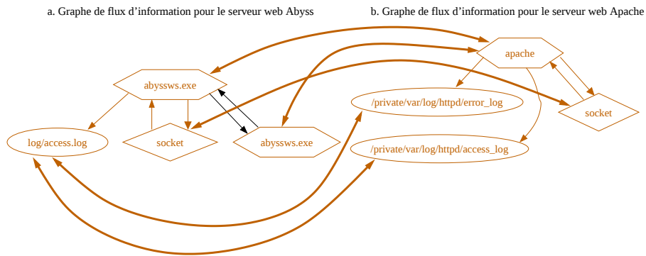
FIG. 4.9 – Meilleur mapping entre les graphes des serveurs Apache et Abyss
