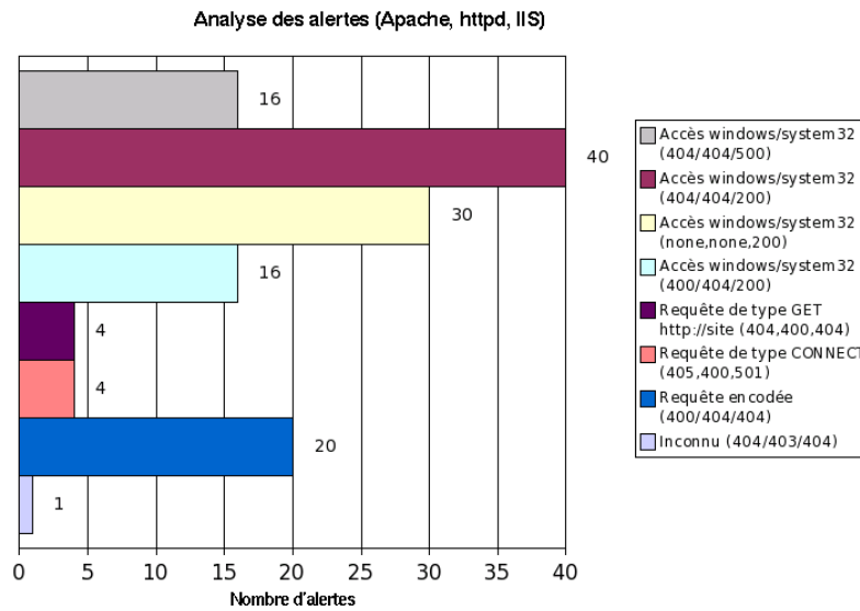
FIG. 4.2 – Analyse des alertes
