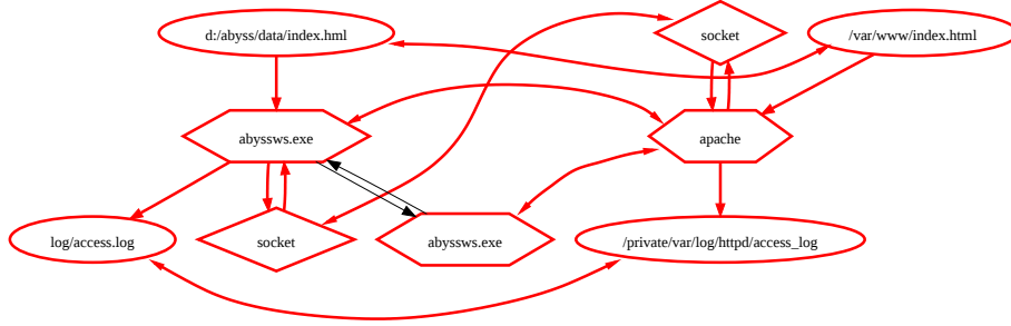
FIG. 2.9 – Exemple d'un meilleur mapping entre deux graphes de flux d'informations
