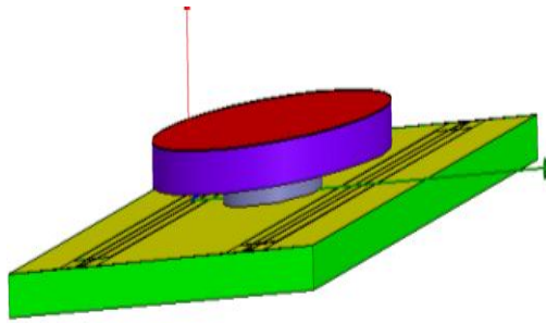
I-7 : Capteur de gaz RF passif à modes de galerie
