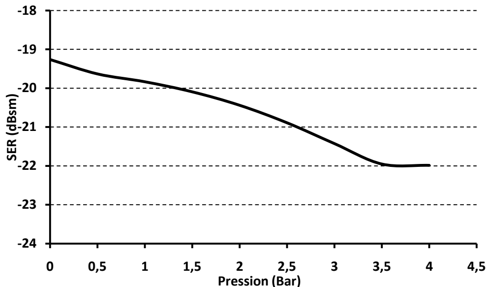
III-30 : SER de la cible (antenne + câble + capteur)
