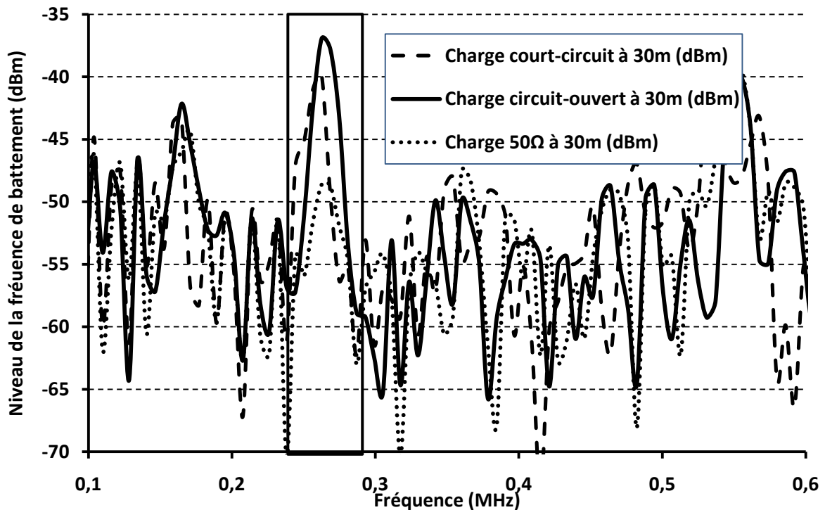
III-14 : Antenne cornet connectée à différentes charges (CC, CO, 50Ω)
