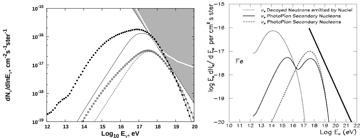
FIG. 6.2 : Gauche : Spectres des neutrinos dans le cas ( \alpha = 2, m = 3 ) pour les courbes du haut, et dans le cas ( \alpha = 2.5, m = 4 ) pour les courbes du bas. Les lignes fines sont calculées uniquement avec le CMB, tandis que les carrés prennent en compte aussi les interactions avec le fond infrarouge (dont l'évolution avec z est la même que dans CRPropa ). La zone grisée correspond à la limite de Waxman-Bahcall. D'après [137]. Droite : Spectres prédits par saveur, dans le cas d'une injection de fer aux sources avec E_{\text{max}} = 4Z \times 10^{20} eV et ( \alpha = 2, m = 3 ). On voit en particulier la contribution due à la désintégration des neutrons. D'après [140].
