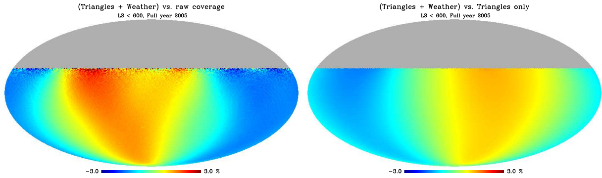
FIG. 2.27 : Gauche : différence relative entre la couverture calculée avec un modèle complet d'acceptance (voir texte) et la couverture correspondante invariance en ascension droite, pour le lot de données « de référence ». Droite : différence relative entre les couvertures prenant et ne prenant pas en compte les effets météorologiques sur l'acceptance.
