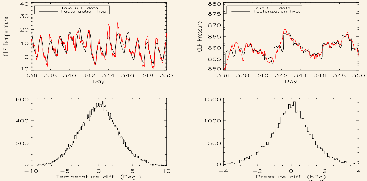
Figure : Haut : exemples de comparaisons entre l'évolution temporelle des paramètres (\tilde{T}, \tilde{P}) « factorisés », en noir, avec les vraies données (T, P) , en rouge. Bas : histogrammes des différences entre (\tilde{T}, \tilde{P}) et (T, P) pour la période 2004 - 2005.
