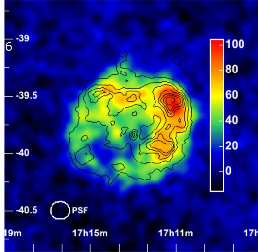
FIG. 4.4 : Le reste de supernova RXJ1713.7-3946 vue en VHE \gamma par HESS, avec les contours en rayons X (ASCA). Carte mise à jour à l'ICRC 2005.
