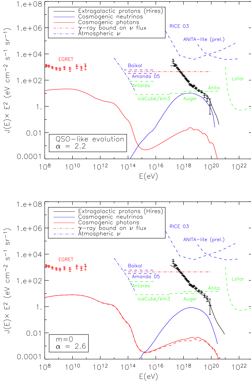
FIG. 6.1 : Spectres des fonds diffus d’UHECRs et des neutrinos et photons secondaires pr dits dans des mod les de propagation rectiligne de protons. La normalisation est fix e par les mesures de HiRes. Haut : la densit  des sources  volue avec z . Bas : densit  comobile de sources uniforme. Les flux de neutrinos repr sentent un flux par saveur, en supposant explicitement un m lange total de ces saveurs sur des distances cosmologiques. On repr sente par ailleurs les flux mesur s de photons (EGRET) et le flux moyen de neutrinos atmosph riques, ainsi que les valeurs limites sup rieures sur le flux de neutrinos qui sont  tablies (en bleu), et les sensibilit s des exp riences futures ou en cours (en vert).
