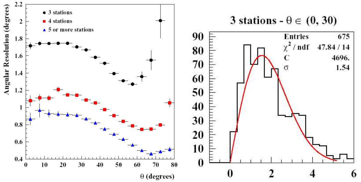
FIG. 1.15 : Gauche : Résolution angulaire estimée (SD seul), en fonction du nombre de cuves de l'événement et de son angle d'incidence. Droite : comparaison entre les directions d'arrivée reconstruites FD et SD pour les hybrides avec 3 cuves touchées. On utilise cette comparaison pour calculer des résolutions angulaires plus conservatrices que celles obtenues avec la reconstruction du SD seul.
