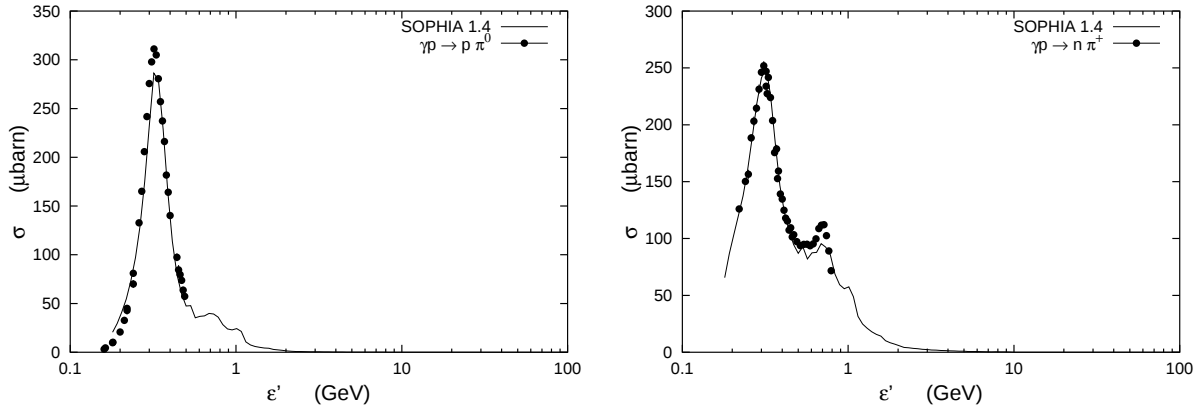
FIG. 4.6 : Sections efficaces totales des réactions générant un pion unique \gamma p \rightarrow \pi^0 p et \gamma p \rightarrow \pi^+ p : comparaison des données d'accélérateur et des simulations SOPHIA [80].
