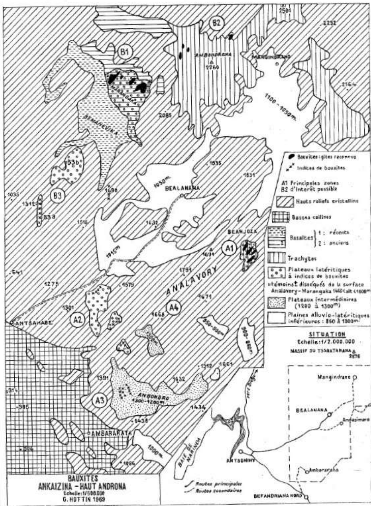
Figure 12 : Localisation des indices de bauxite à Analavory, Bealanana (Razafiniparany A. 1969).
